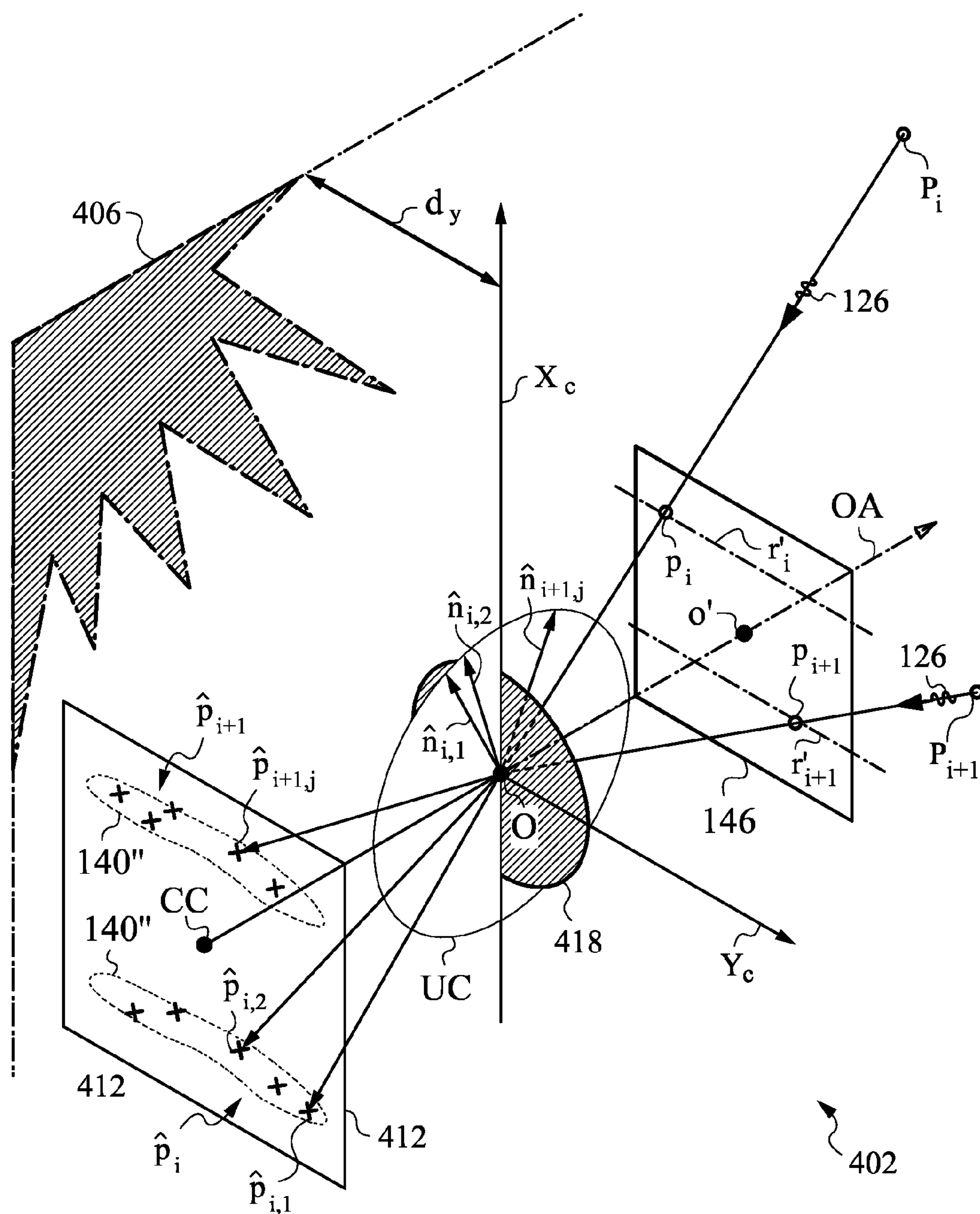
FIG. 15
