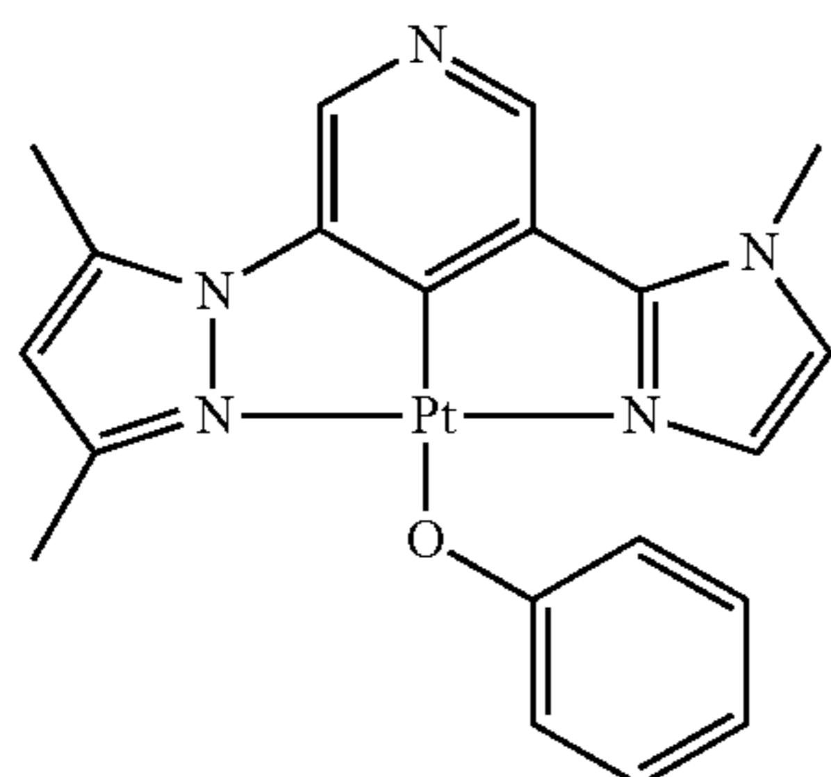
DMPz—Py—MIz—PtOPh
