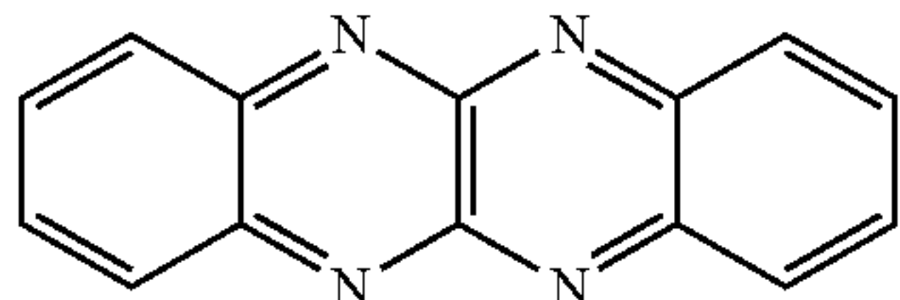
quinoxalino[2,3-b]quinoxaline
