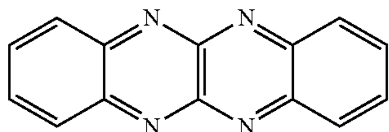
quinoxalino[2,3-b]quinoxaline
