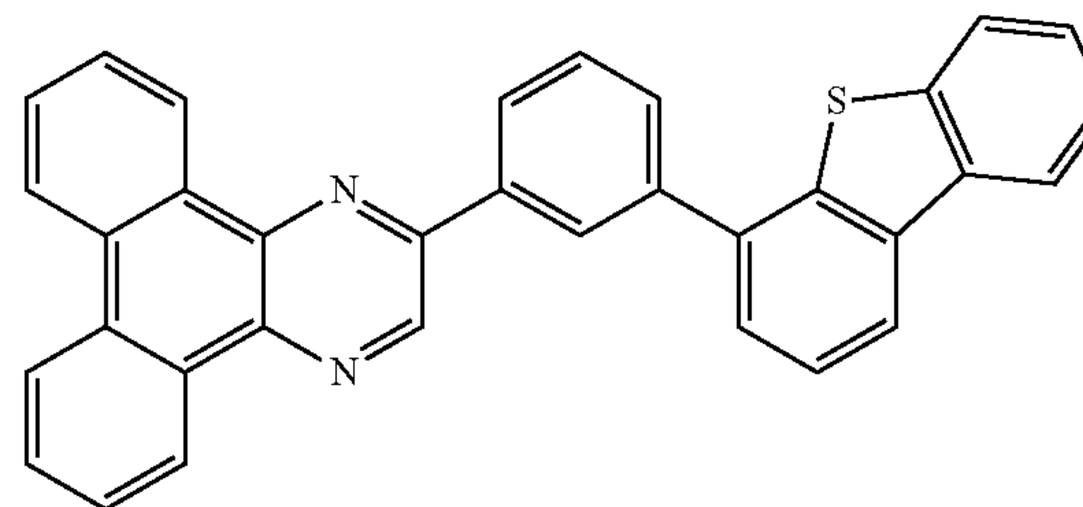
2mDBTPDBq-II
