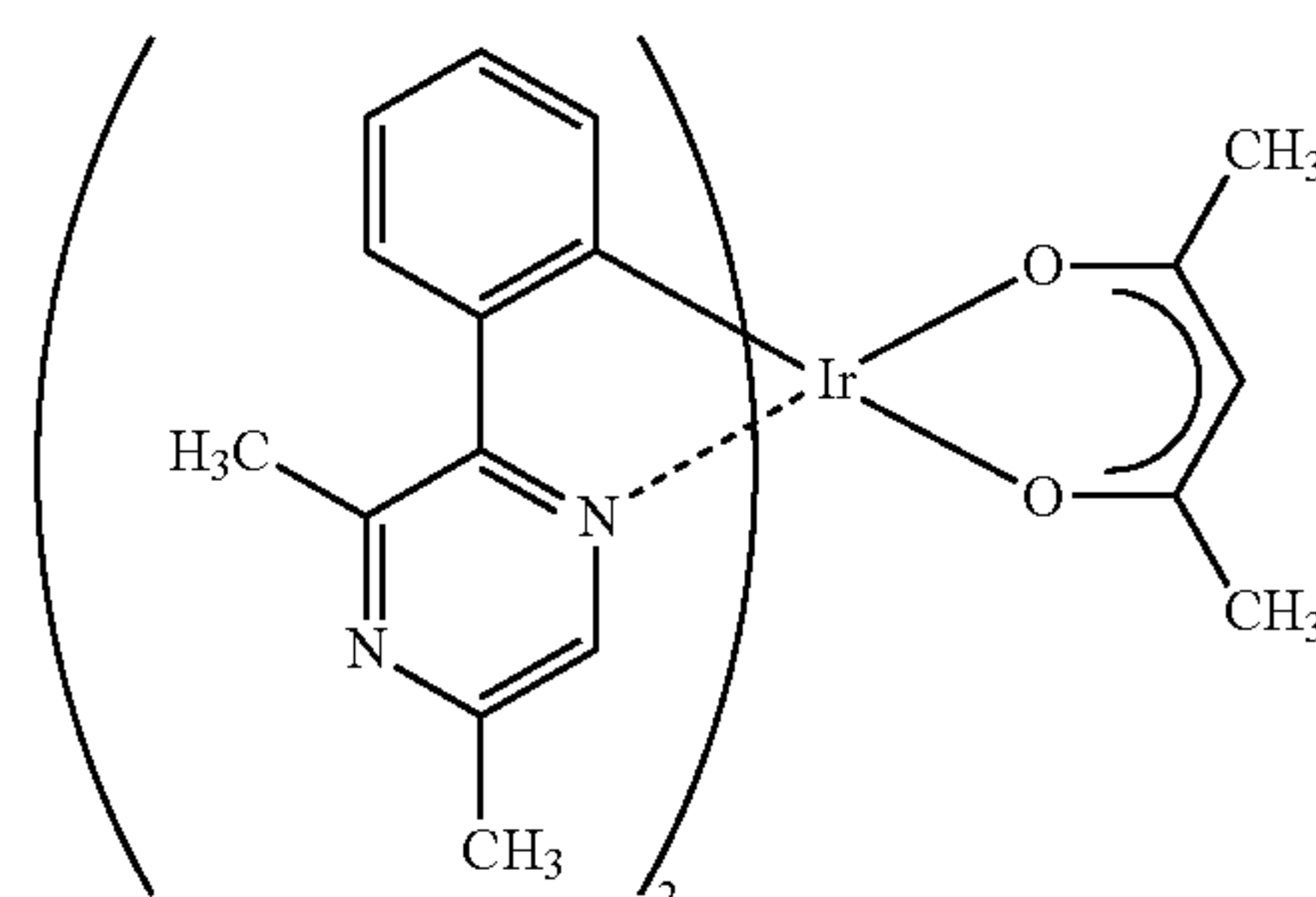
Ir(mppr-Me) 2 (acac)
