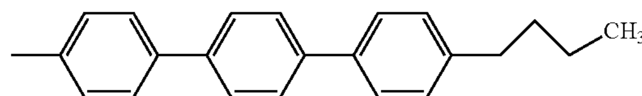
4-butyl-[1,1';4',1'']terphenyl-4-yl
