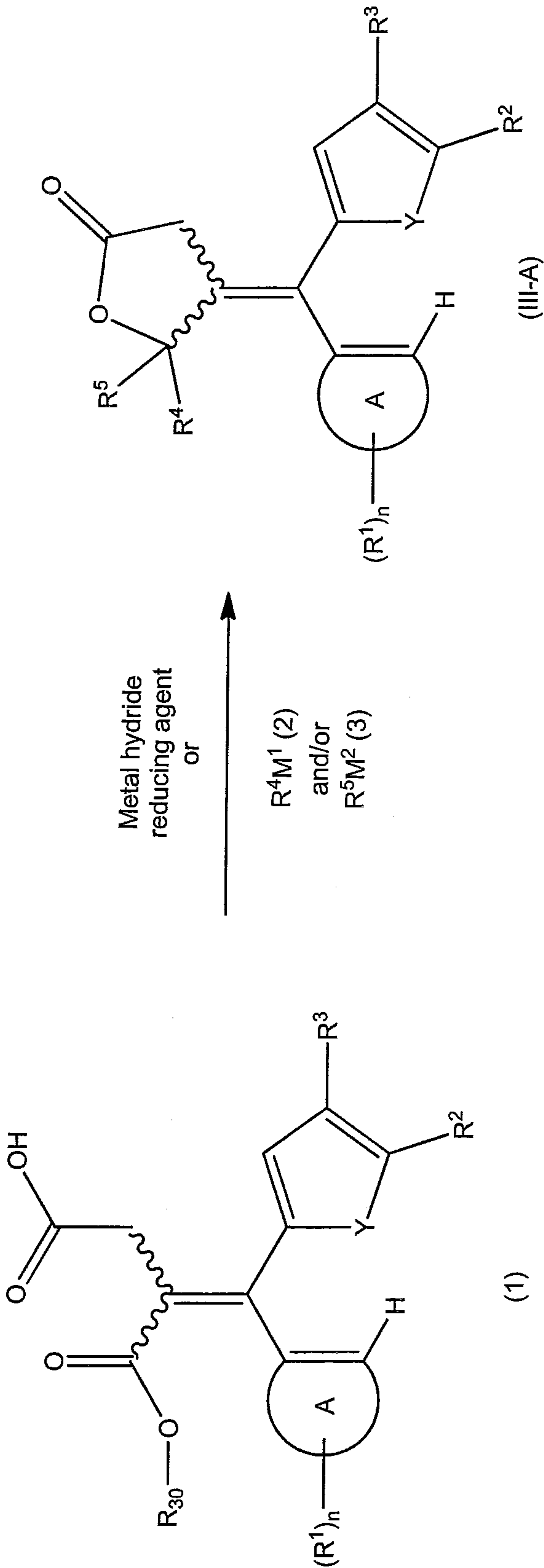
Scheme-(5)
