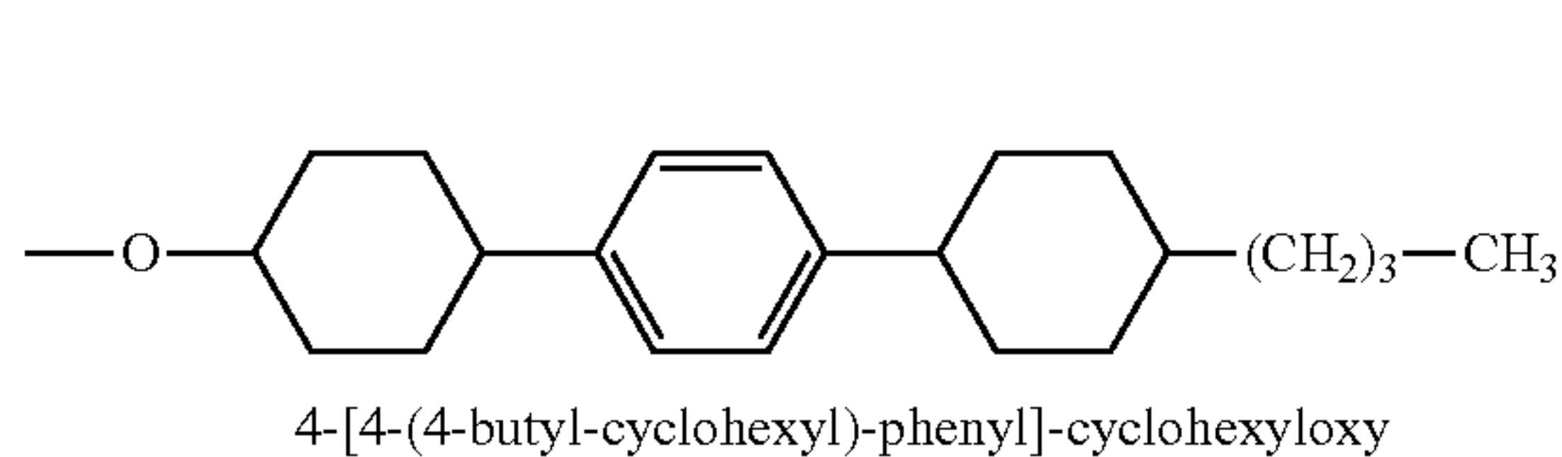
L(1)
