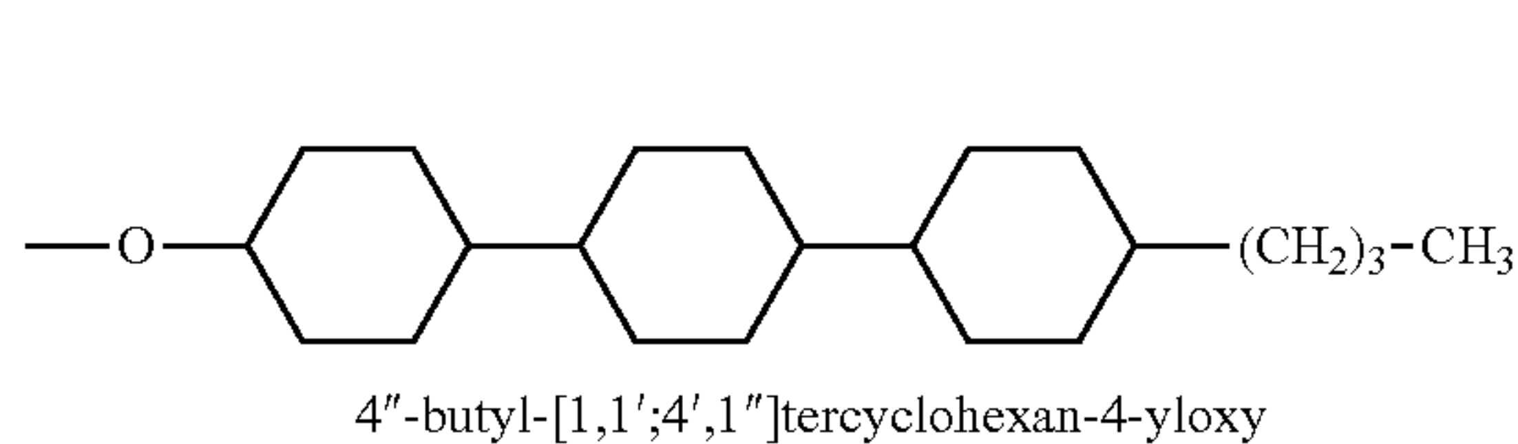
L(2)
