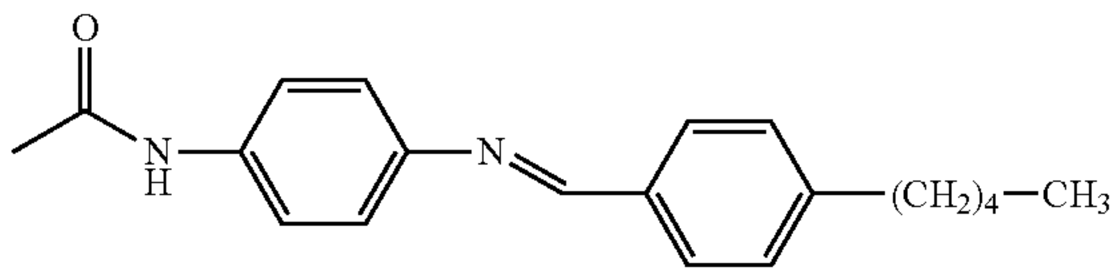
N-{4-[4-pentyl-benzylidene)-amino]phenyl}-acetamidyl
