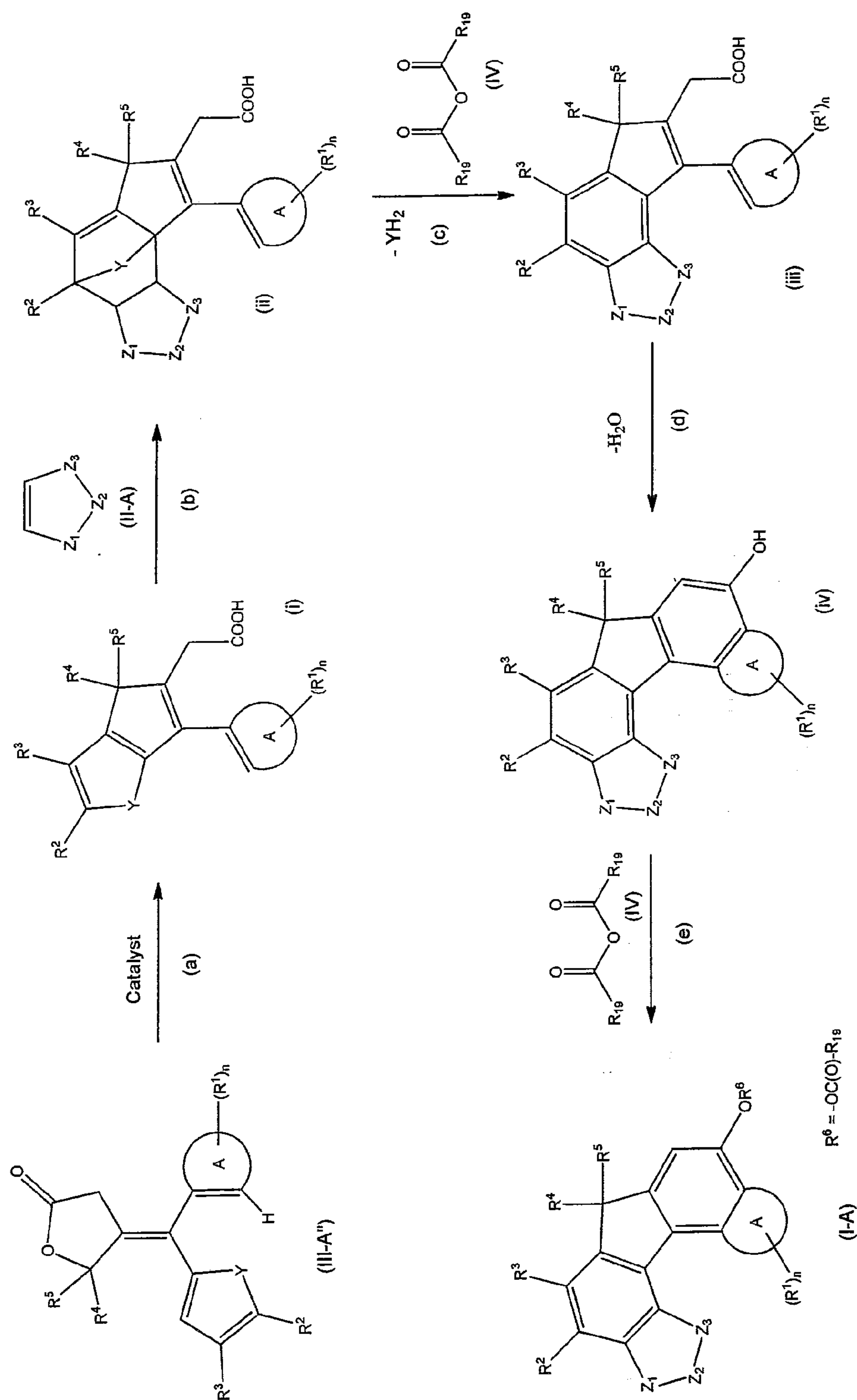
Scheme-(2)
