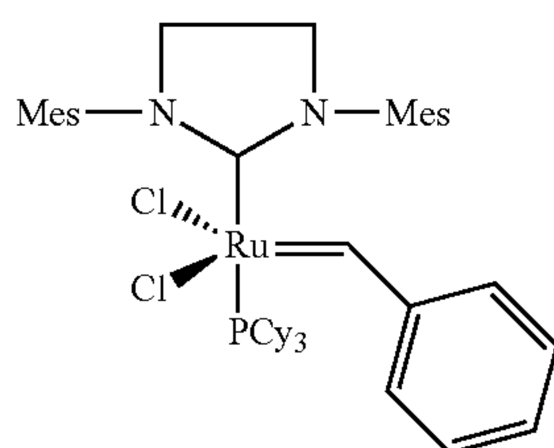
(Grubbs II)
