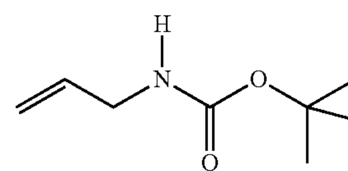
t-butyl-N-allylcarbamate
