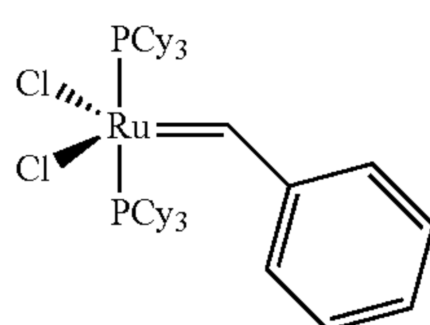
(Grubbs I)
