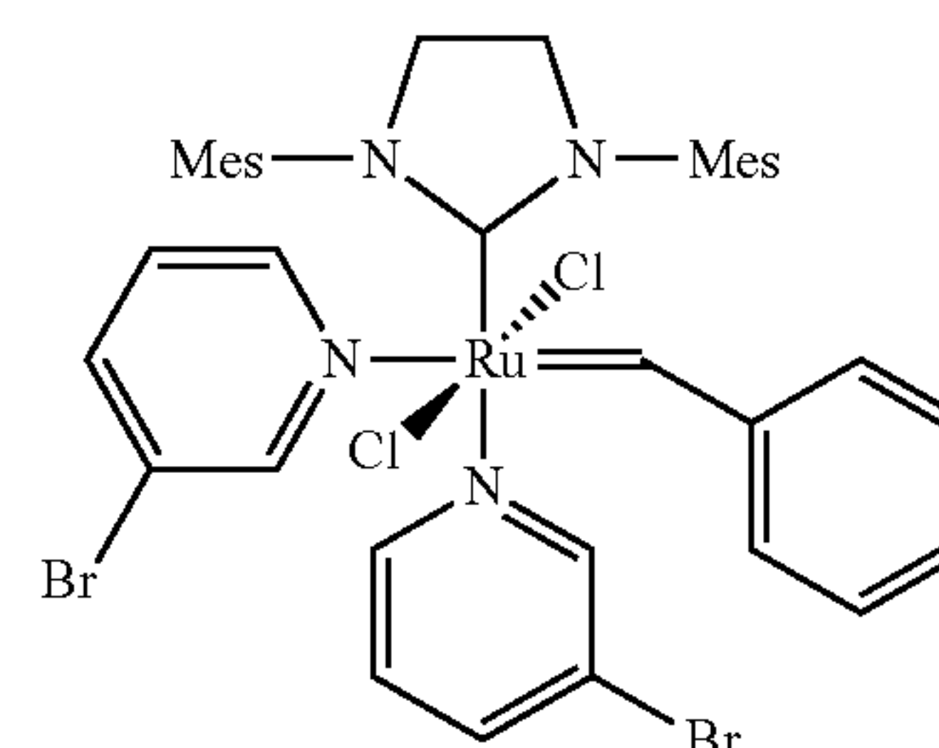
(Grubbs III)
