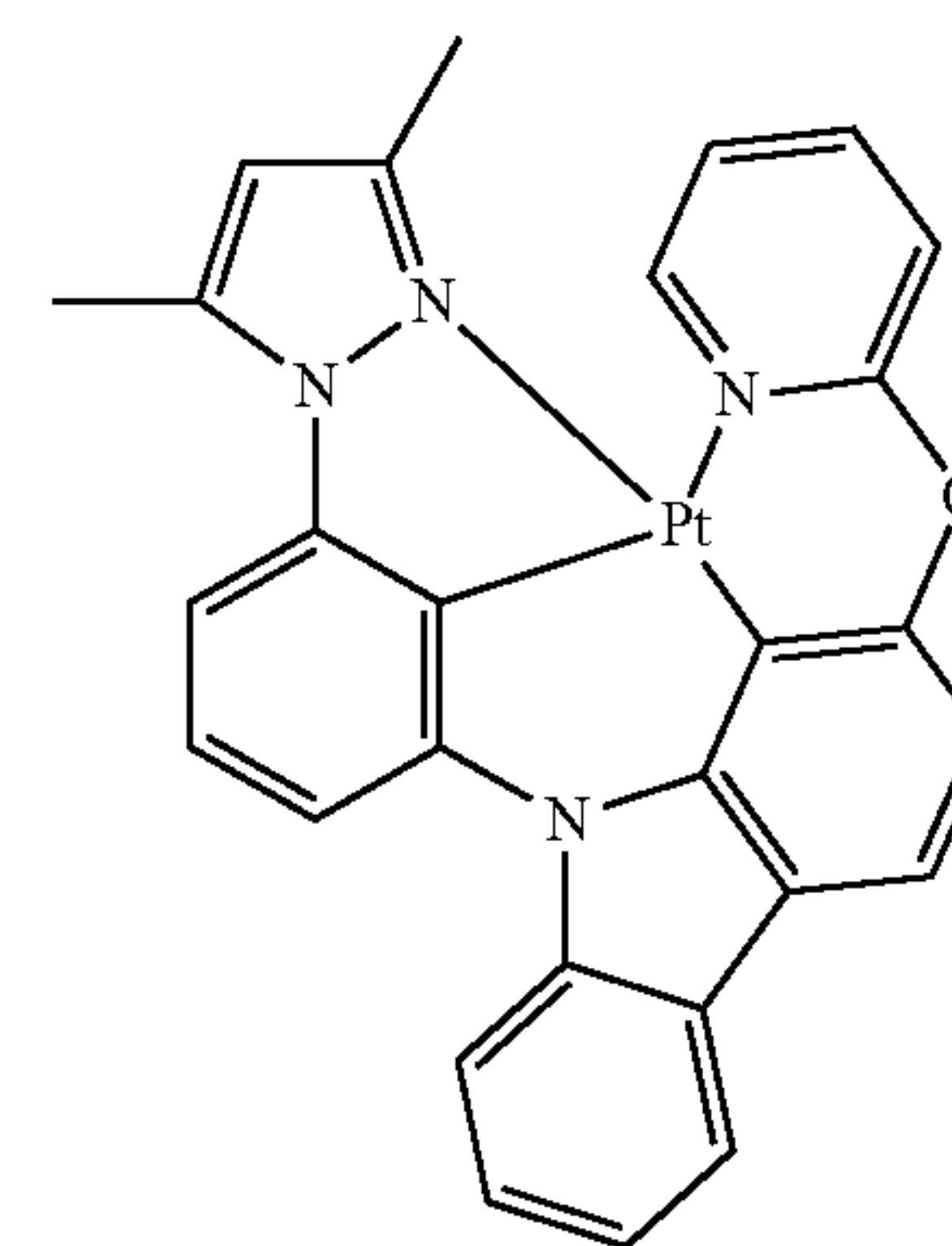
Pt-008
