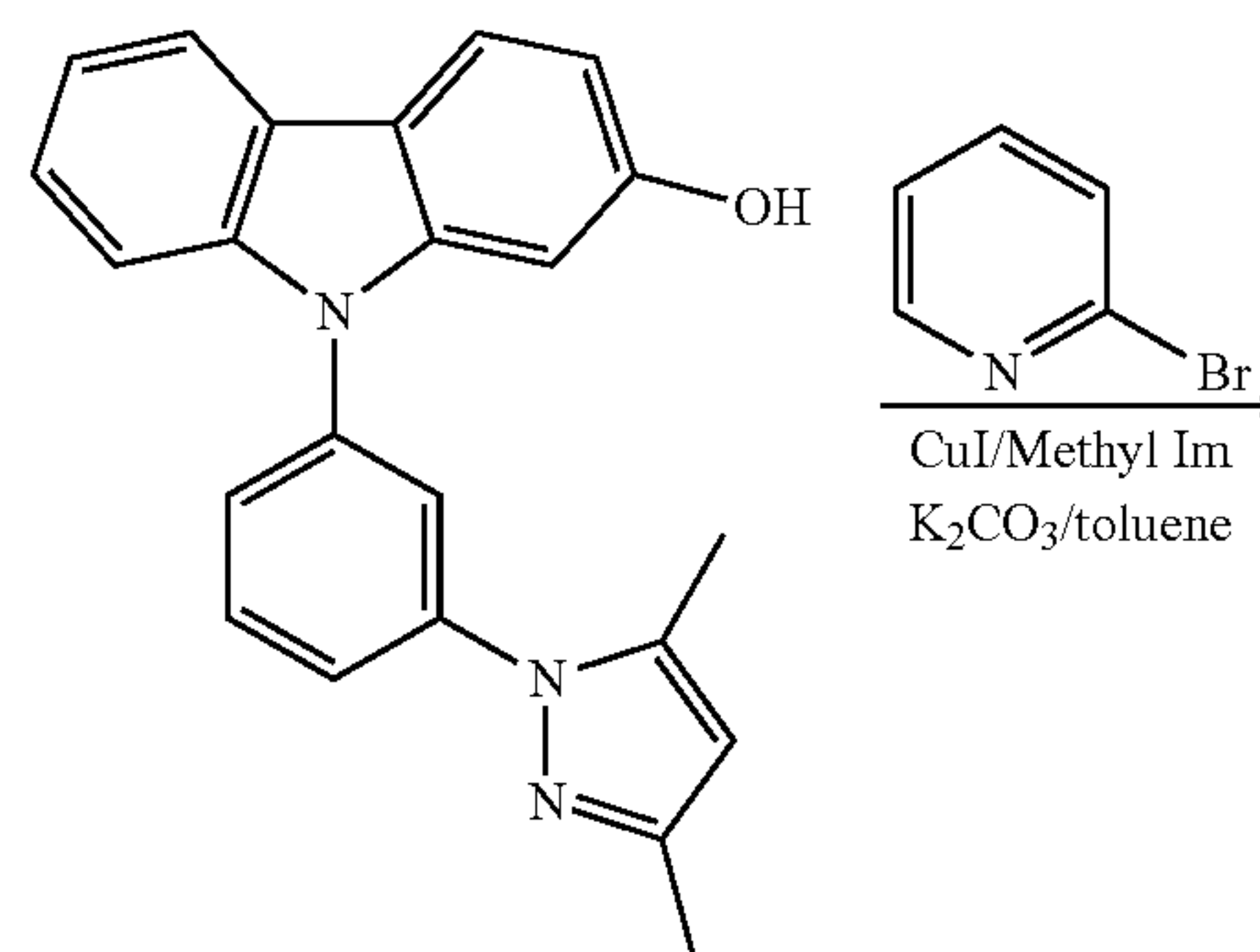
N-(3,5-Dimethylpyrazol-1-yl)-2- hydroxycarbazole
