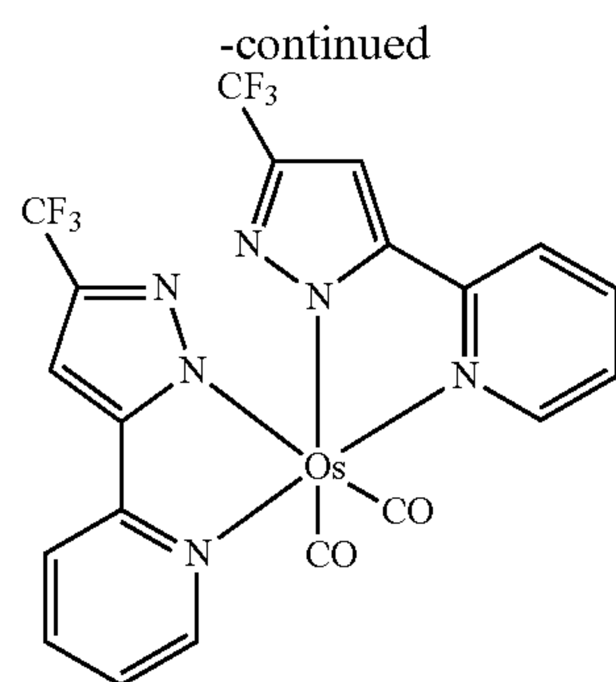
Os(fppz) 2 (CO) 2
