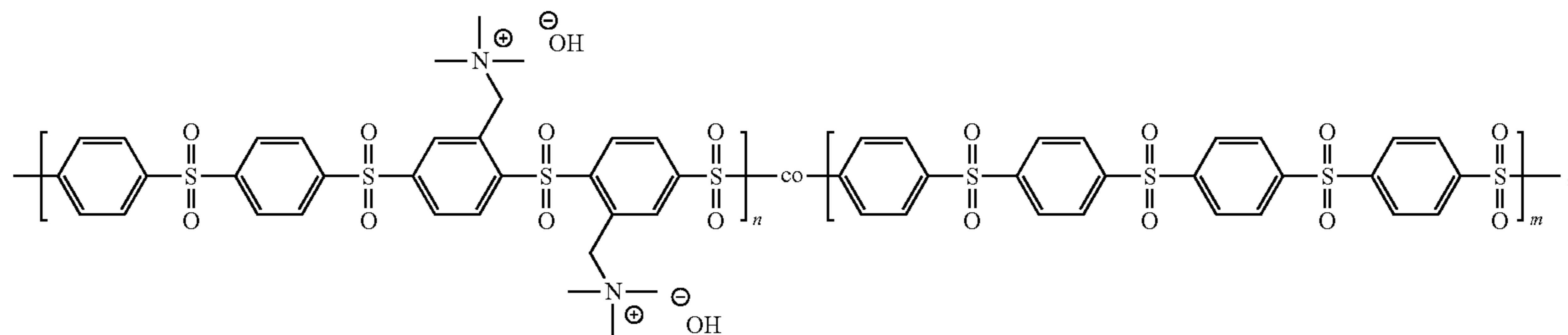
Copolymer 4
