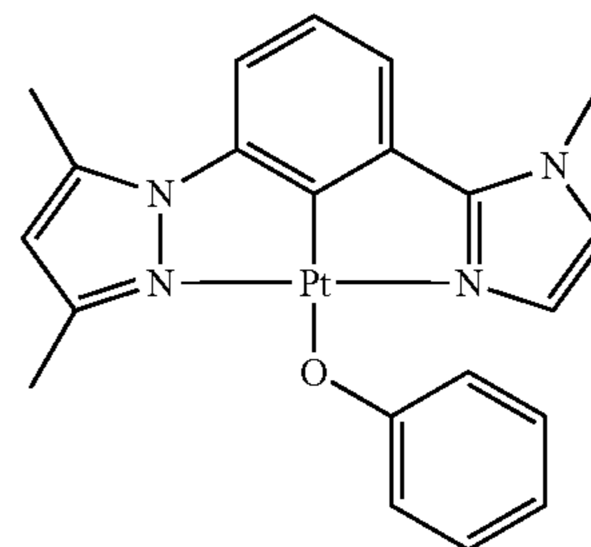
DMPz—Ph—MIz—PtOPh
