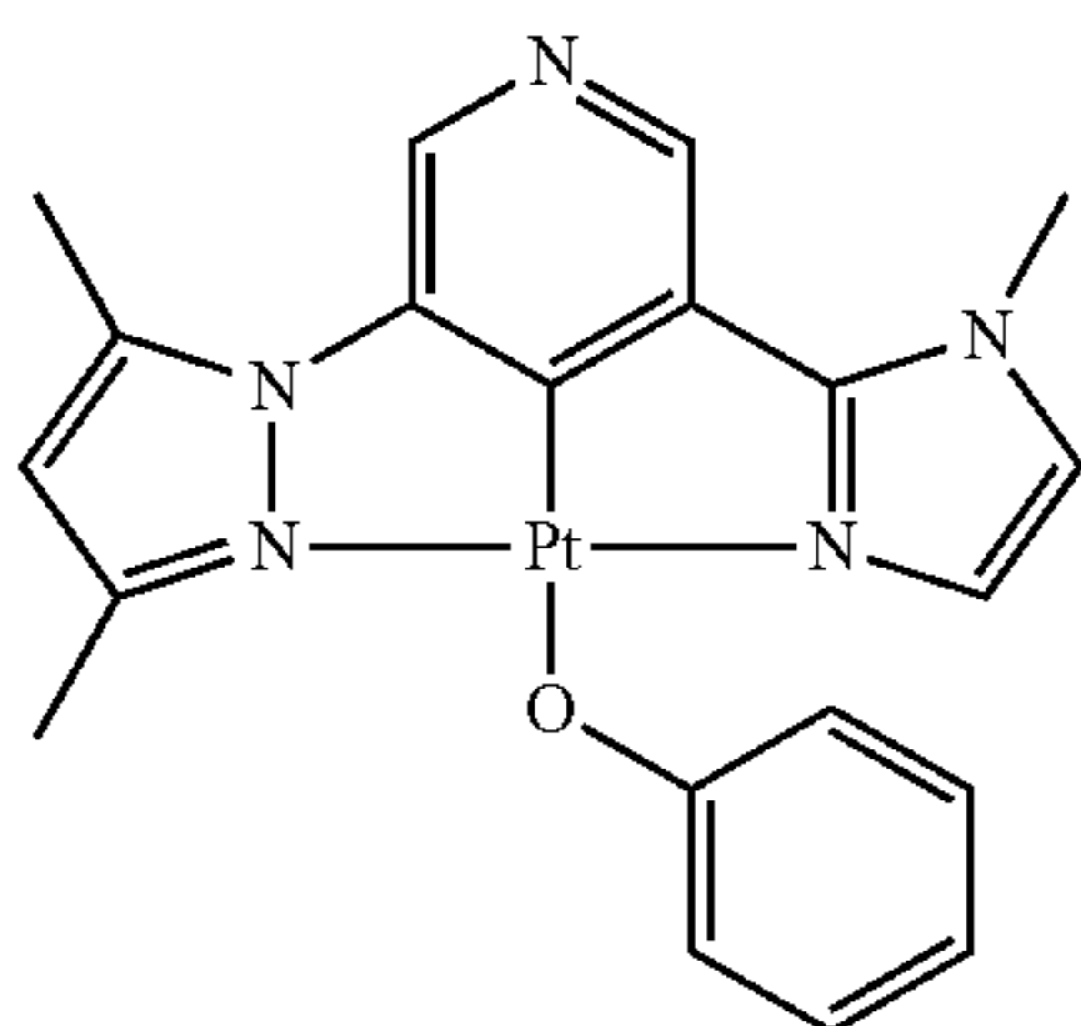
DMPz—Py—MIz—PtOPh
