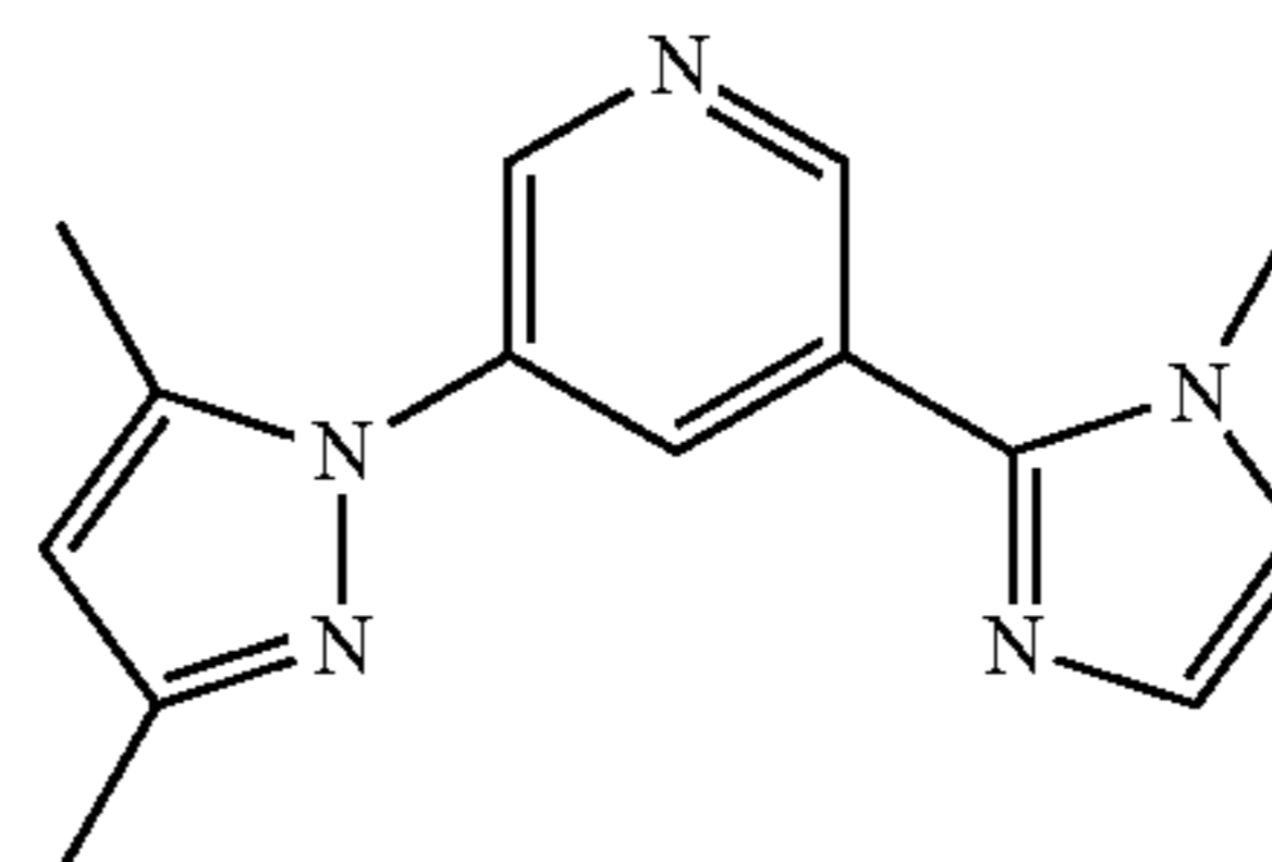
DMPz—Py—MIz
