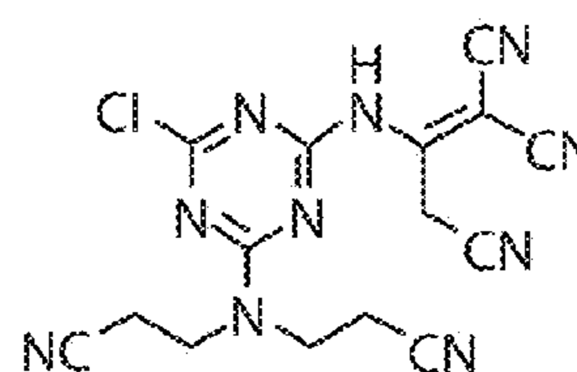
2-((4-(bis(2-cyanoethyl)amino)-6-chloro-1,3,5-triazin-2-yl)amino)prop-1-ene-1,1,3-tricarbonitrile
