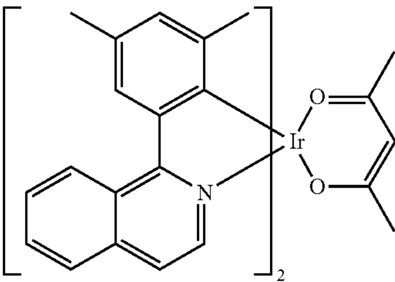
Btp 2 Ir(acac)
