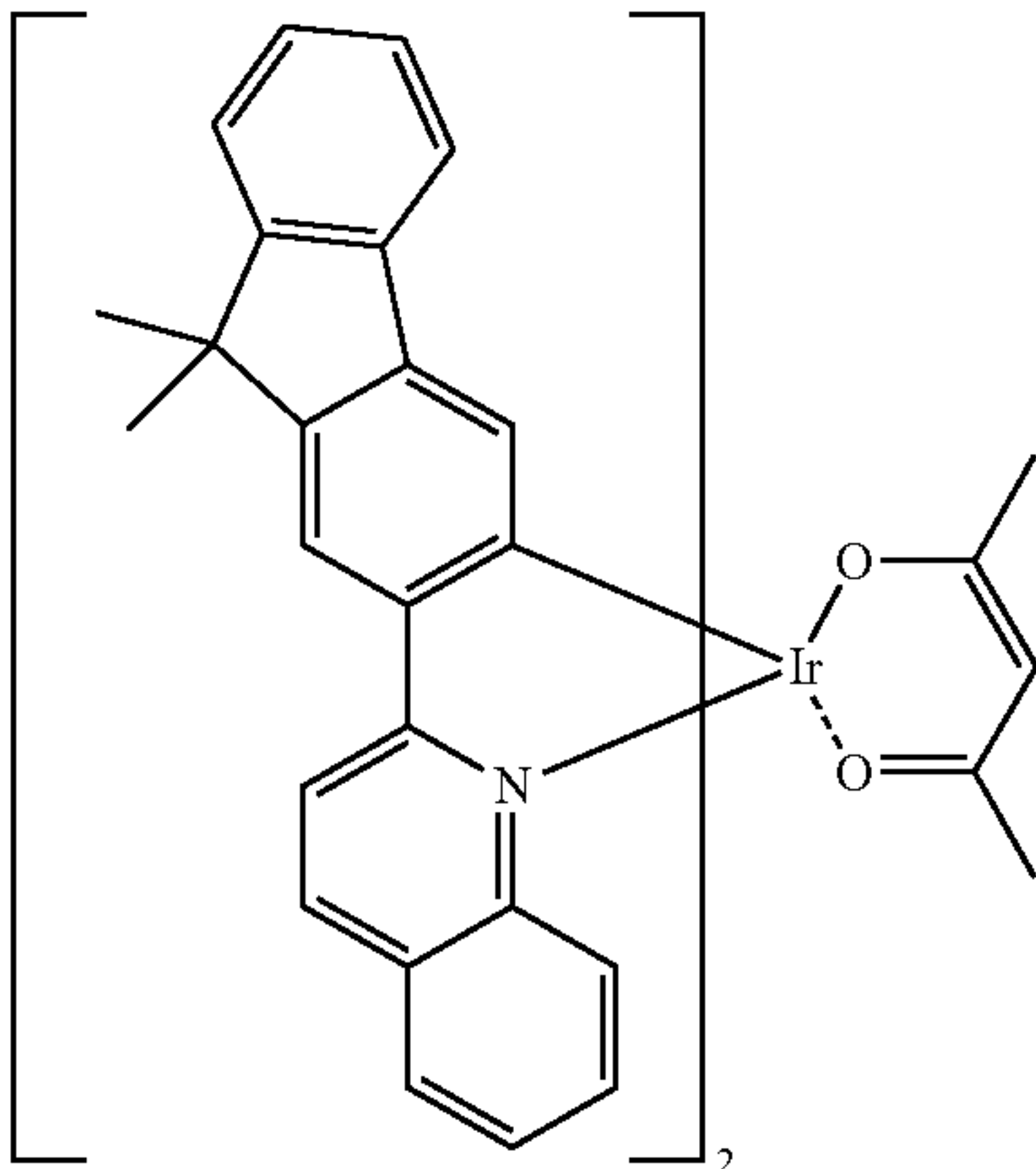
Ir(flq) 2 (acac)
