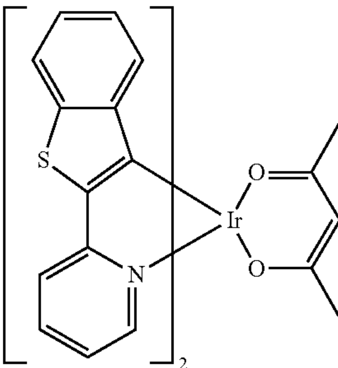
Btp 2 Ir(acac)
