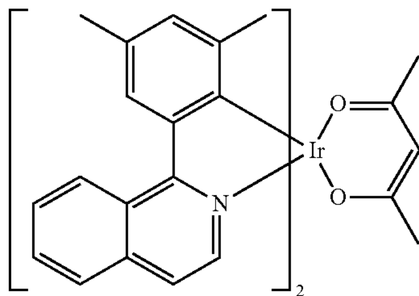
Btp 2 Ir(acac)
