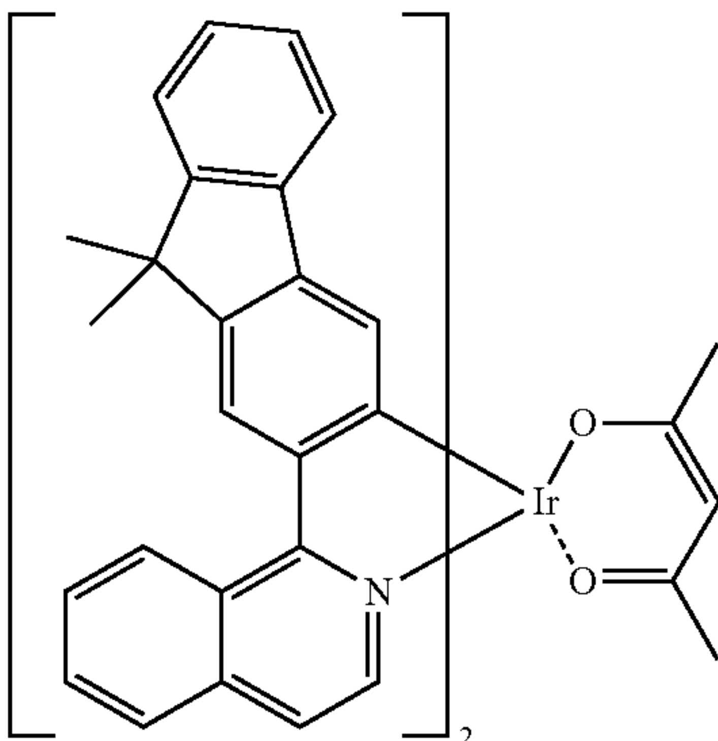
Ir(fliq) 2 (acac)
