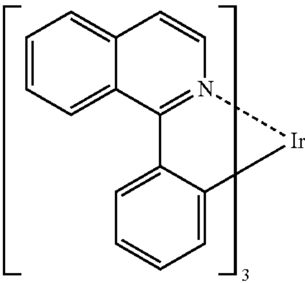
Ir(piq) 3
