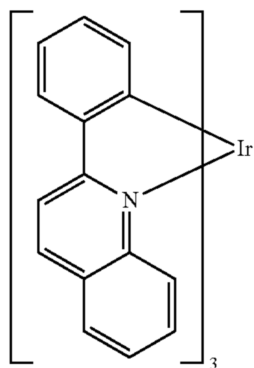
Ir(2-phq) 3
