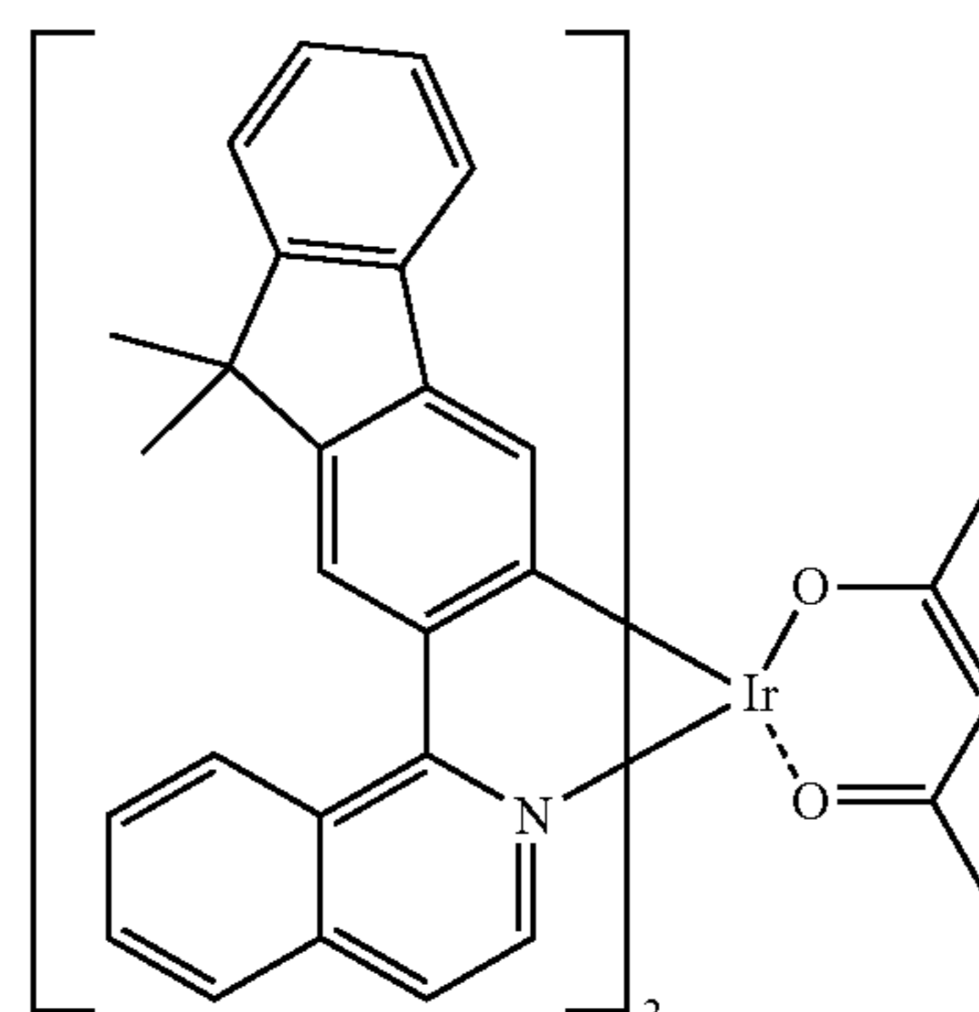
Ir(fliq) 2 (acac)
