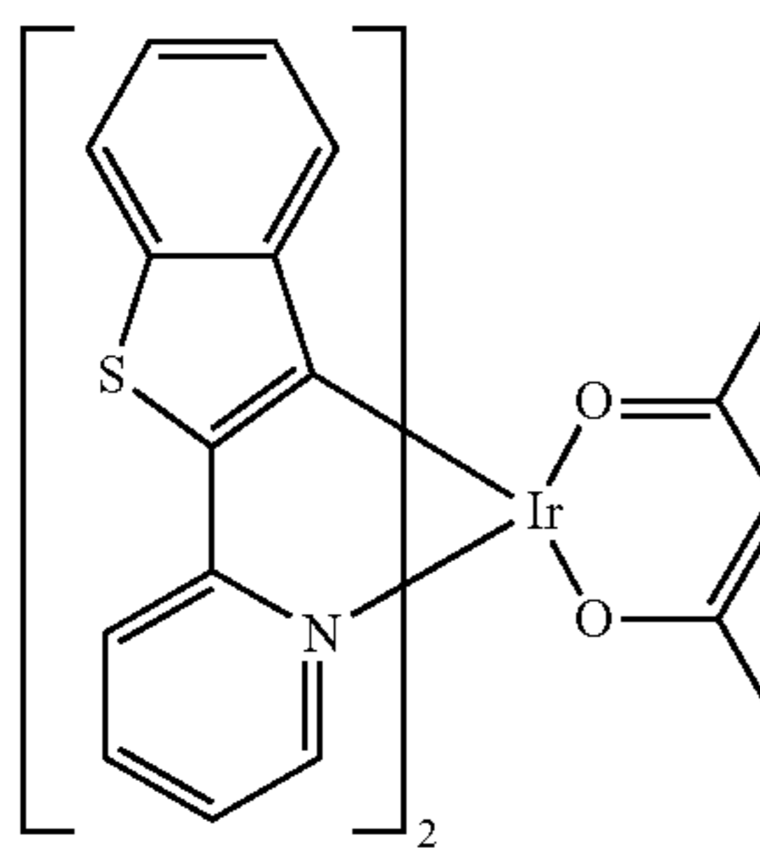
Btp 2 Ir(acac)
