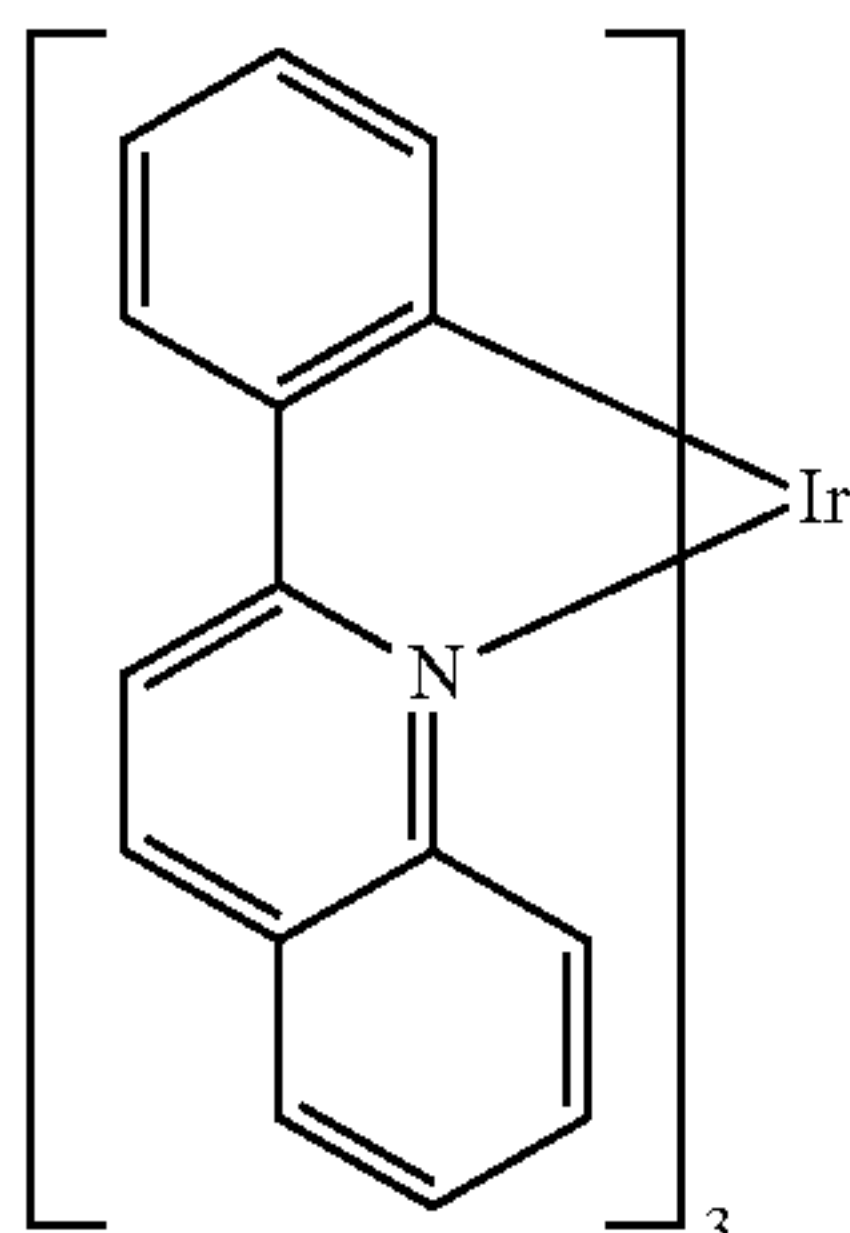
Ir(2-phq) 3
