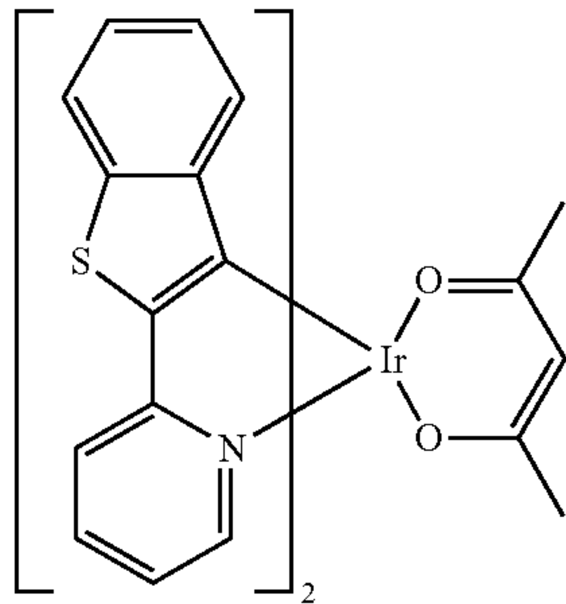
Btp 2 Ir(acac)
