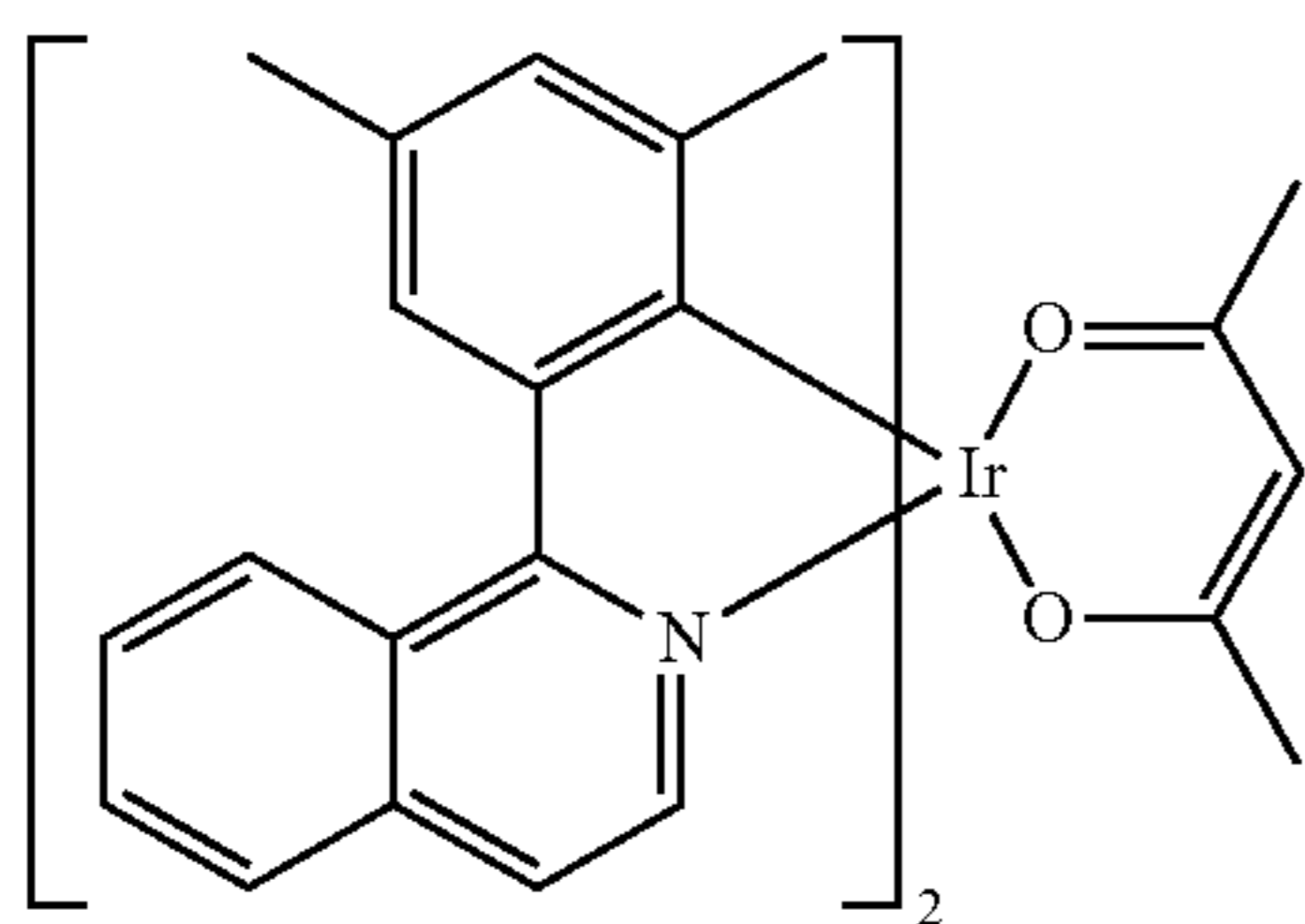
Btp 2 Ir(acac)
