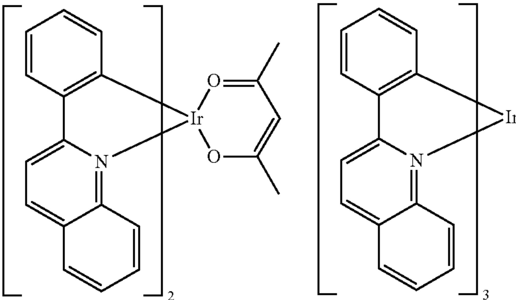
Ir(pq) 2 (acac)
