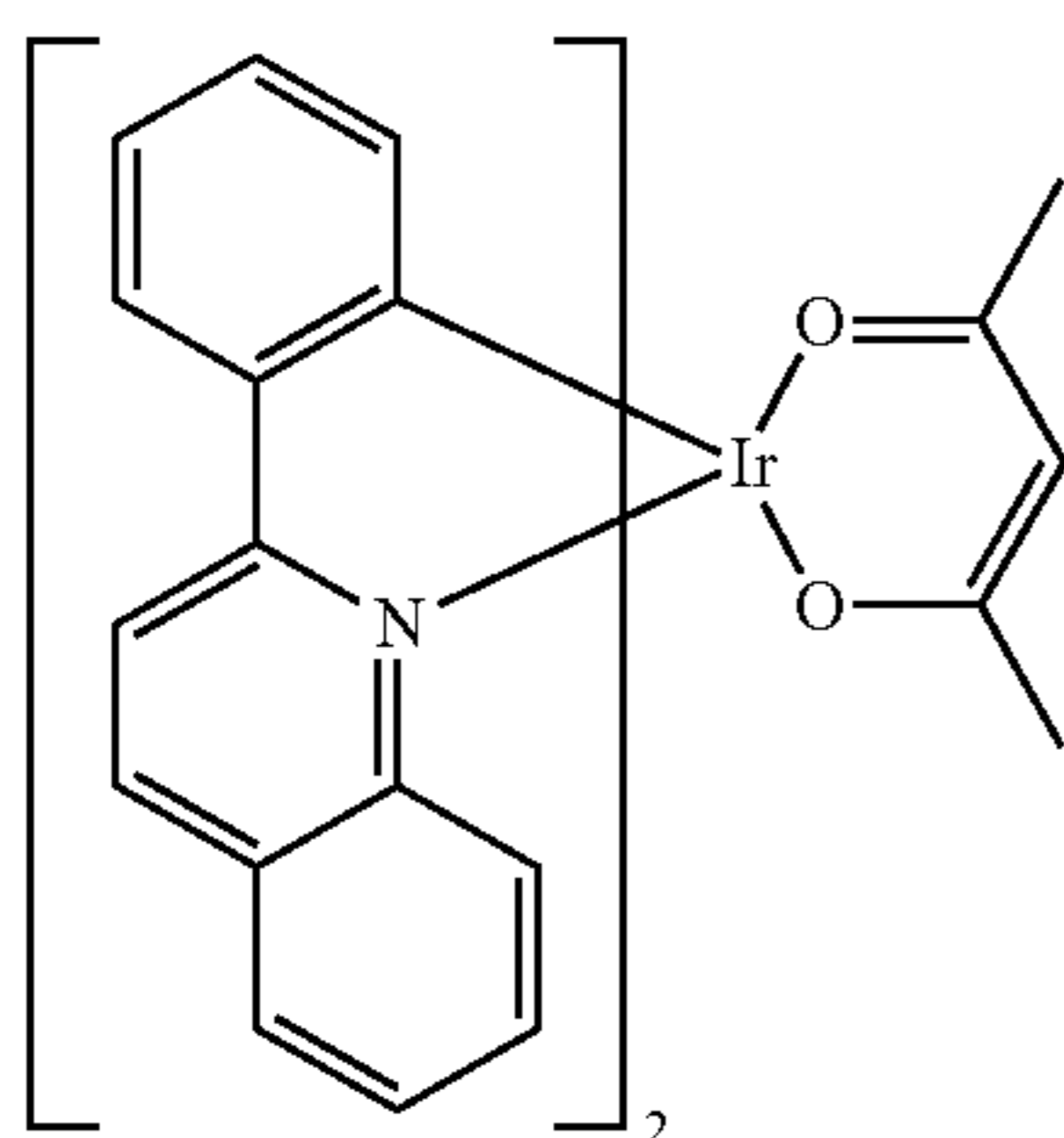
Ir(pq) 2 (acac)
