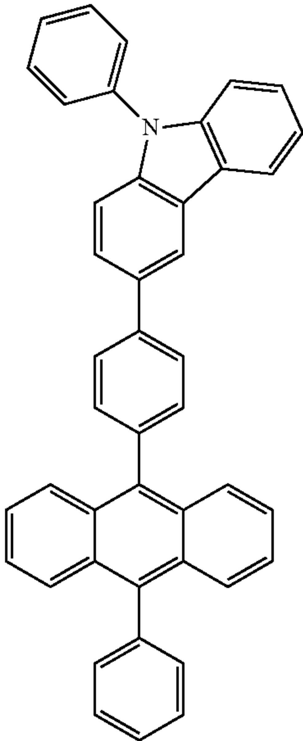
PCzPA
