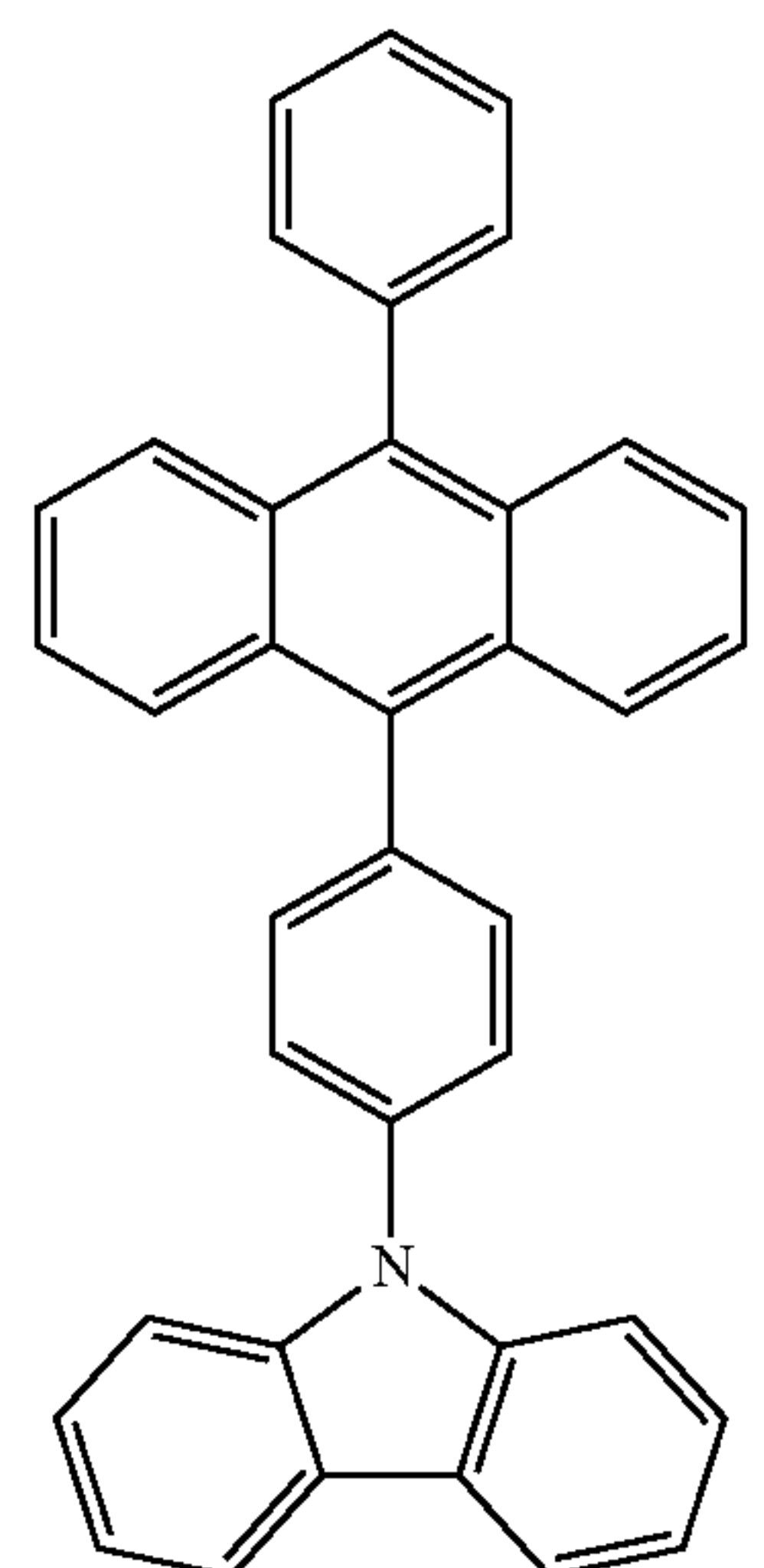
CzPA
