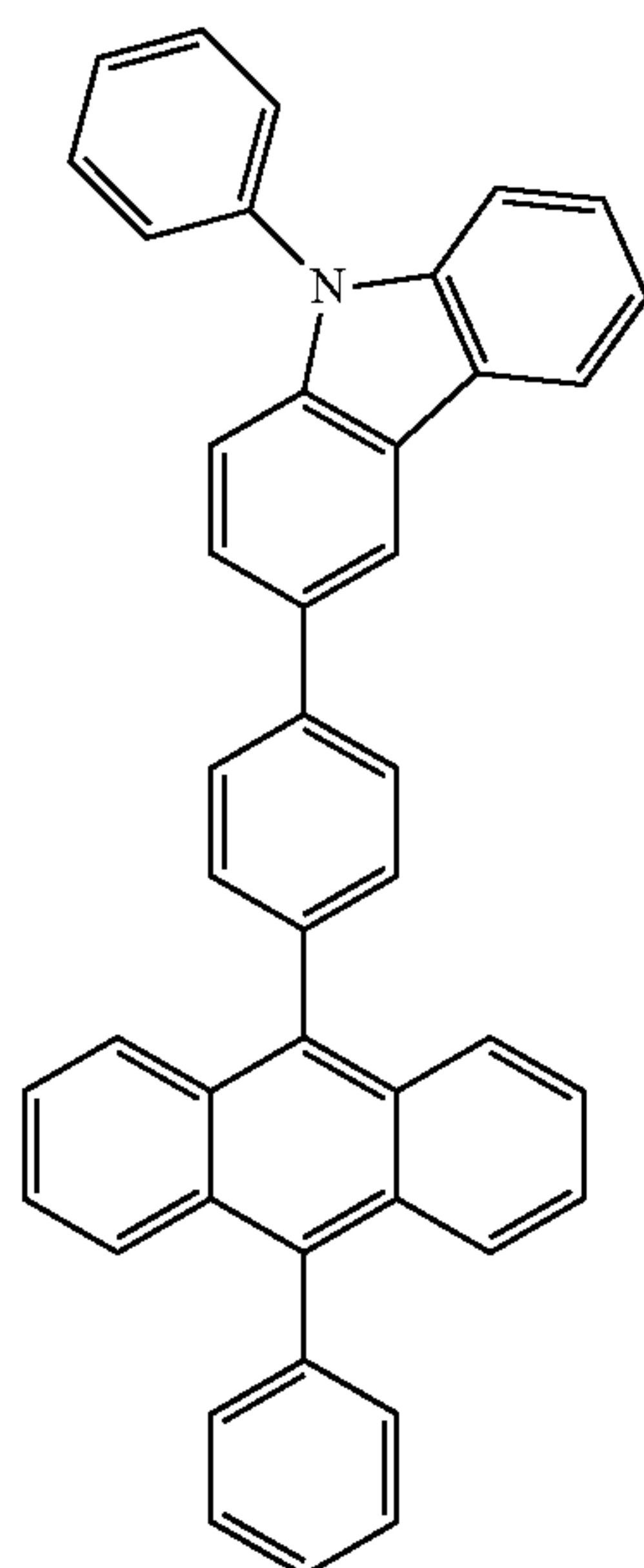
PCzPA
