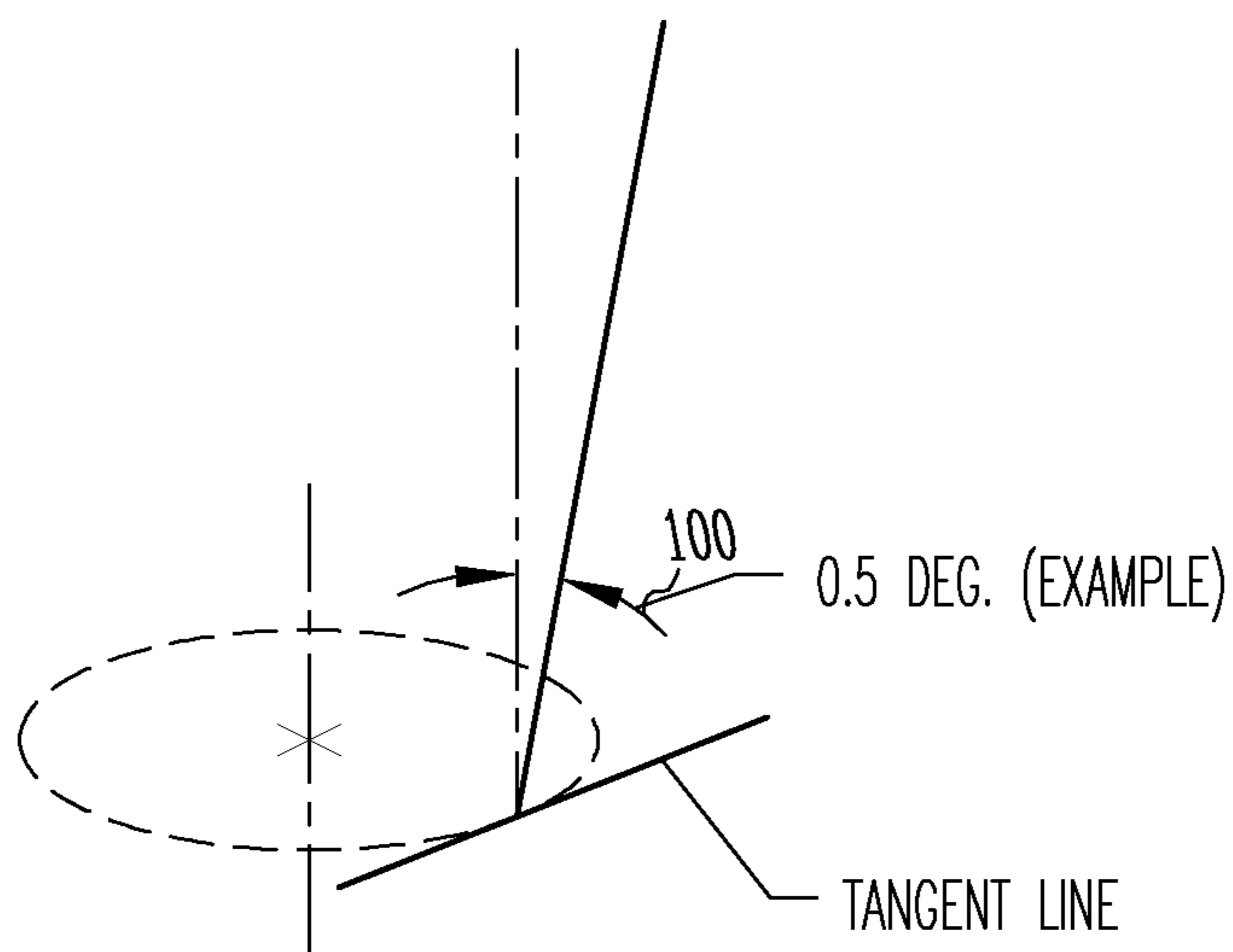
Fig. 3C
