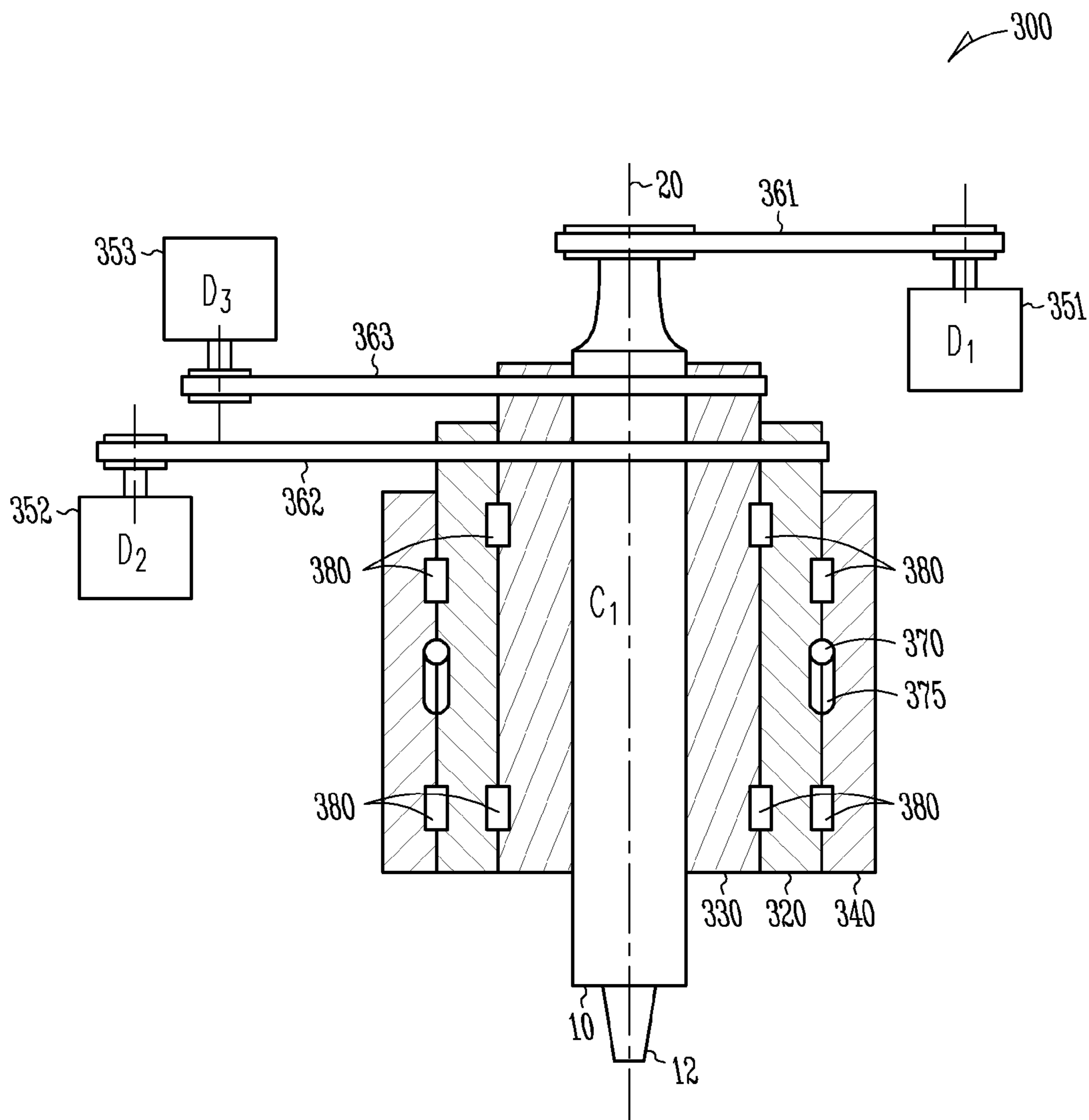
Fig. 3A
