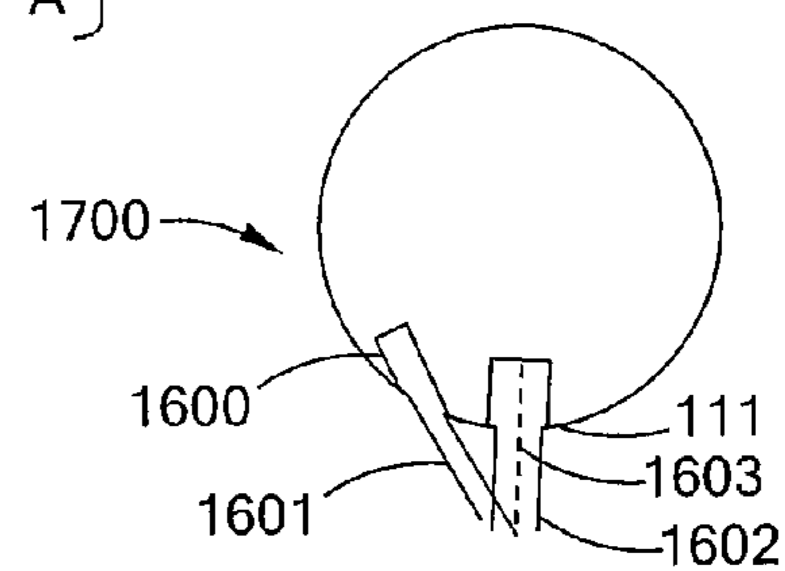
Fig. 16A
