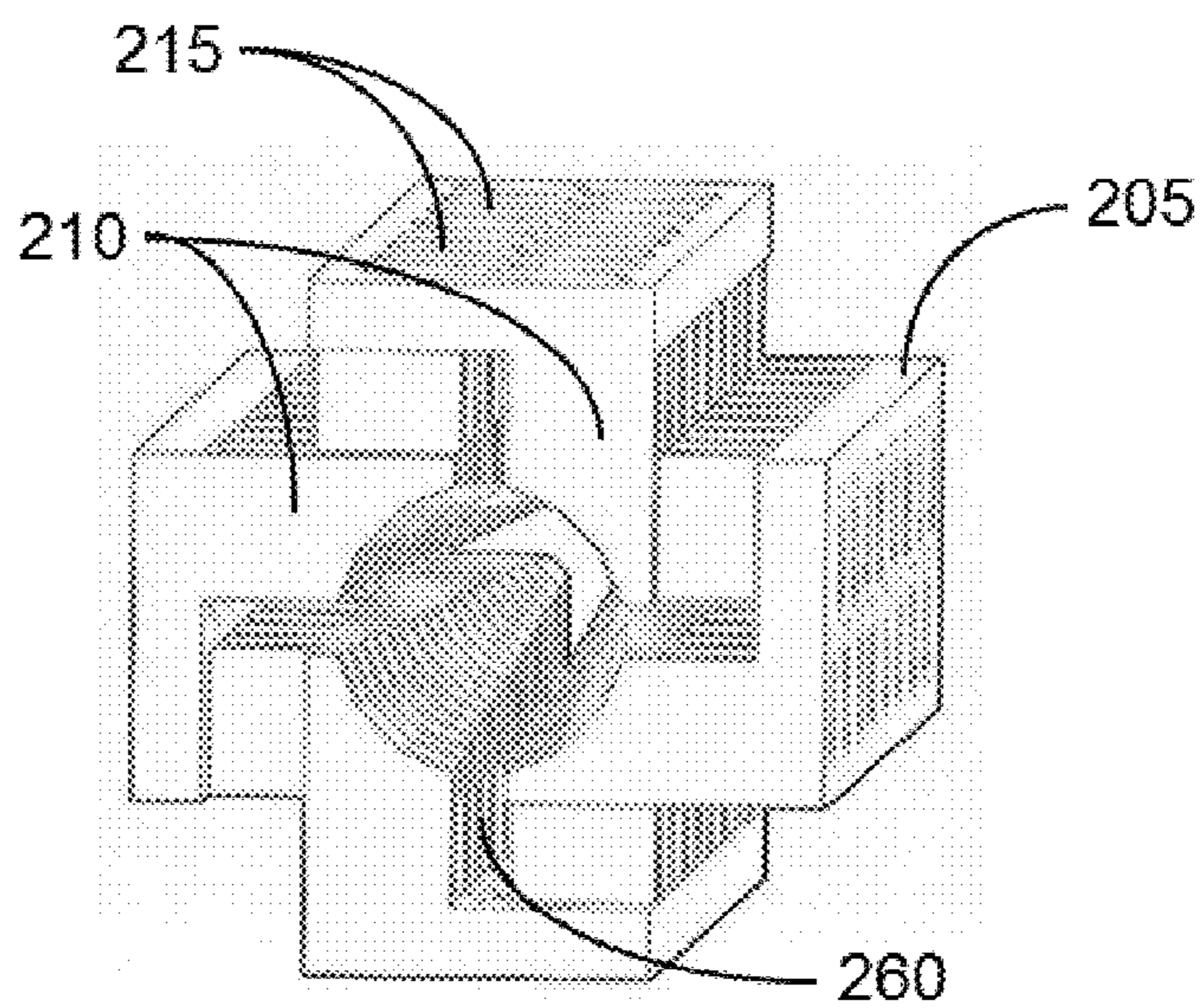
FIG. 2B
