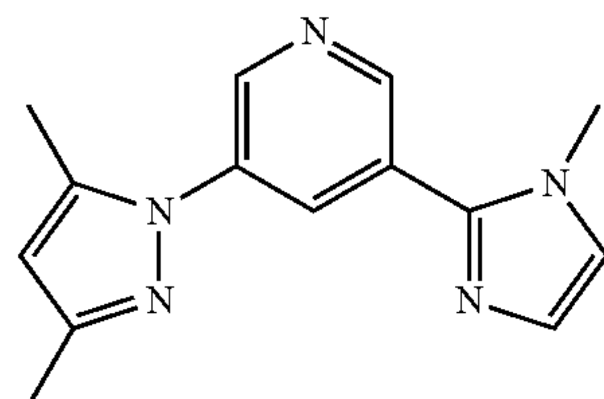
DMPz—Py—MIz
