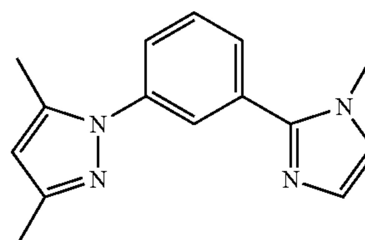
DMPz—Ph—MIz
