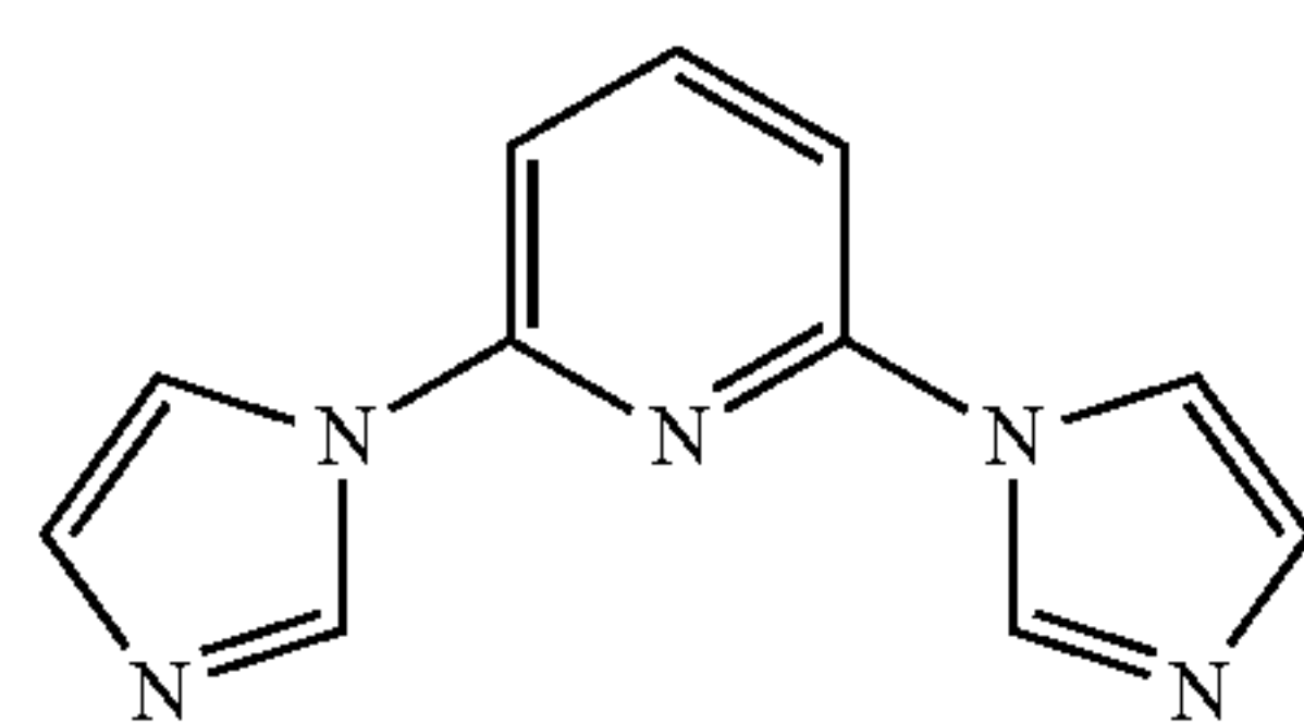
DIz-Py
