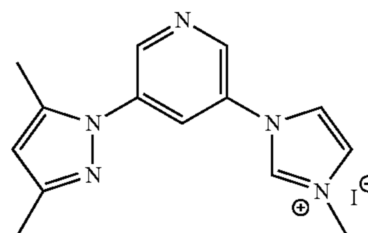
DMPz—Py—IMIz
