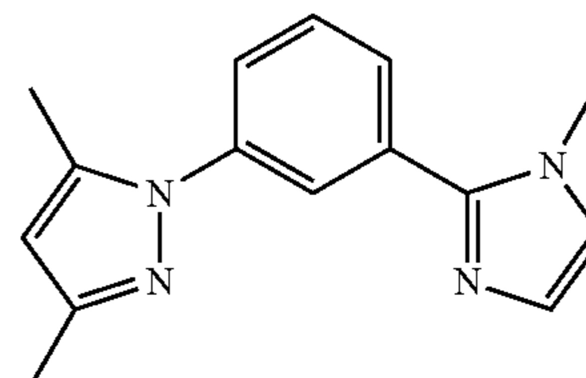
DMPz—Ph—MIz
