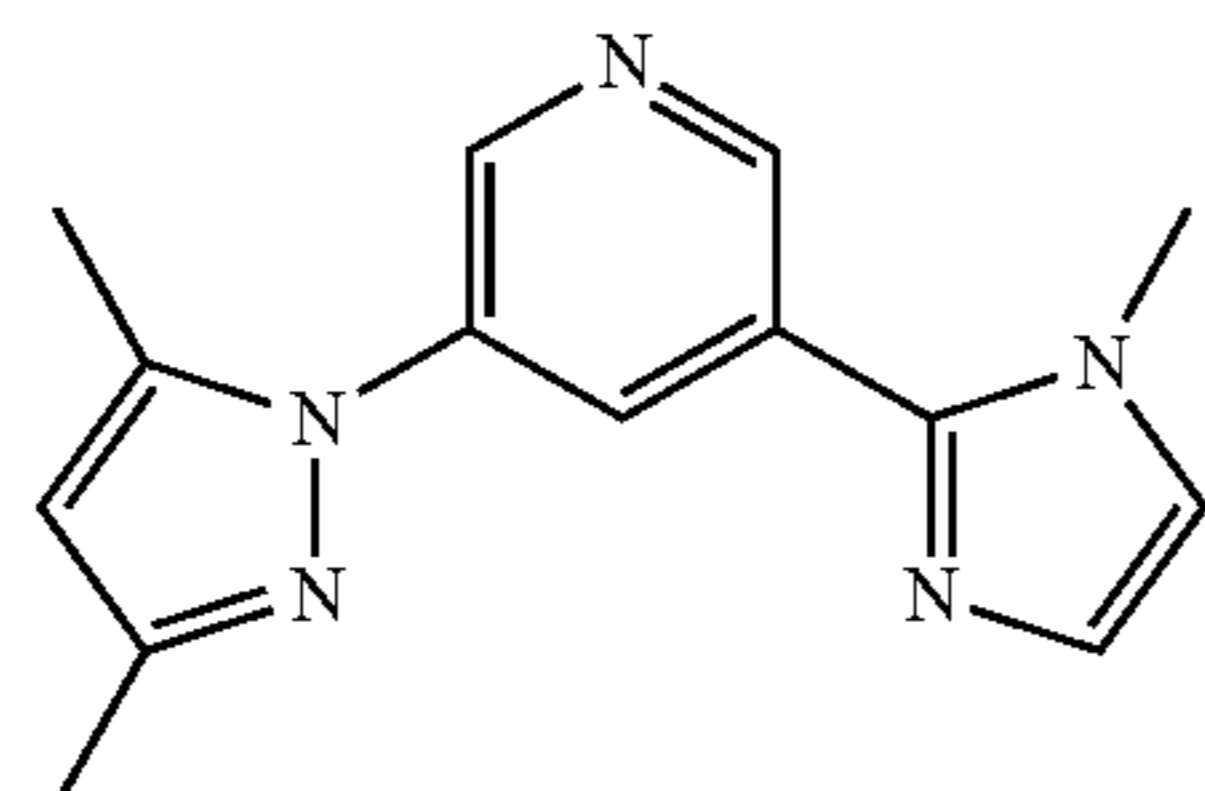
DMPz—Py—MIz
