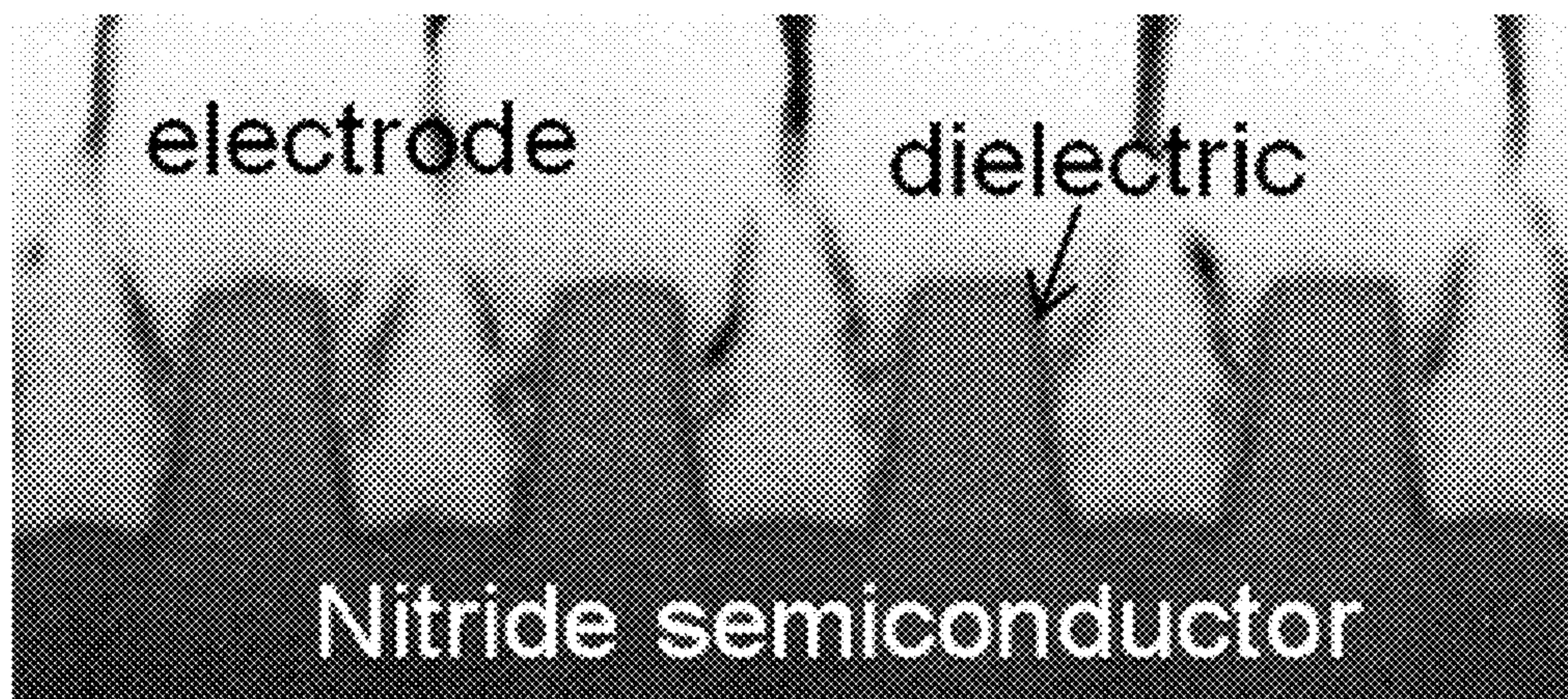
SEM cross section
