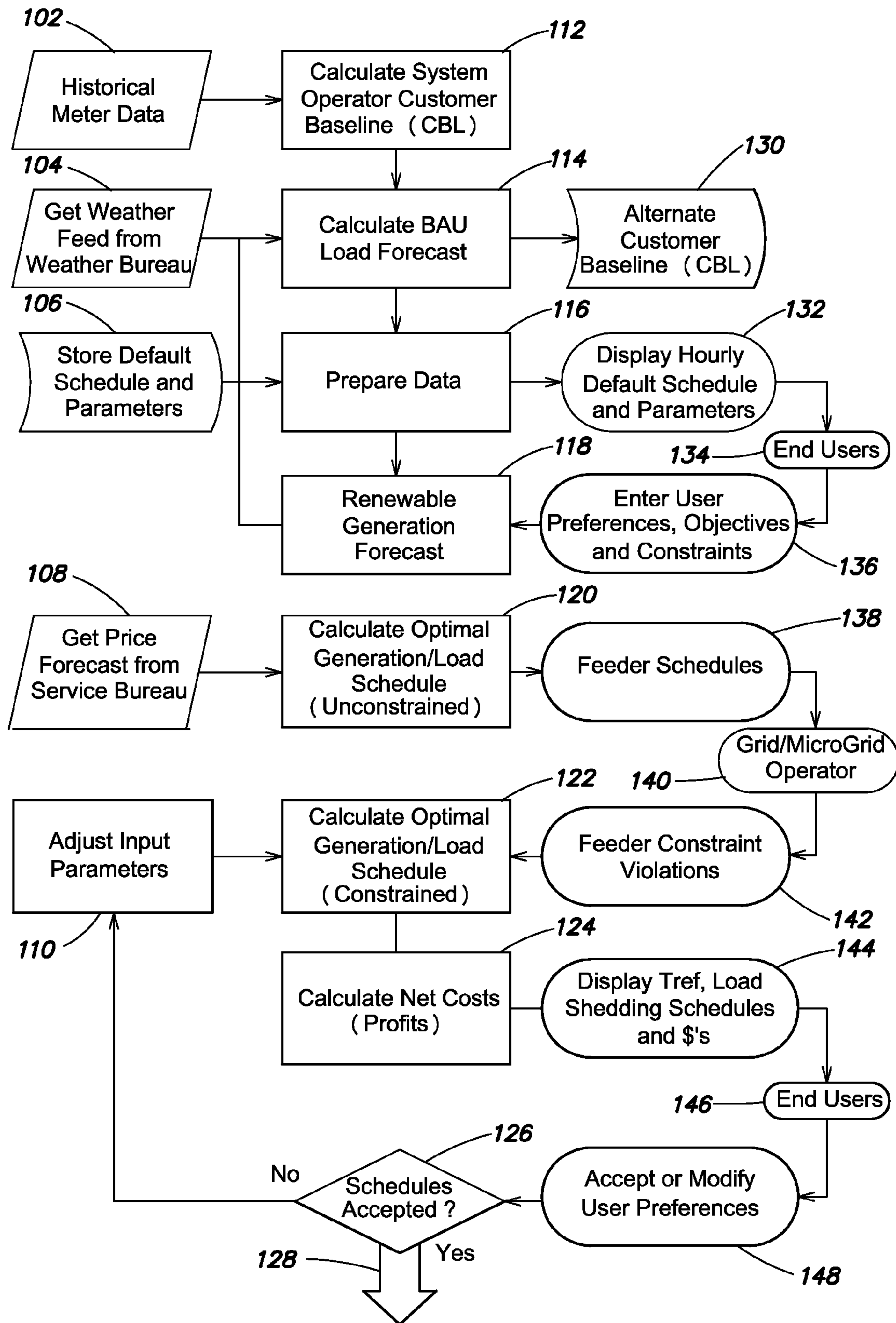
FIG. 14
