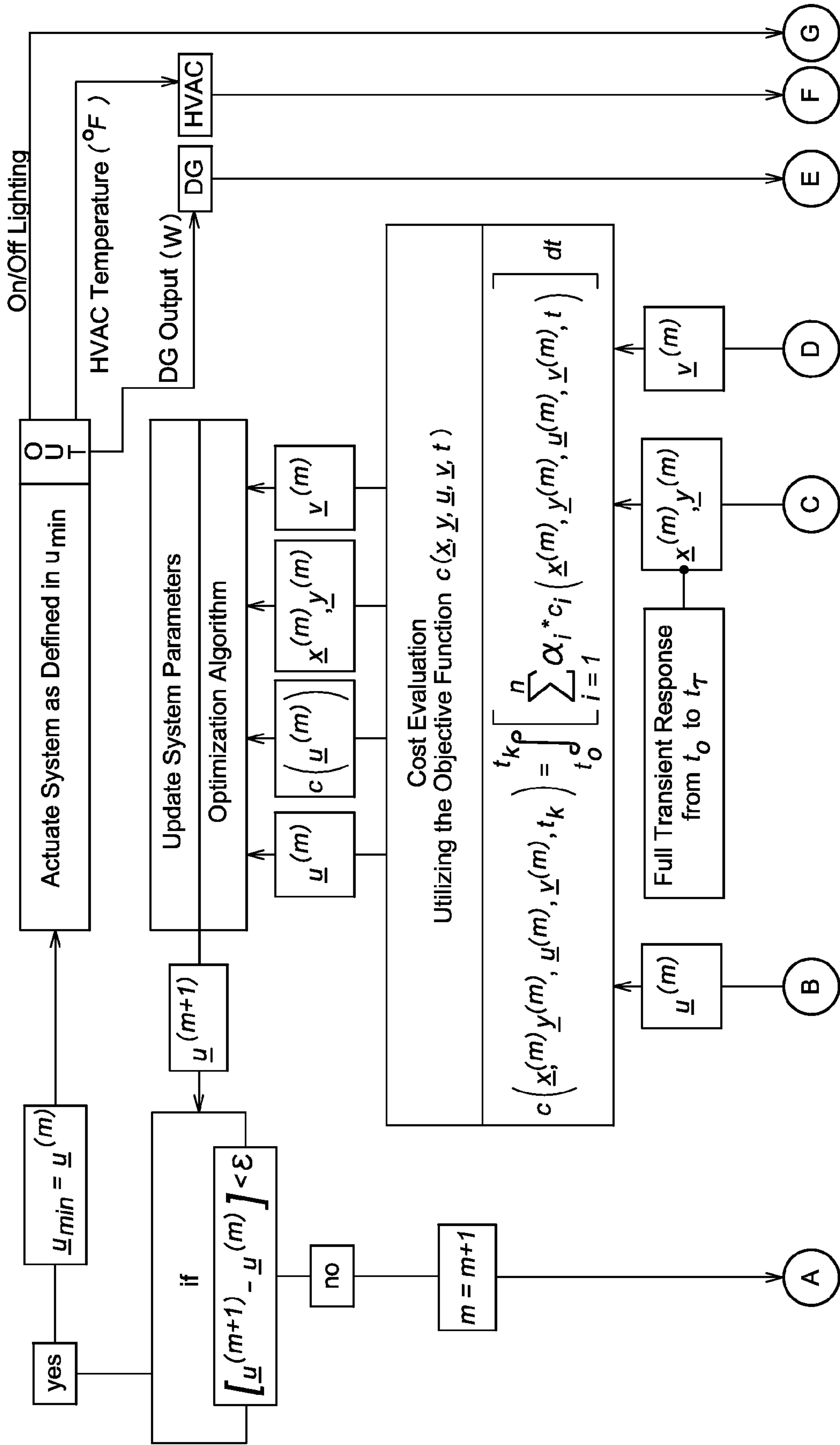
FIG. 17
