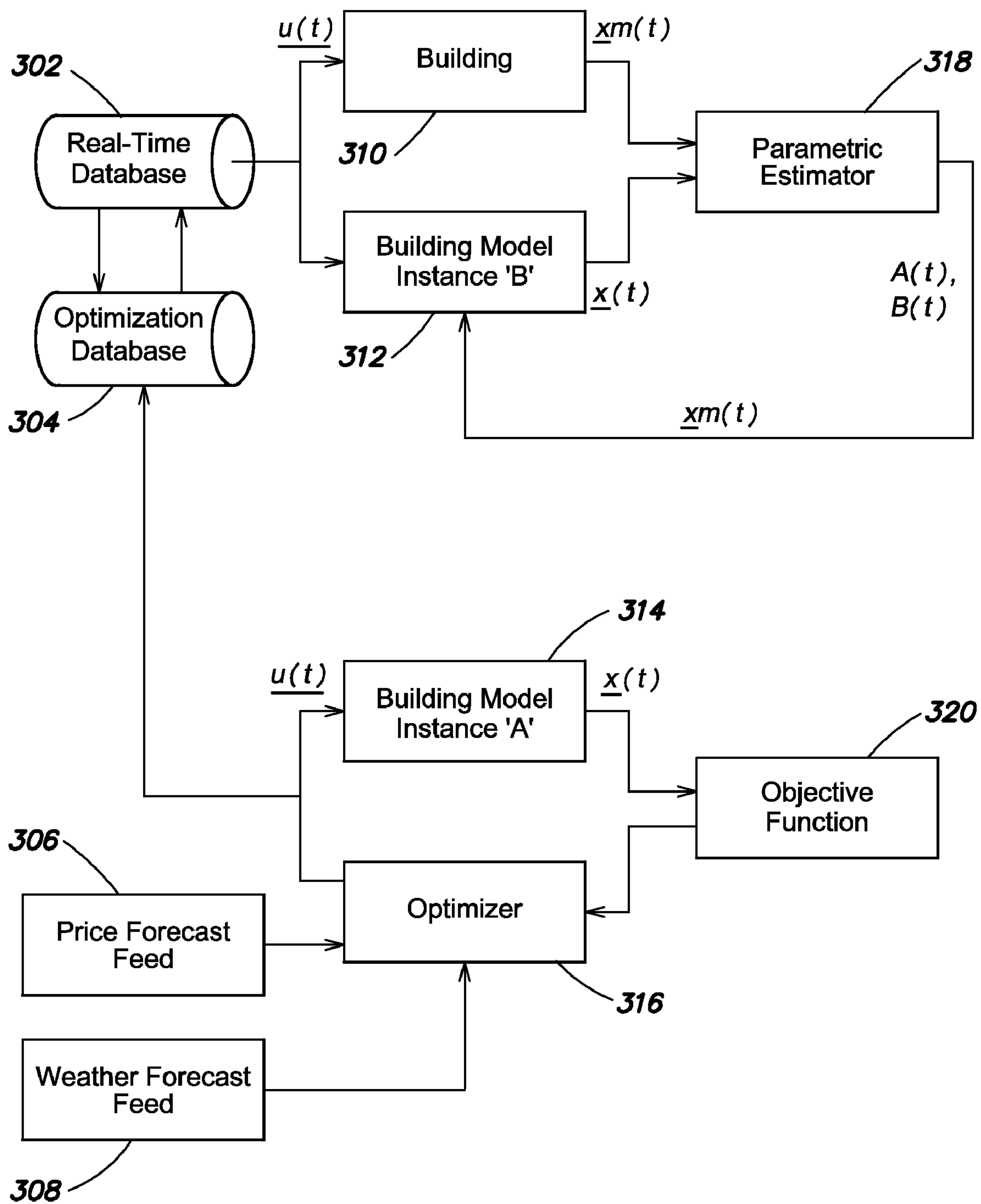
FIG. 16
