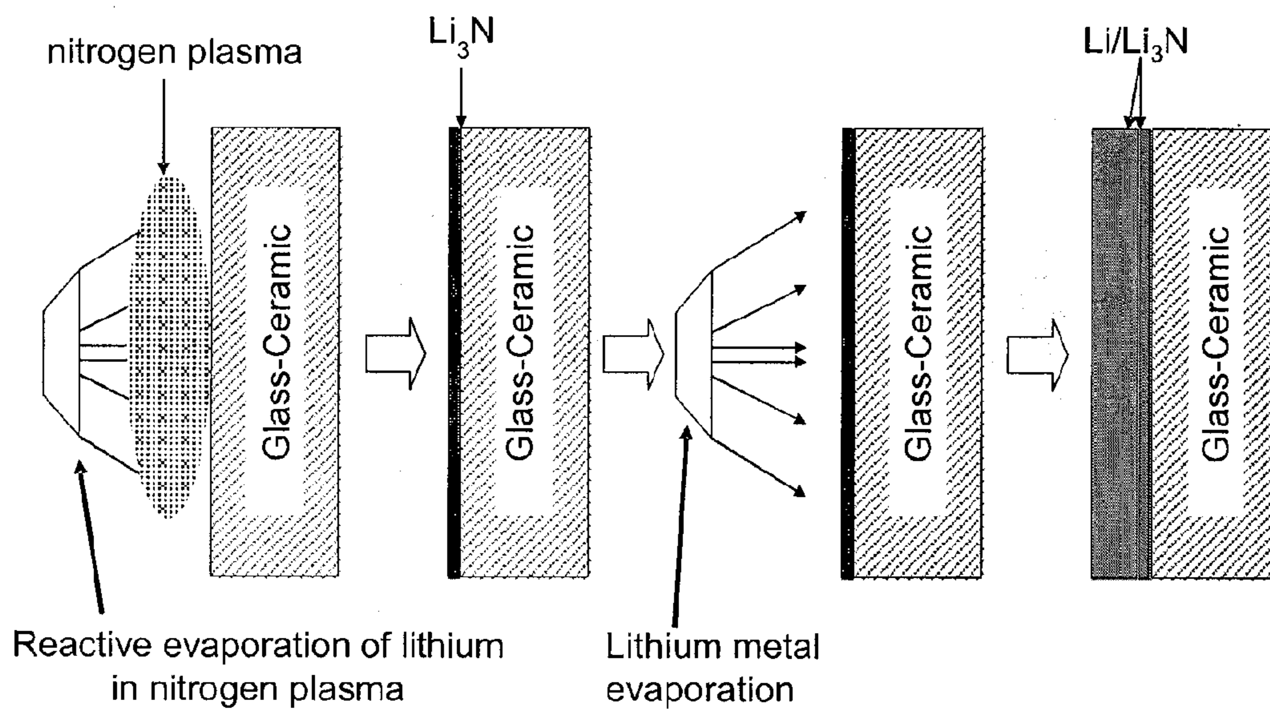
FIG. 4A
