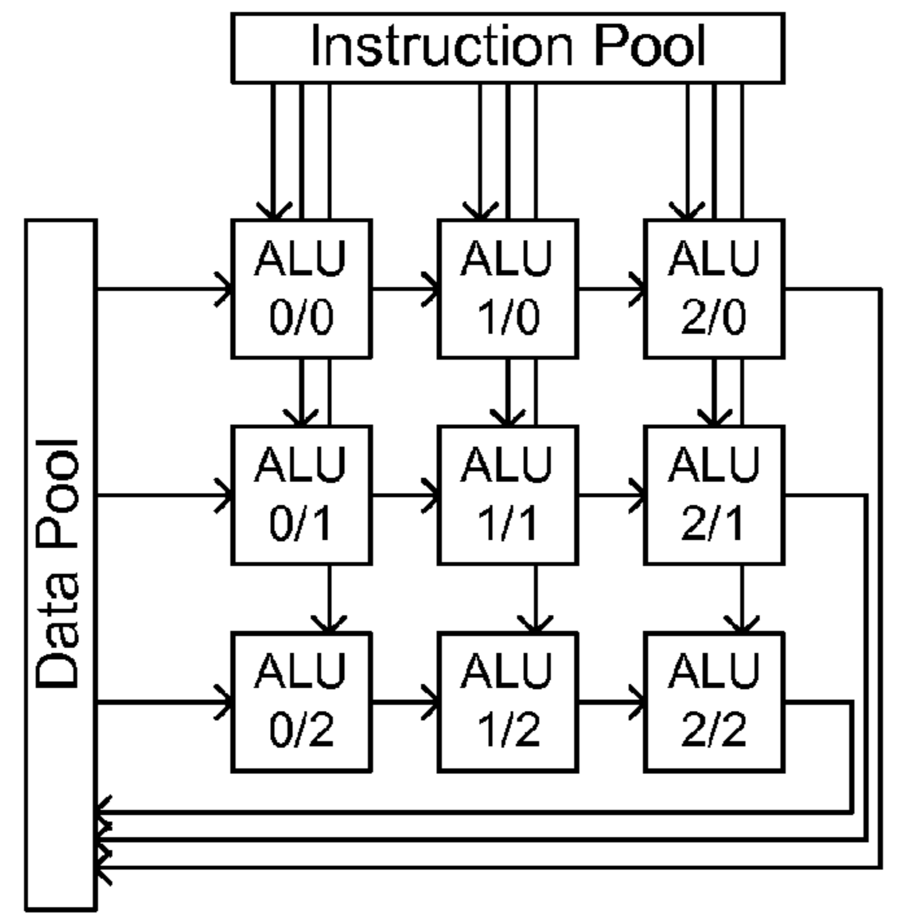
Fig. 3b (matrix)
