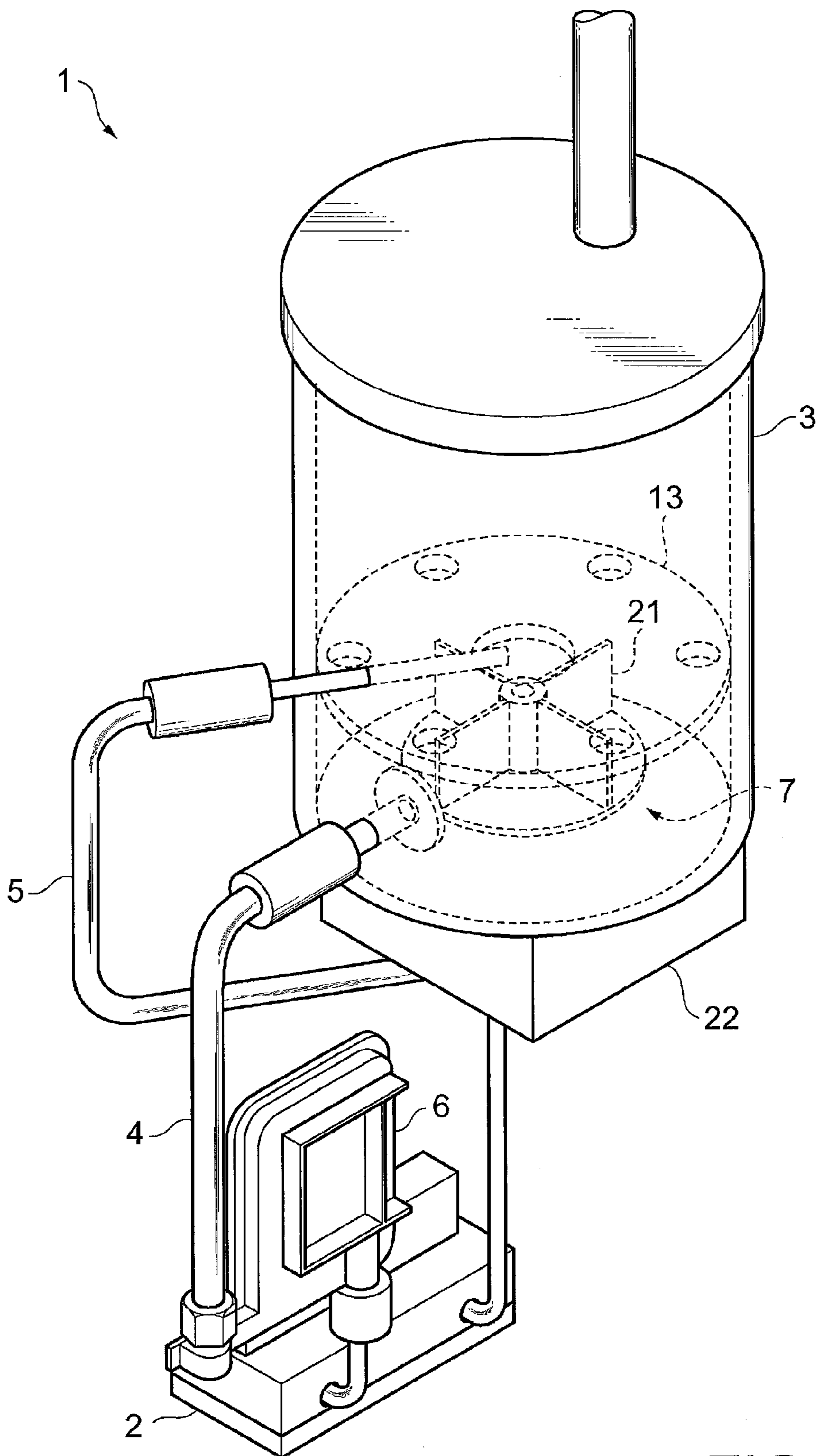
FIG. 1
