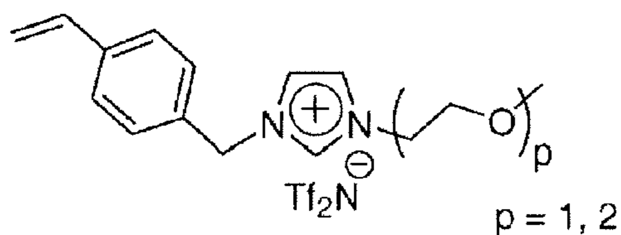
3a, b: OEG p -type
