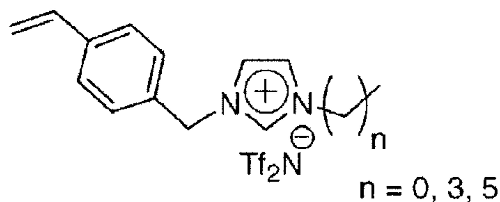
1a - c: C n CH 3 -type
