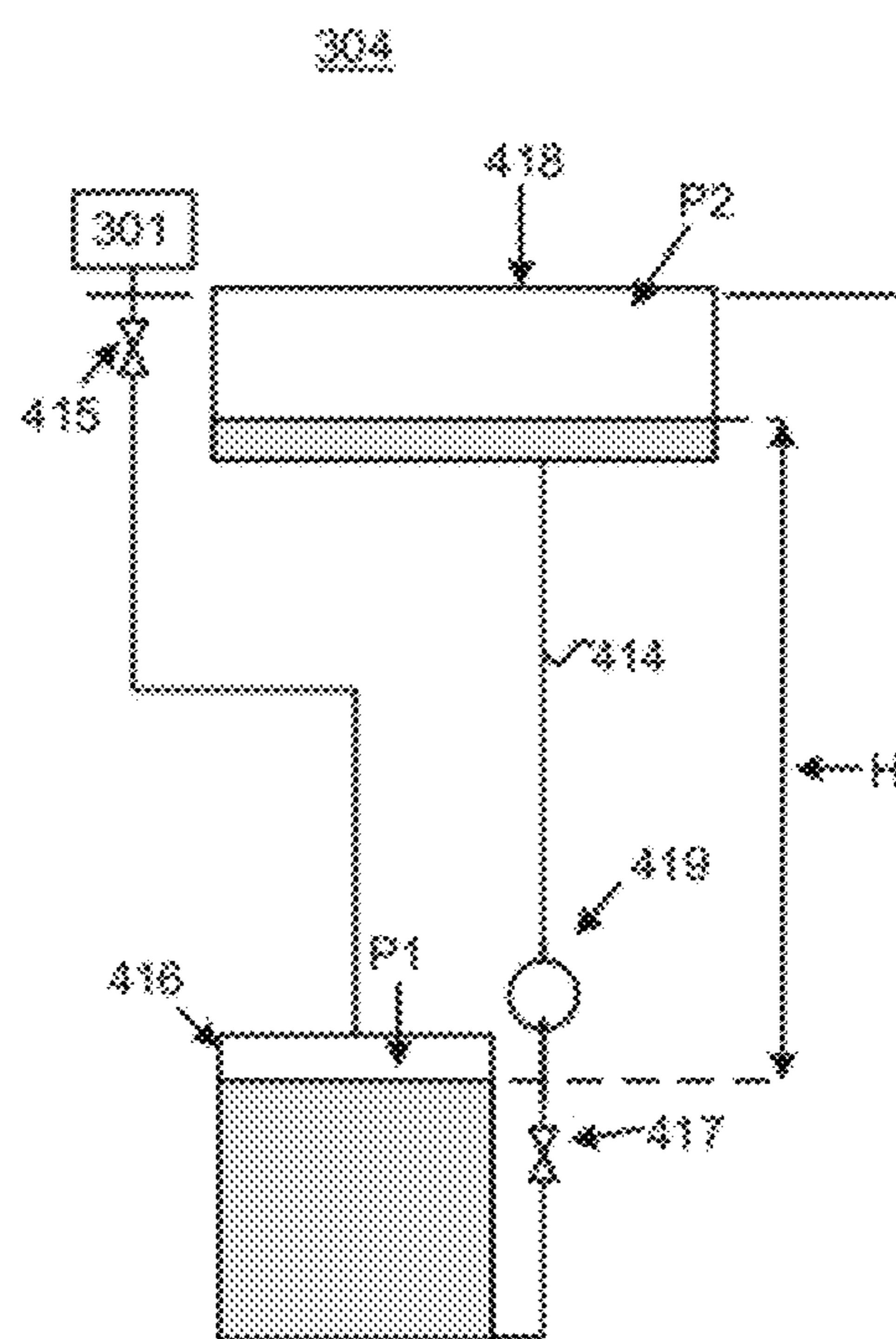
FIG. 4B
