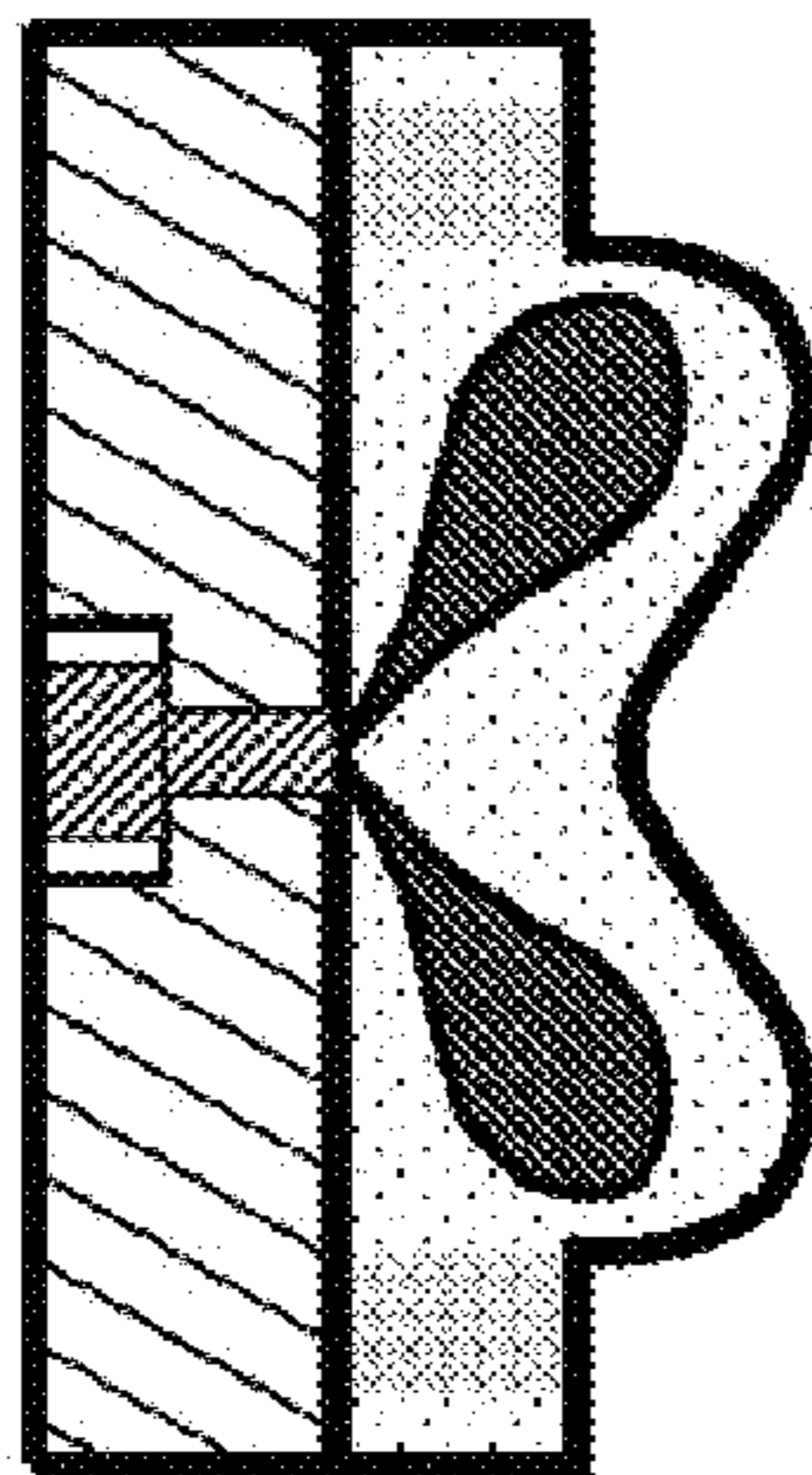
Fig. 1C 30 °BTDC
