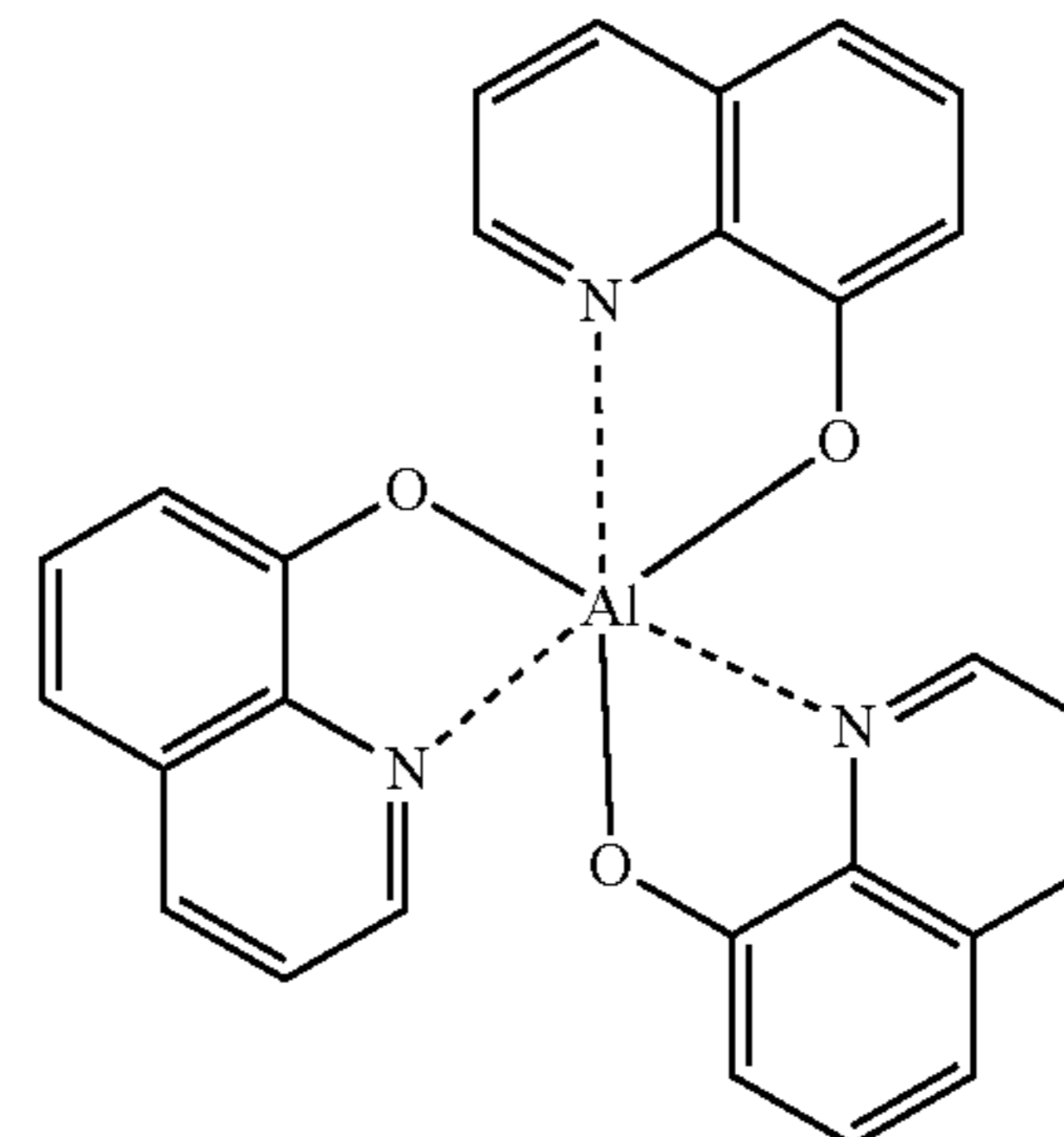
Alq
