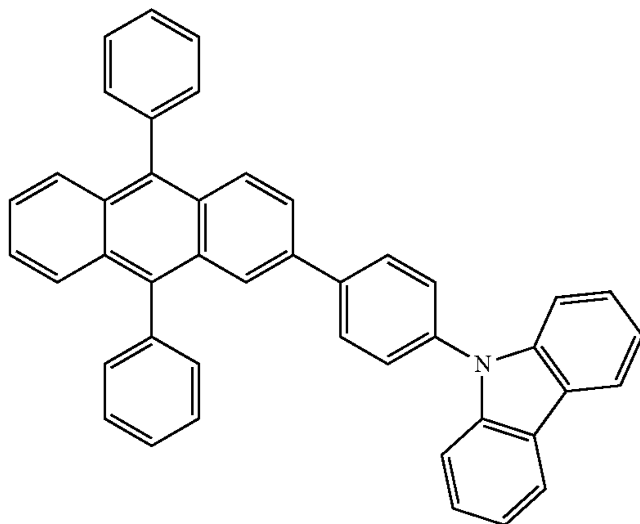
(2CzPPA)
