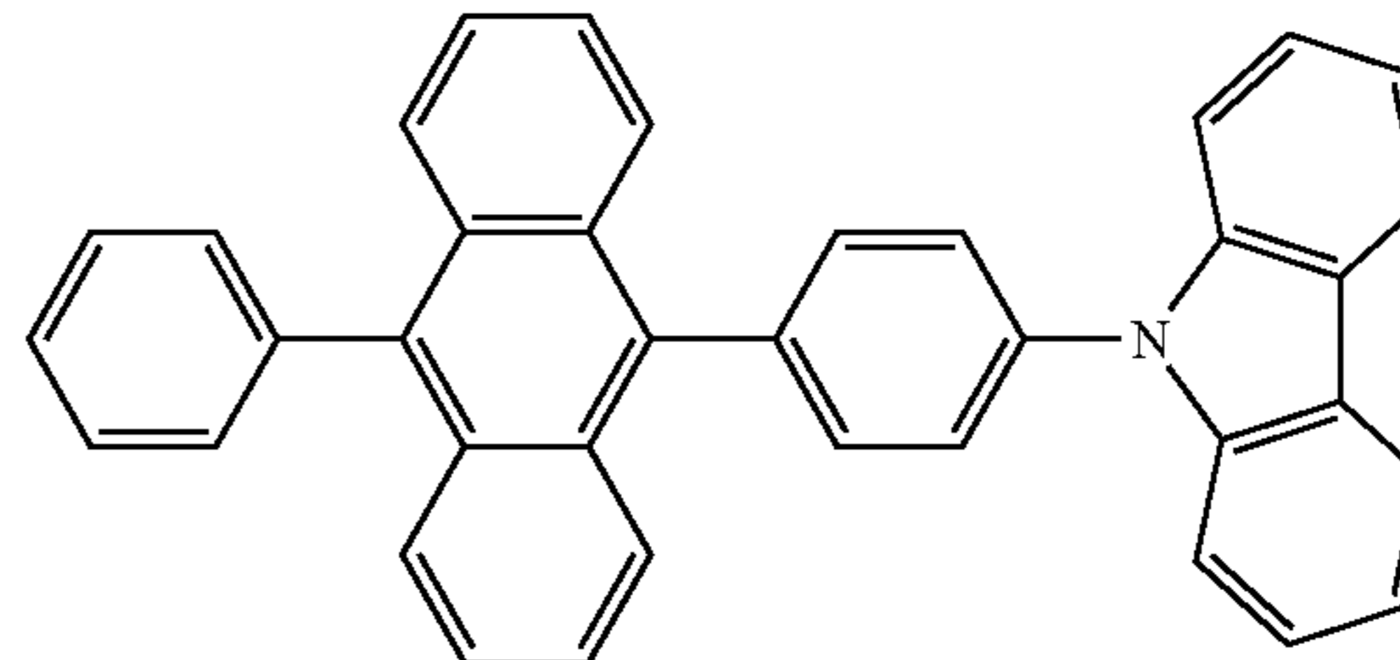
CzPA
