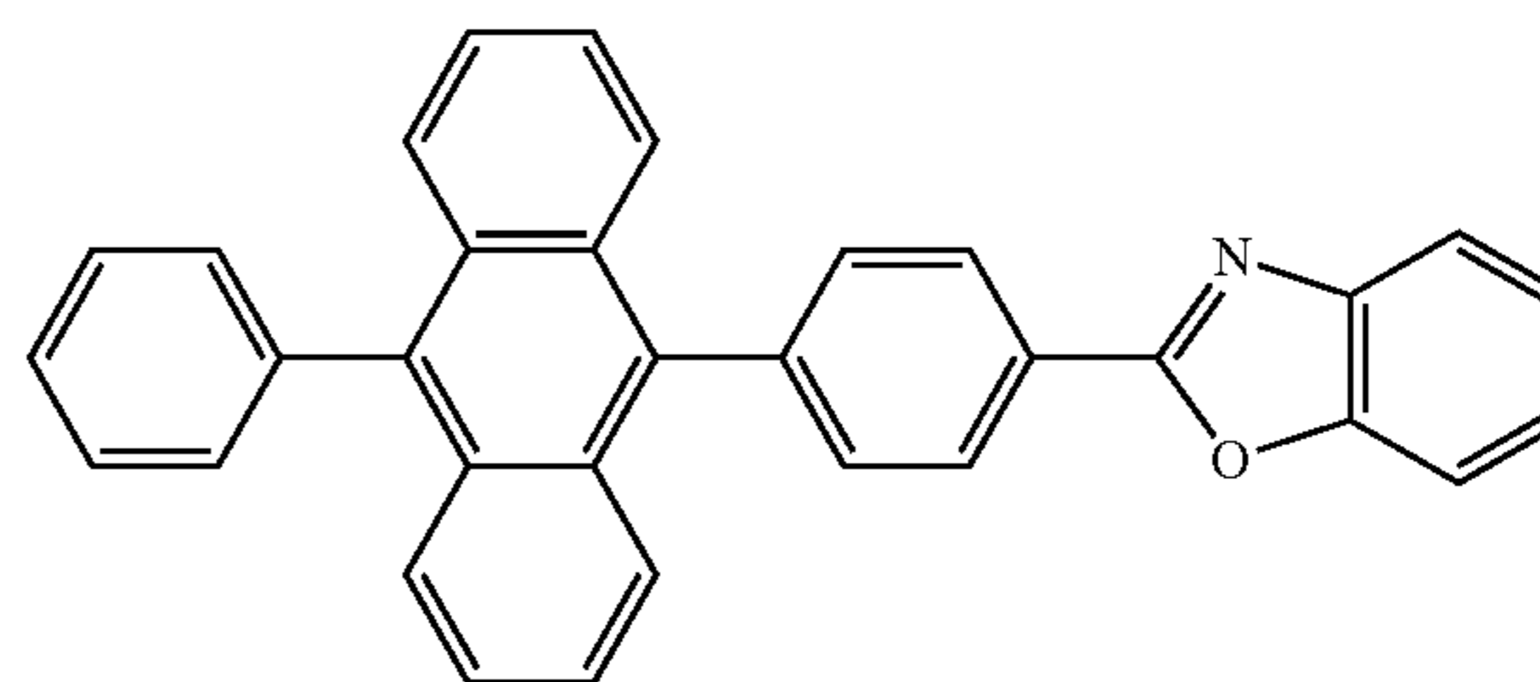
PABOx
