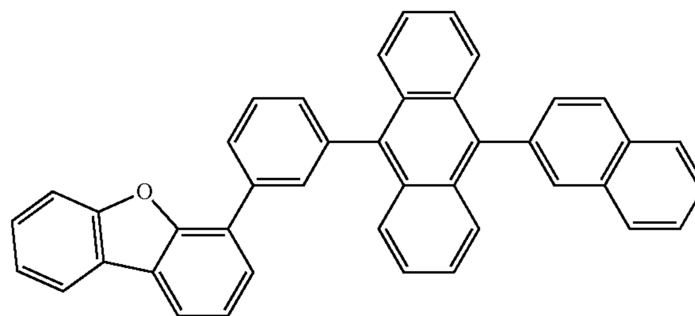
(BH-2)
