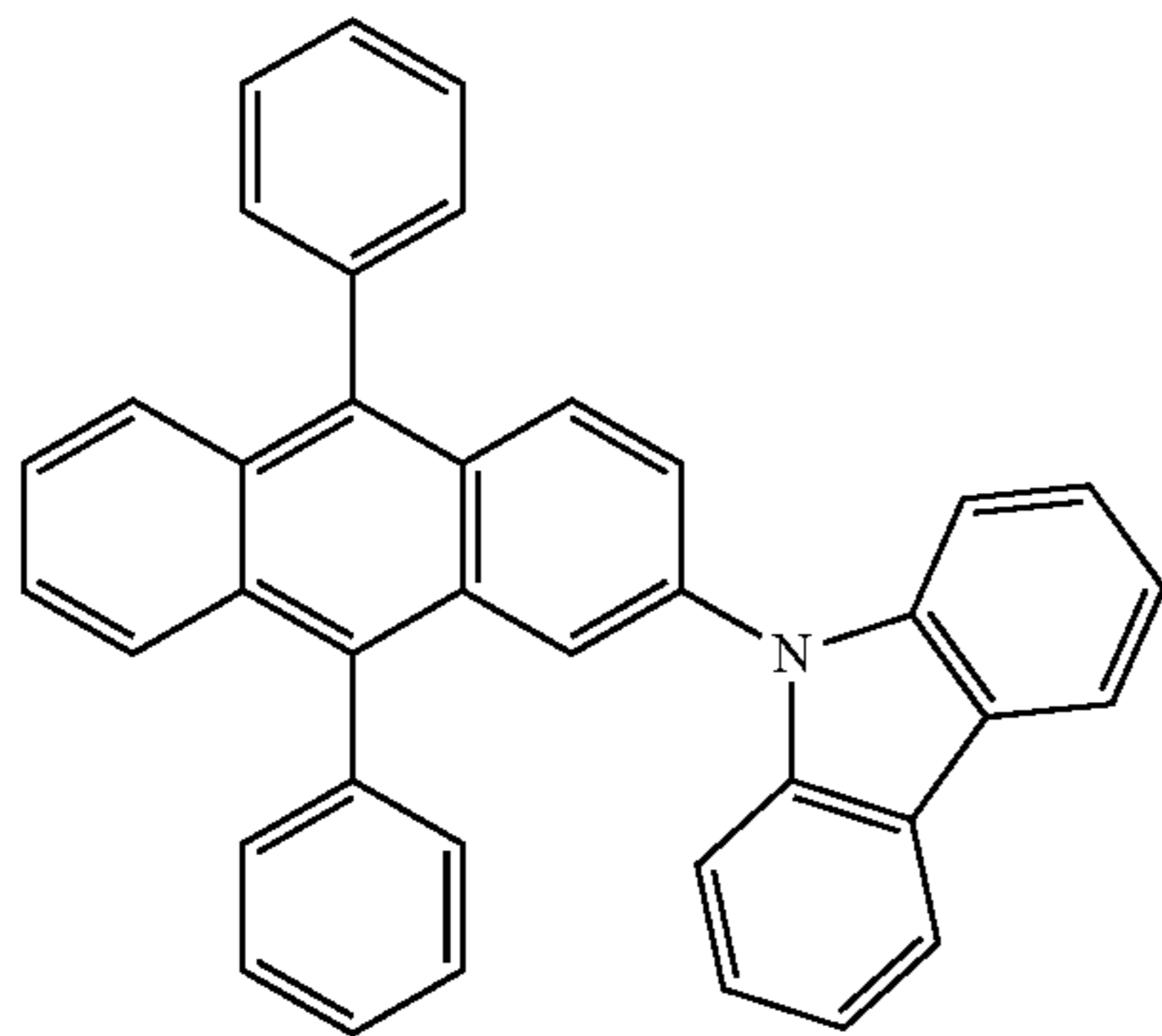
(2CzPA)
