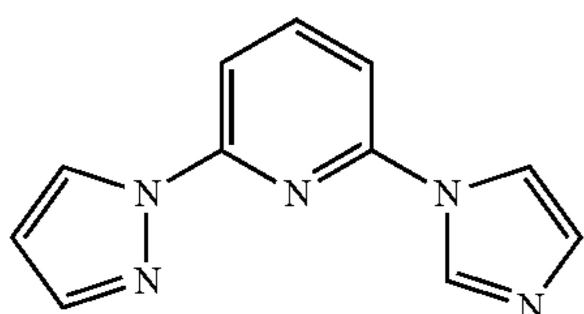
DIz-Py
