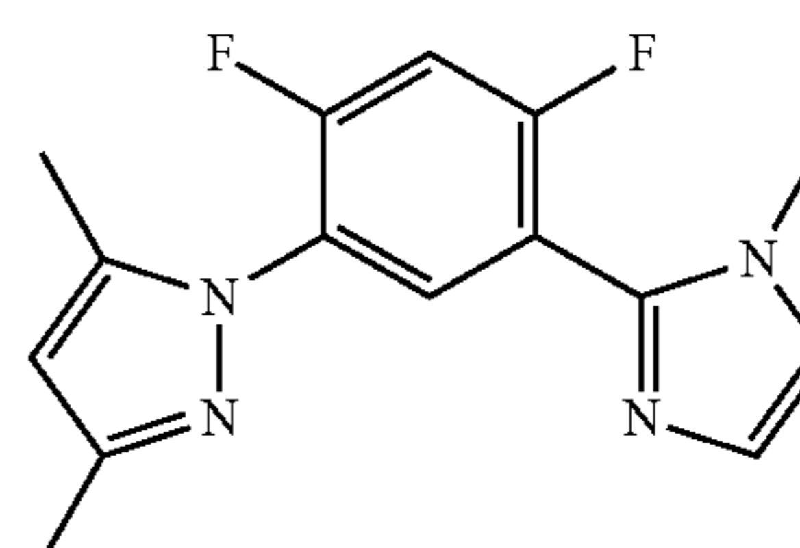
DMPz-DFPh-MIz
