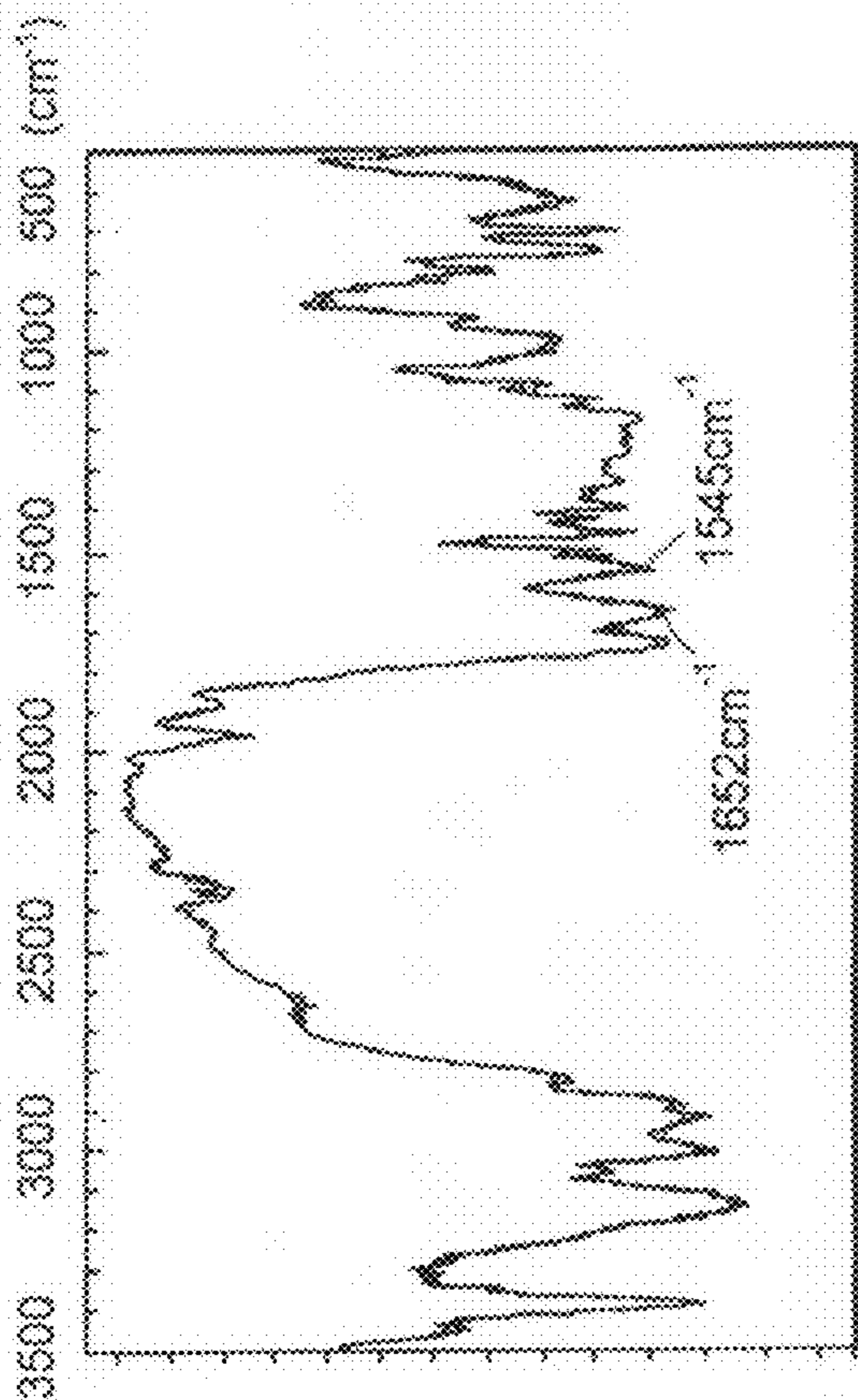
FT-IR Spectrum
