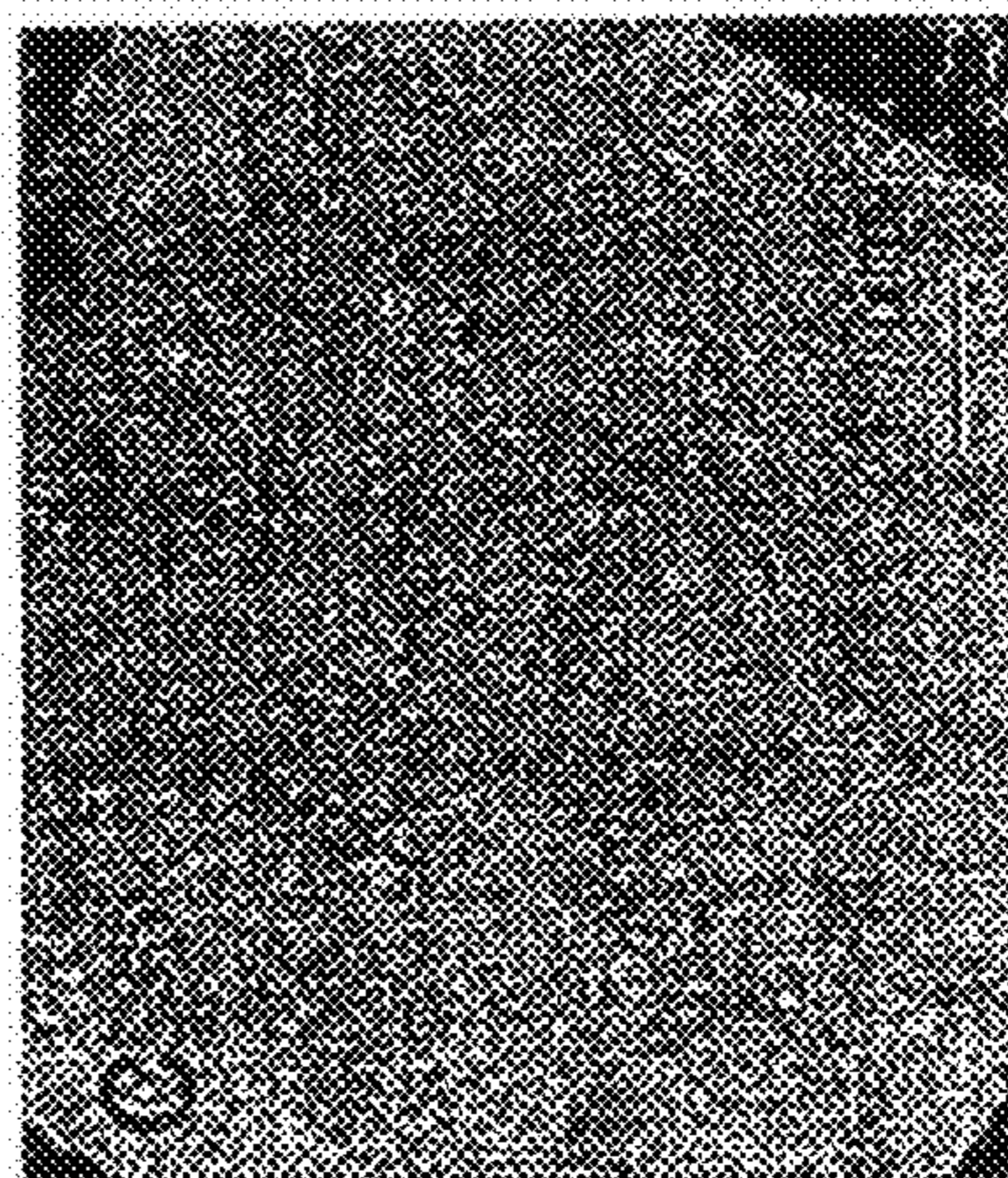
TEM
