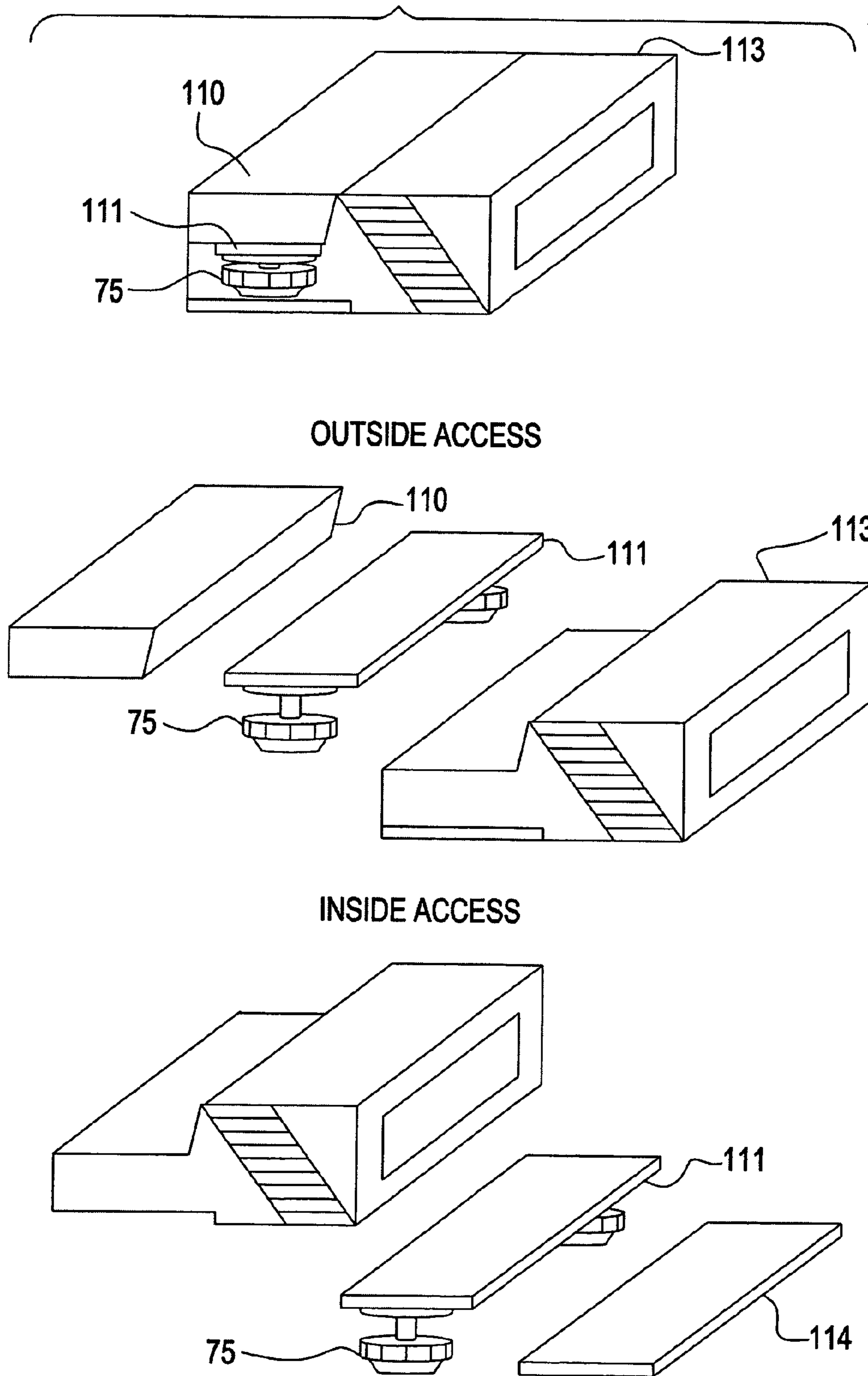
FIG. 35 EVAPORATOR FAN ACCESS
