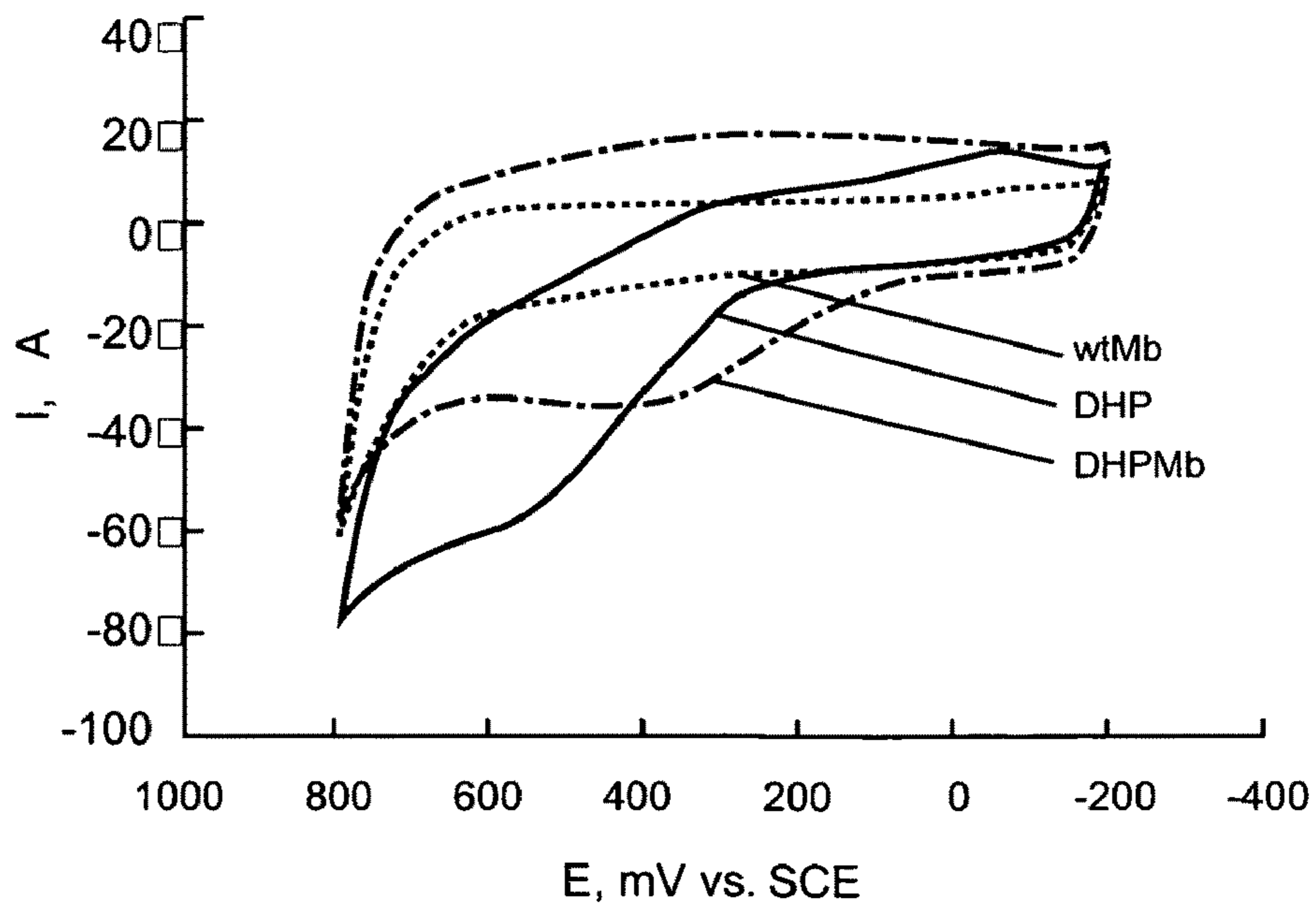
Fig. 3B
