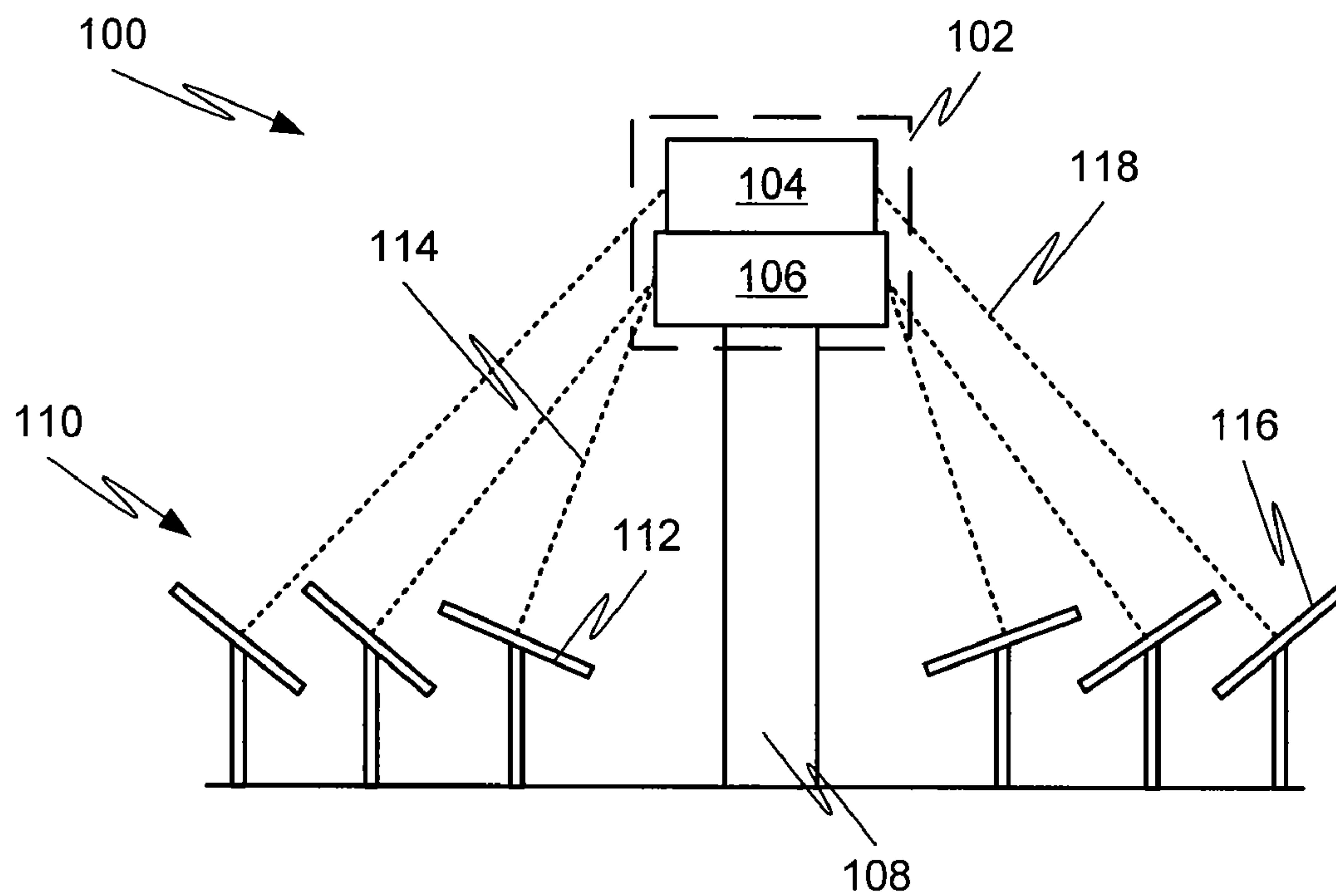
FIG. 1A
