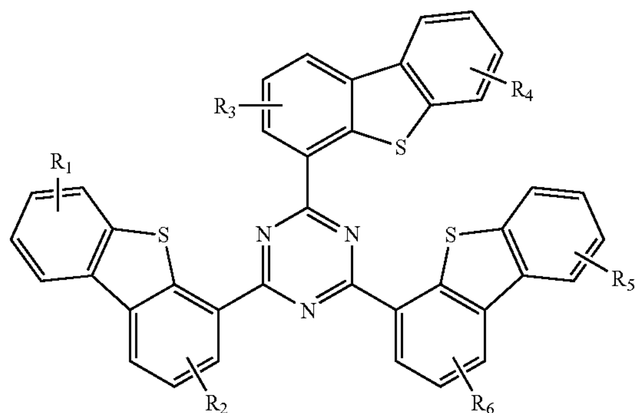
Compound 6G
