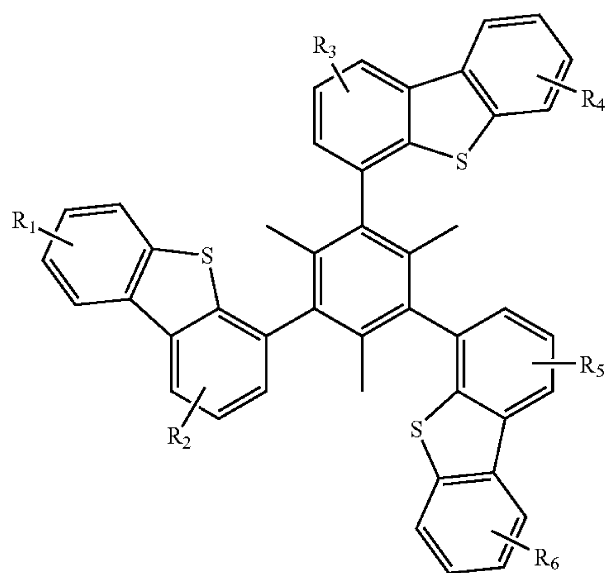
Compound 6G
