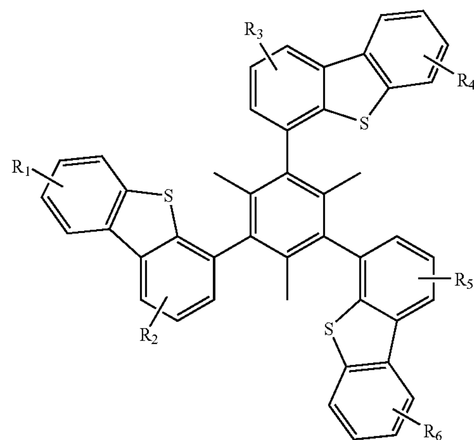
Compound 6G
