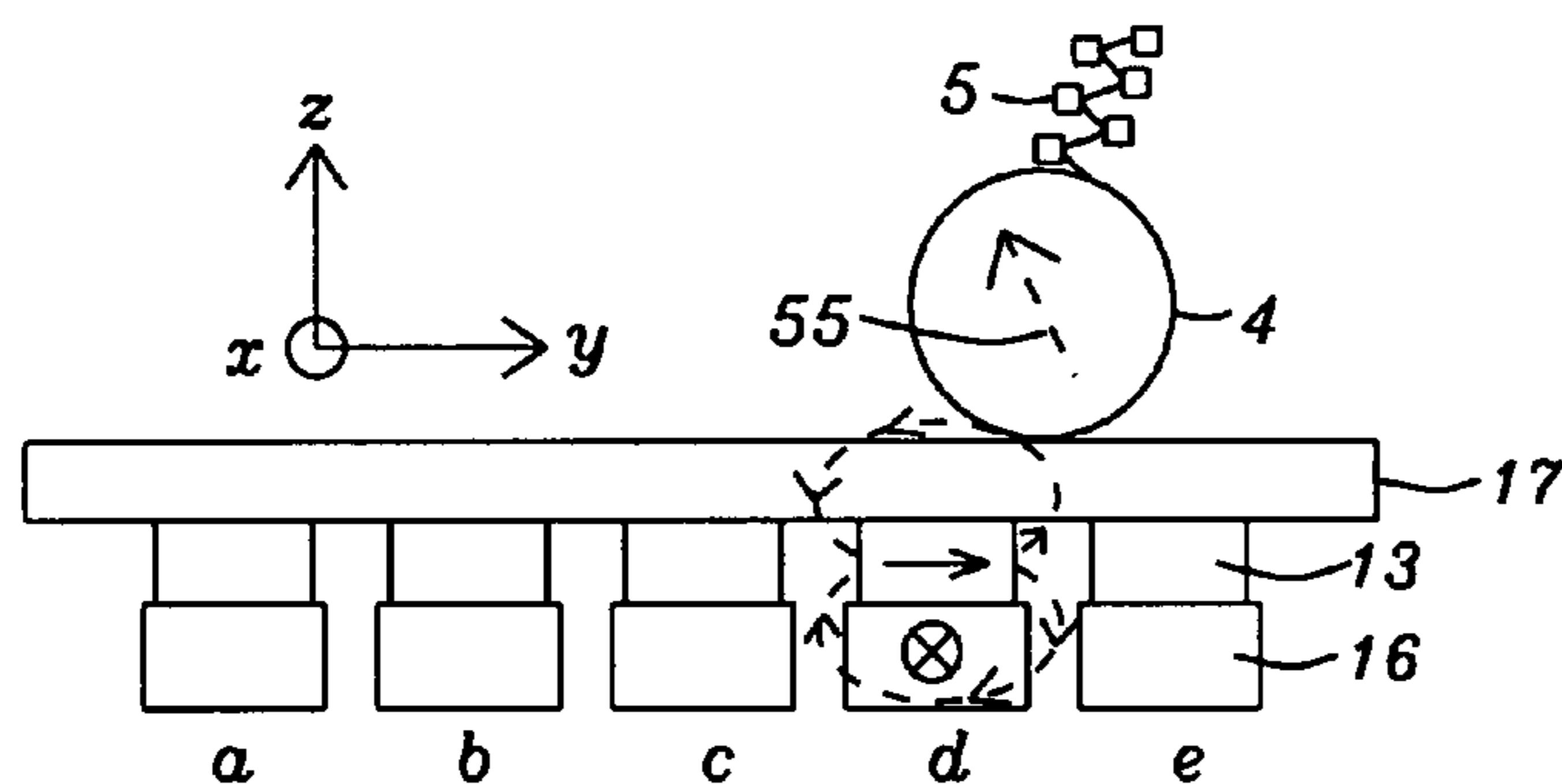
FIG. 6A
