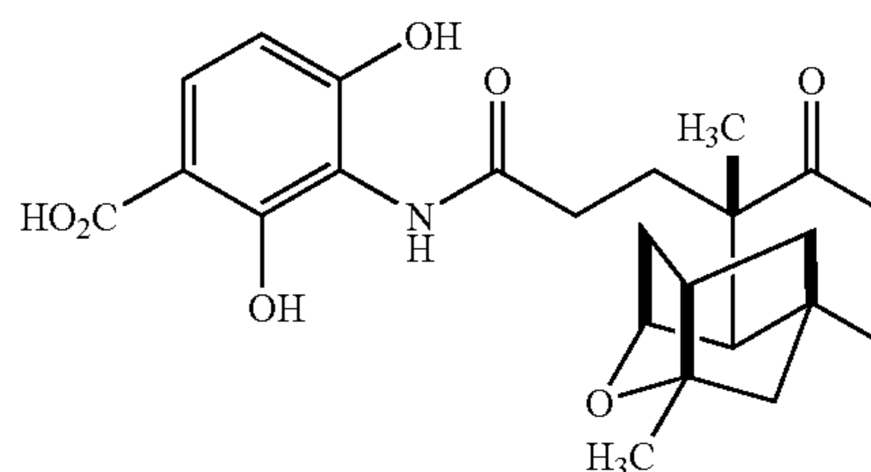
Platensimycin (PTM)
