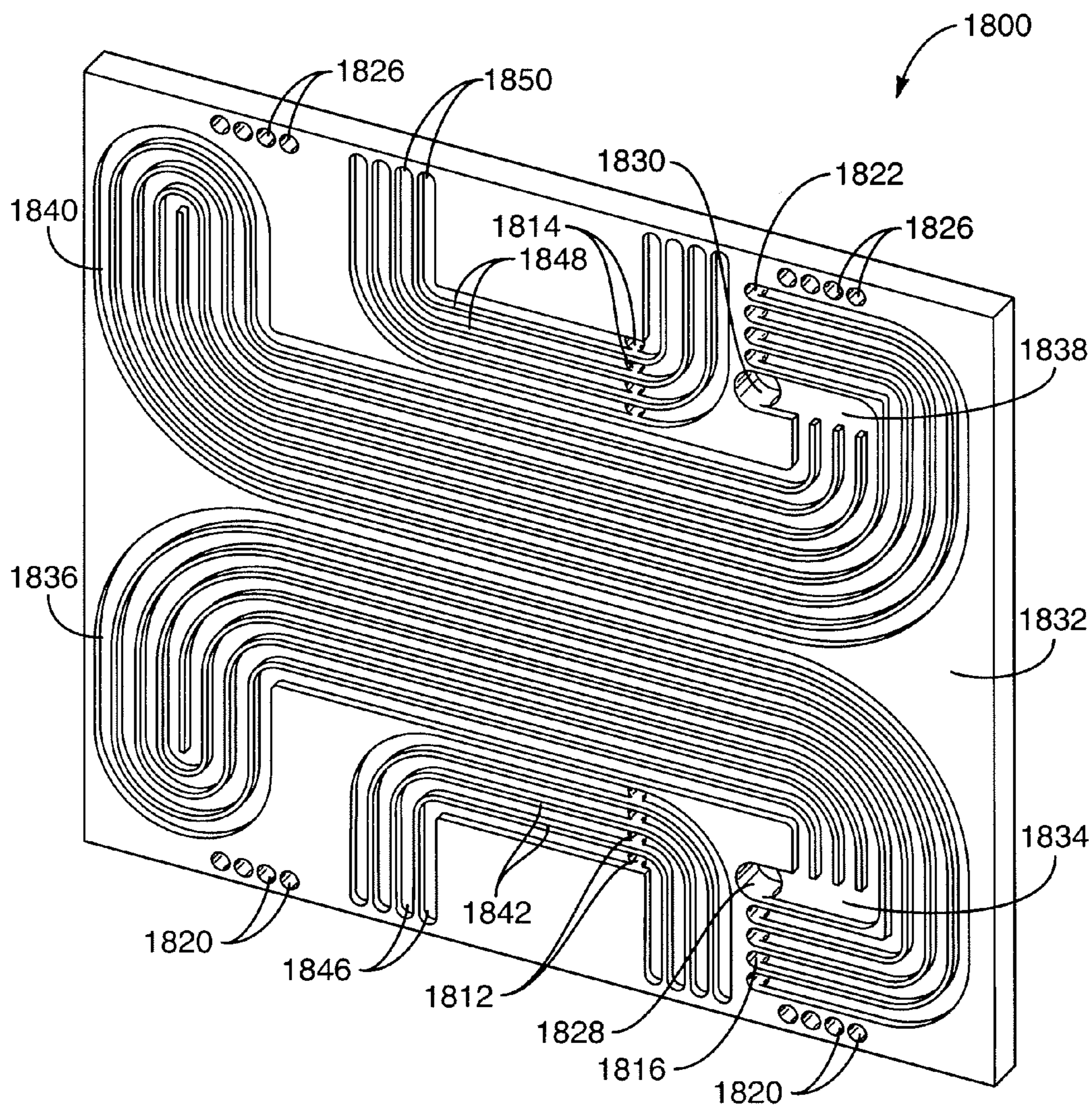
FIG. 19
