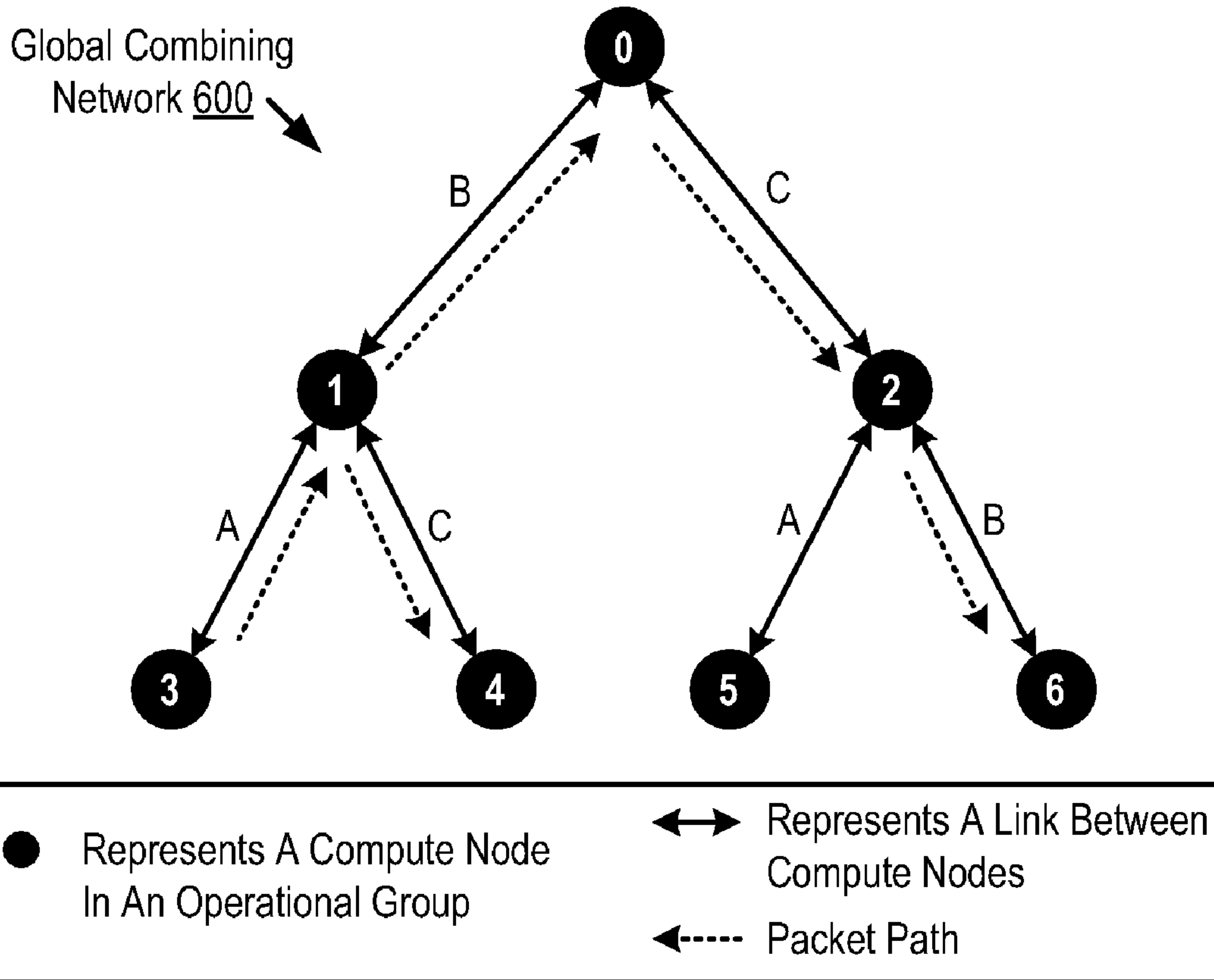
FIG. 8A
