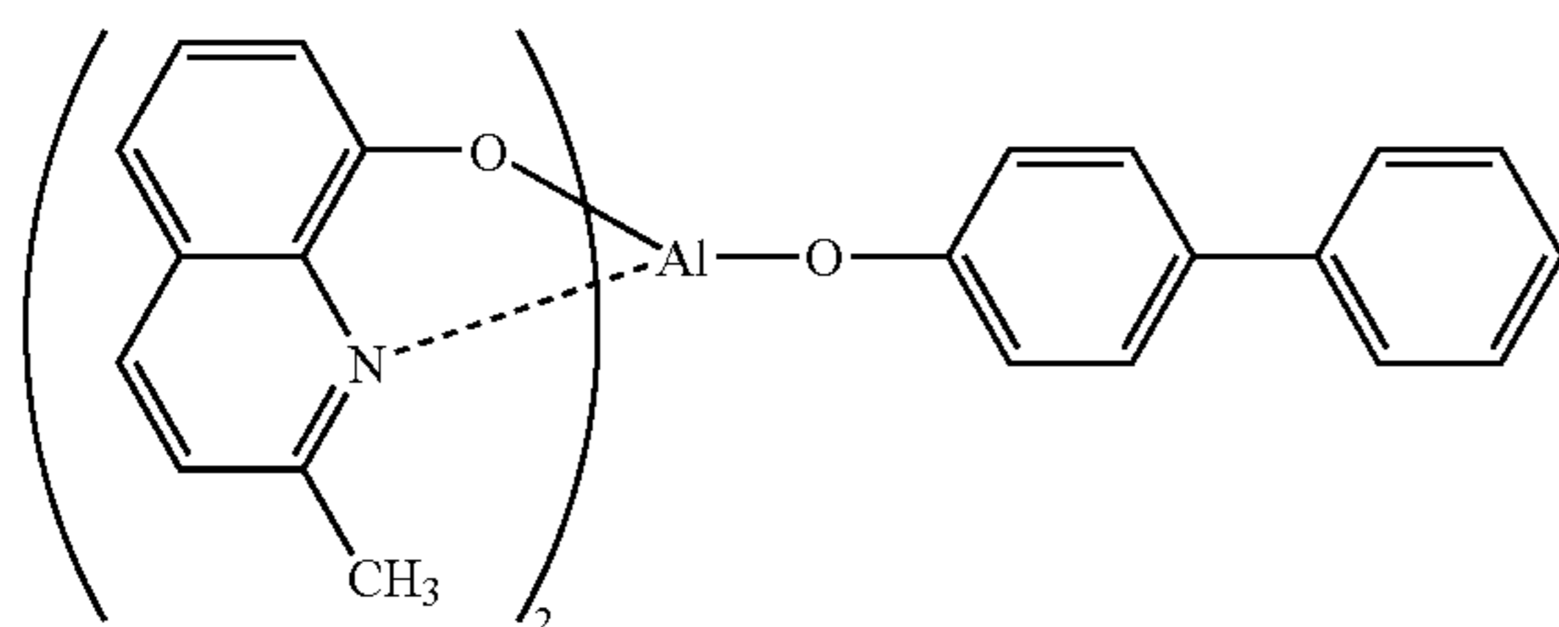
BAlq
