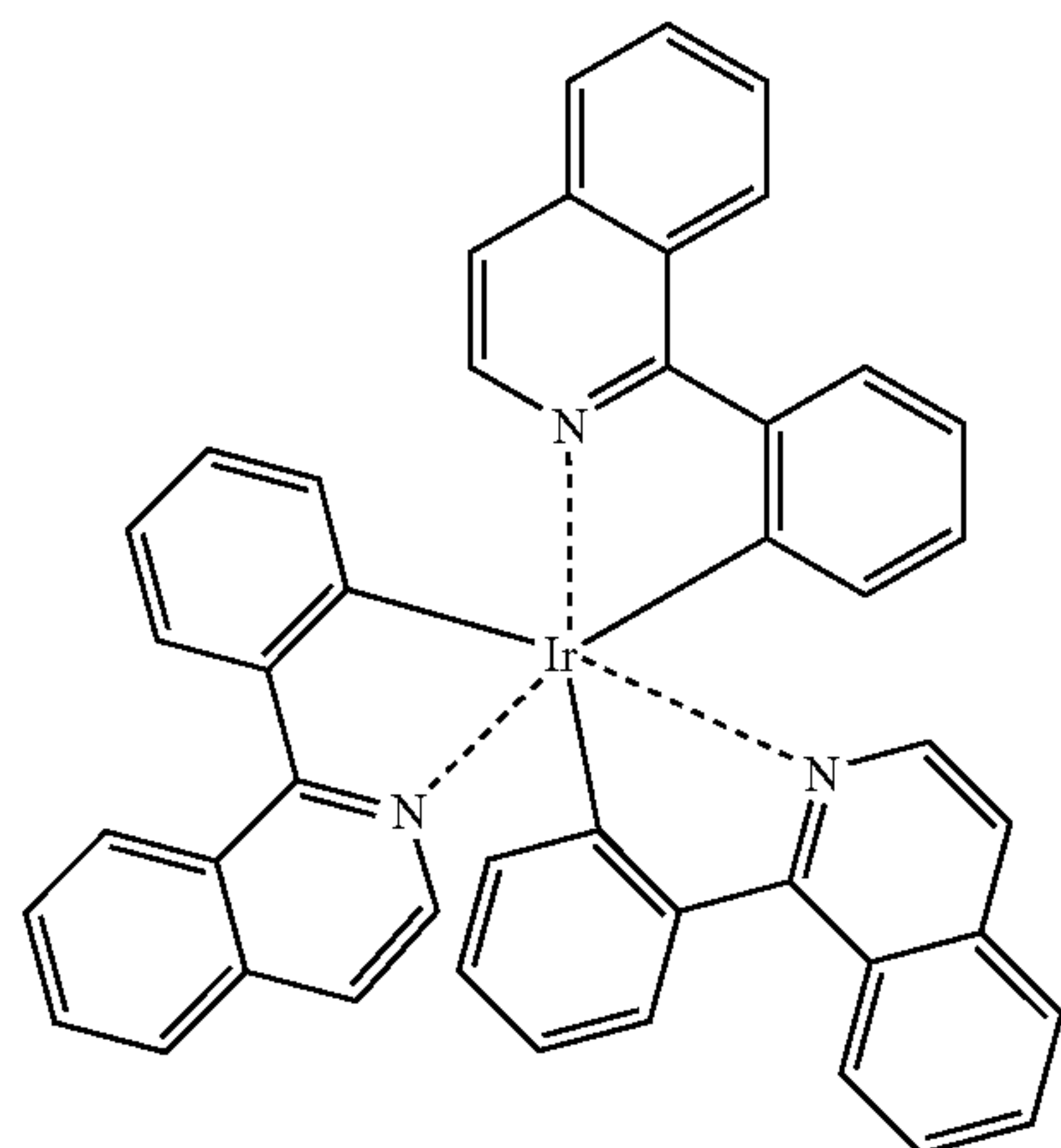
Ir(piq) 3
