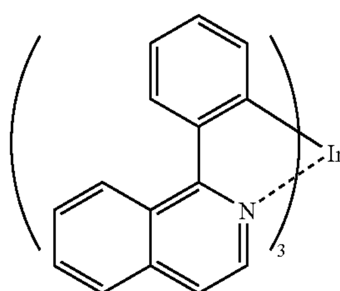
PQIr
