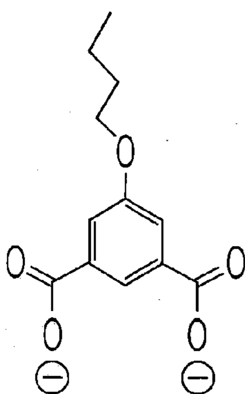
5-butoxy-1,3-benzenedicarboxylate BOBDC
