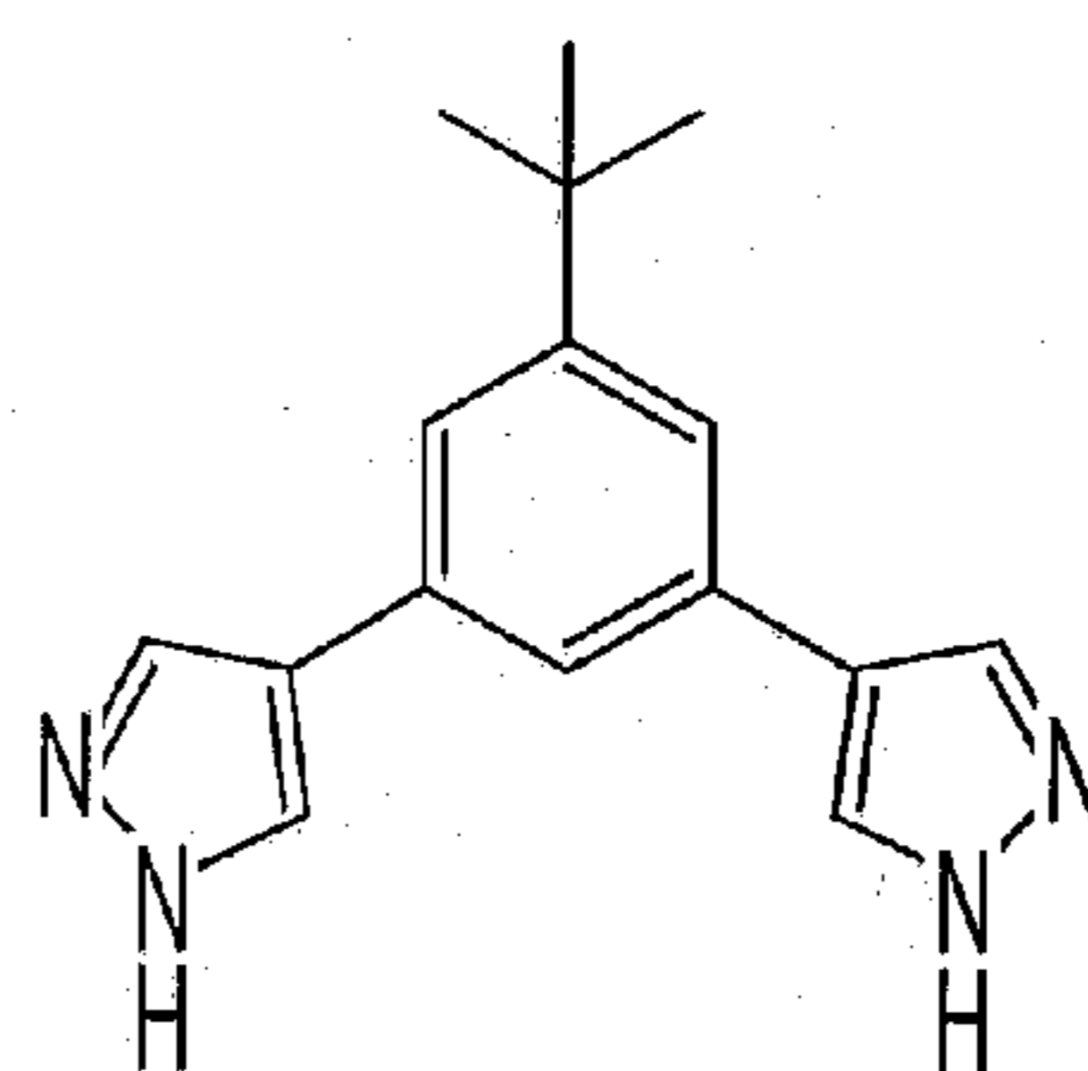
5-tert-butyl-1,3-benzenedi(3'H-4'pyrizable) 4'-BBDPz
