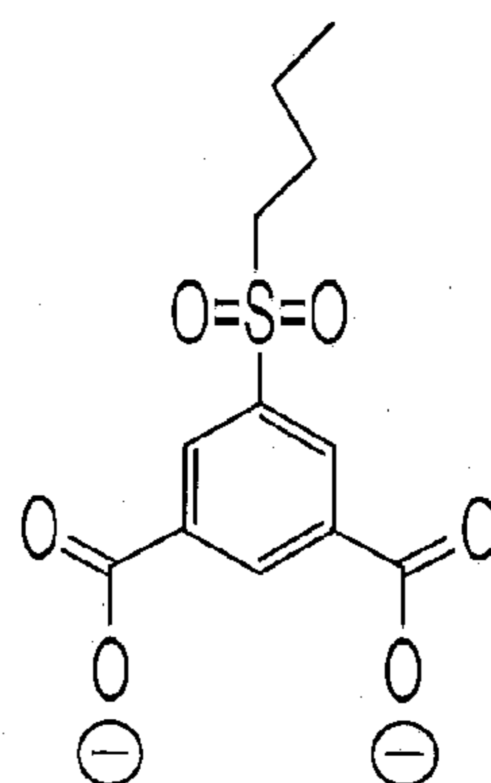
5-butylsulfonyl-1,3-benzenedicarboxylate BSBDC
