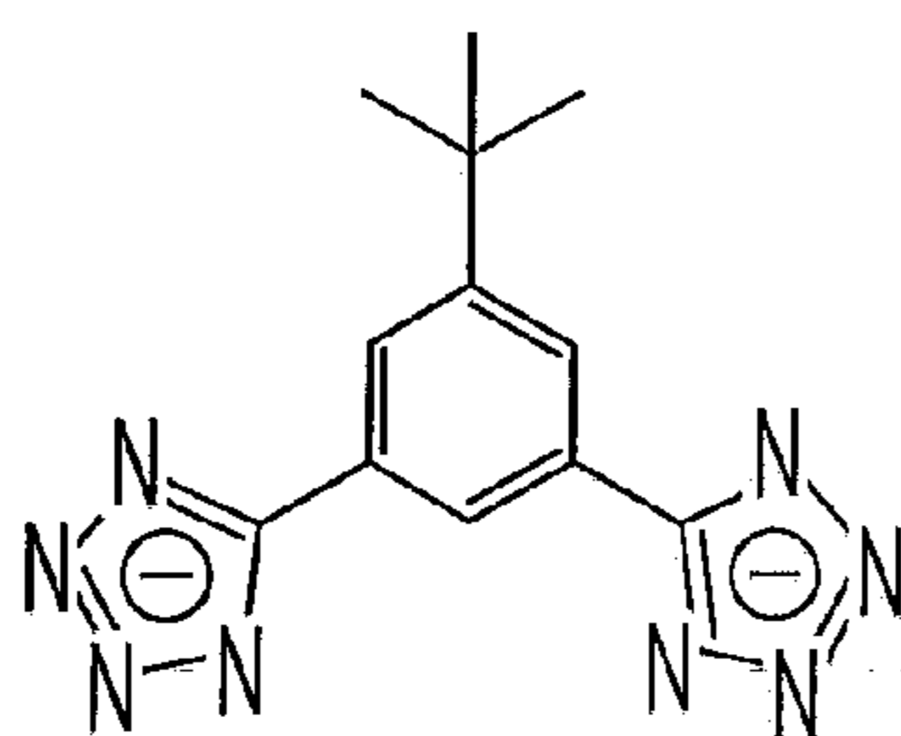
5-tert-butyl-5,5-benzeneditetrazolate BBDT
