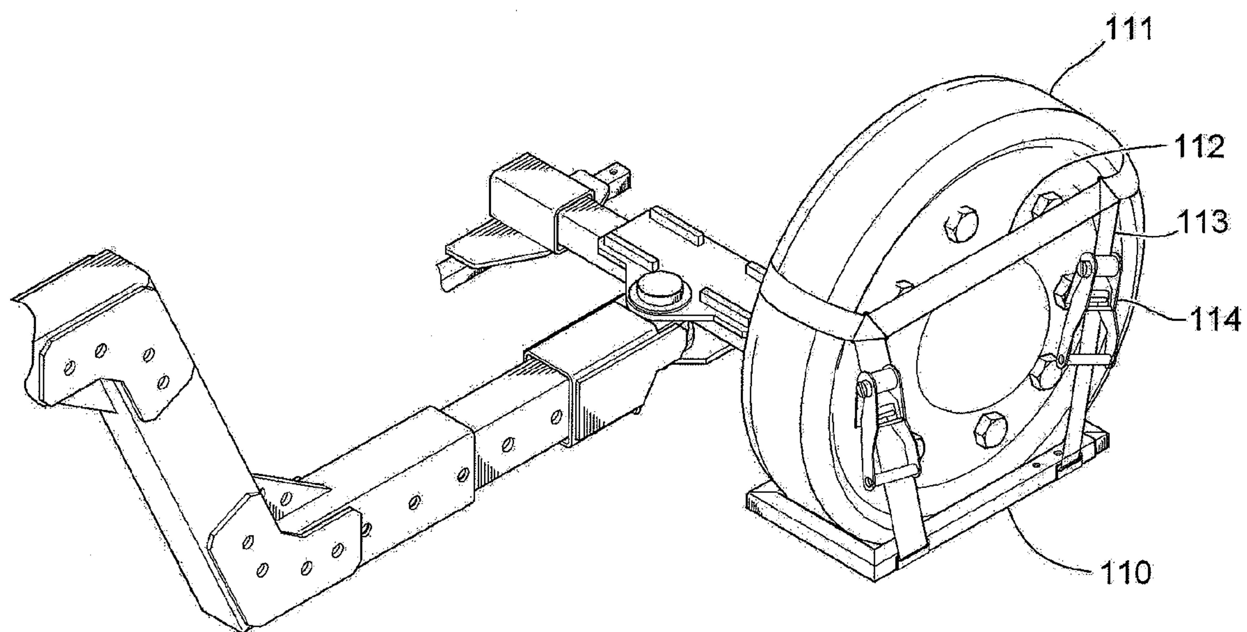
FIG. 11
