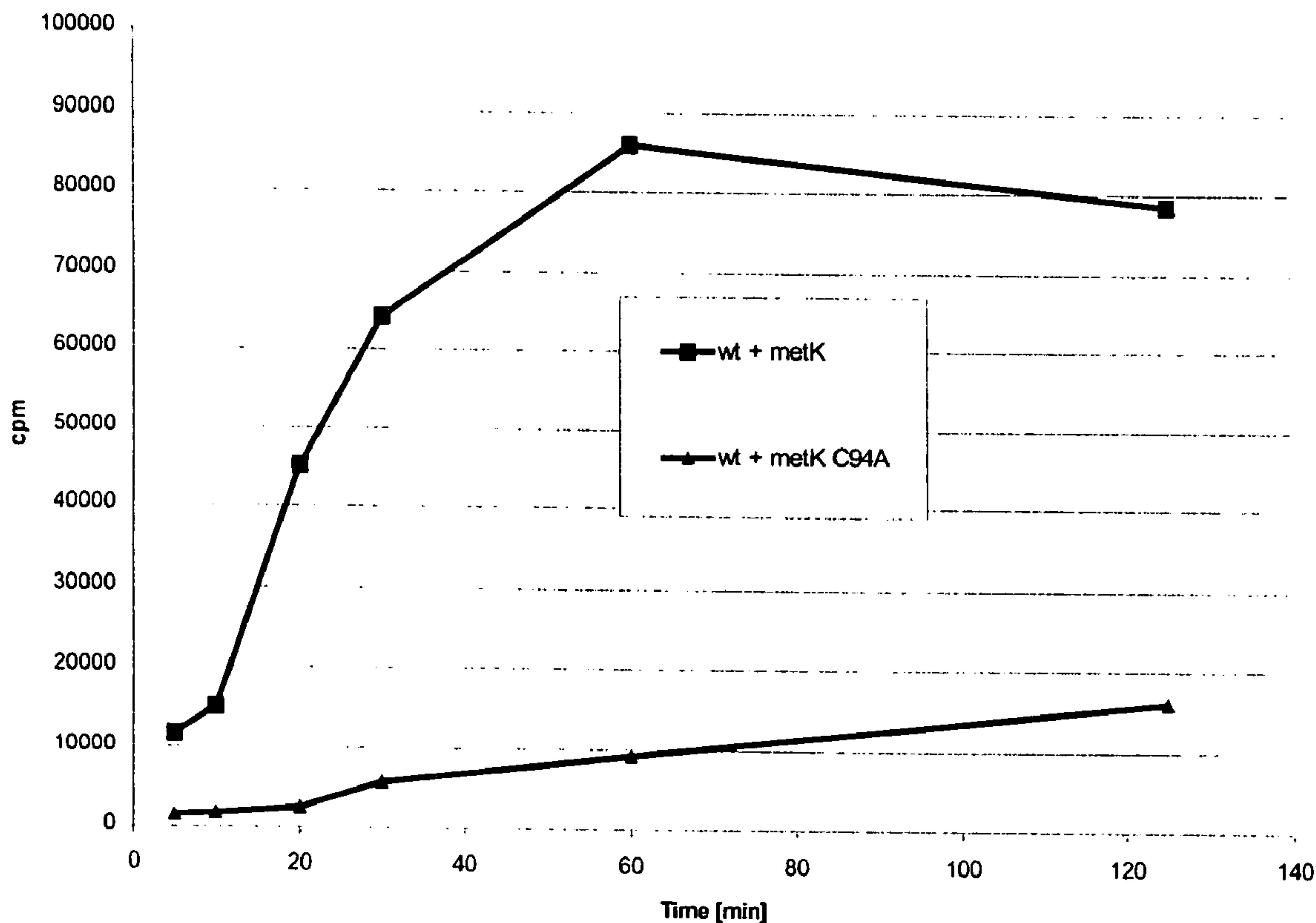
metK-Assay
