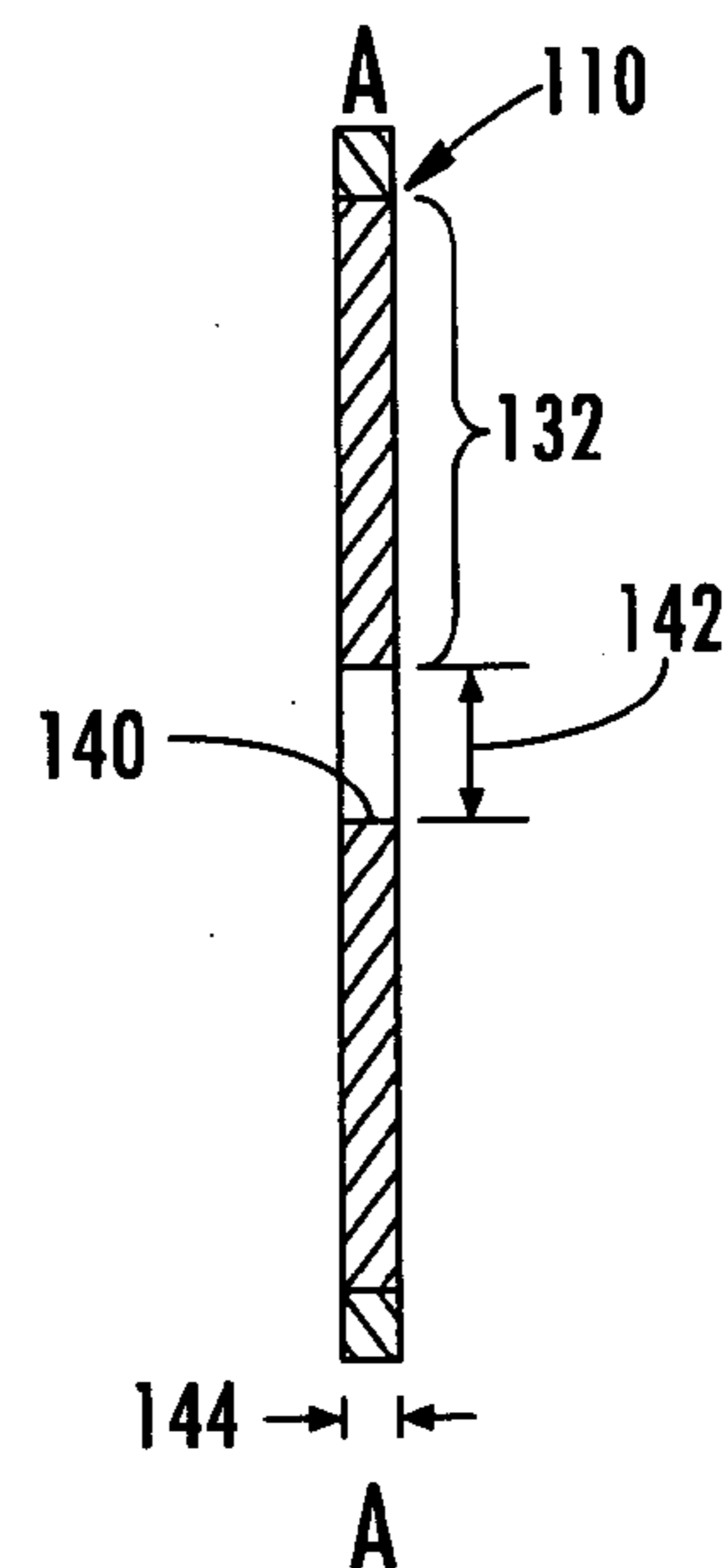
FIG. 5B
