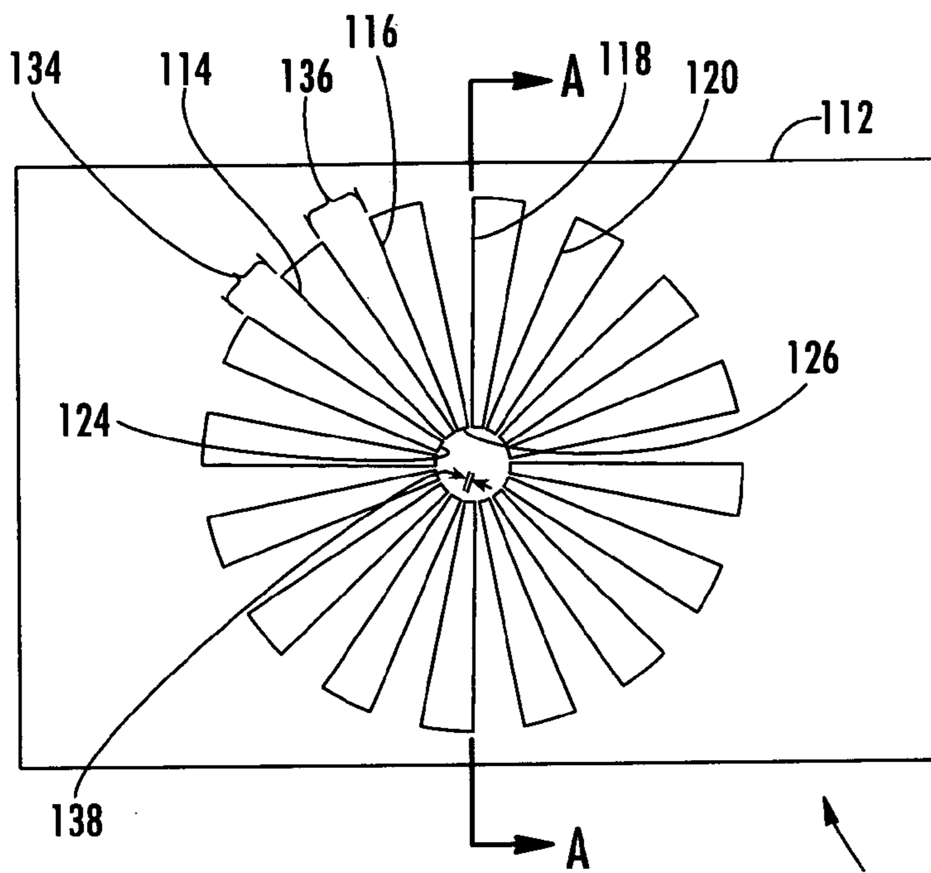
FIG. 5A
