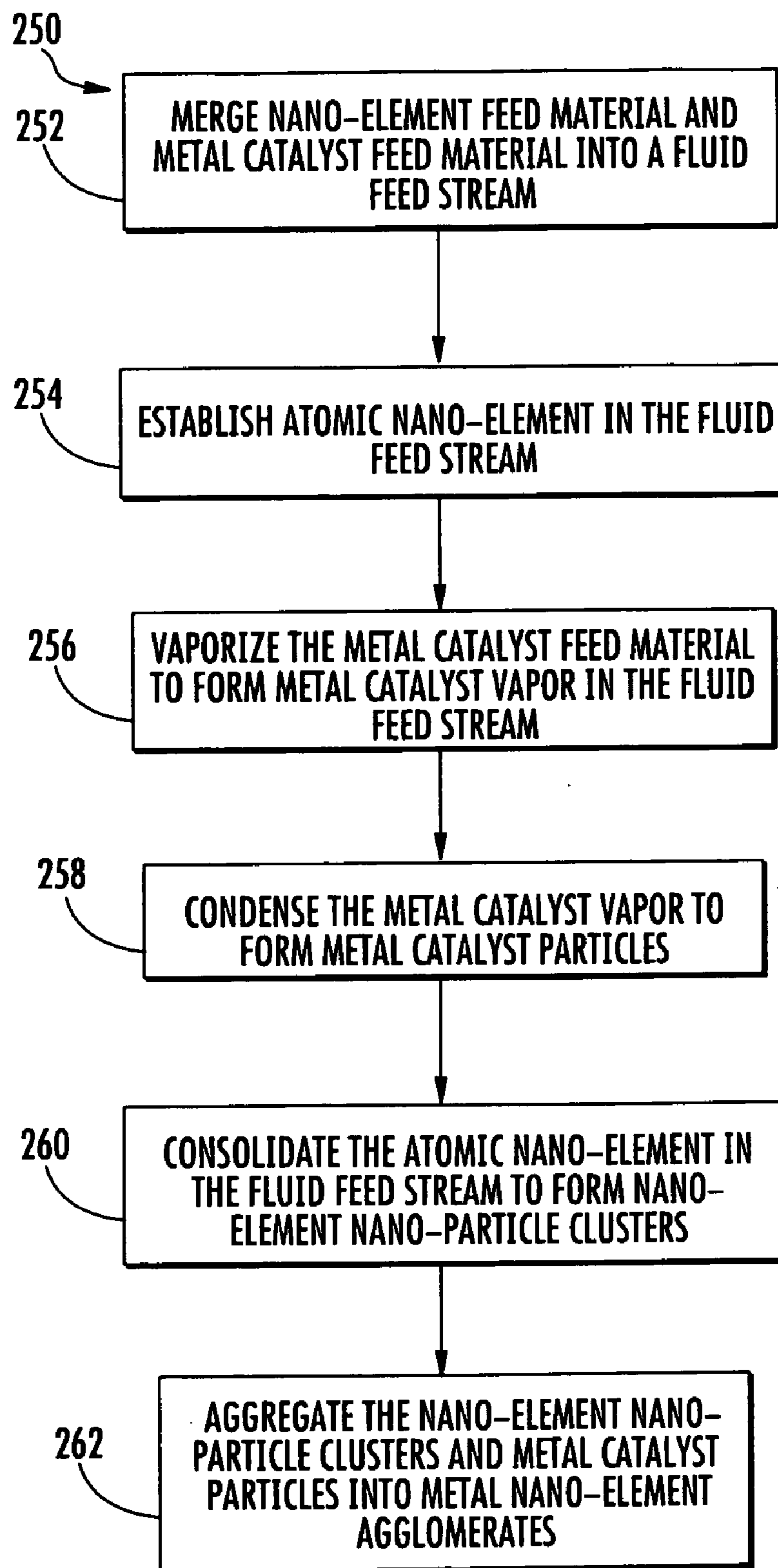
FIG. 9
