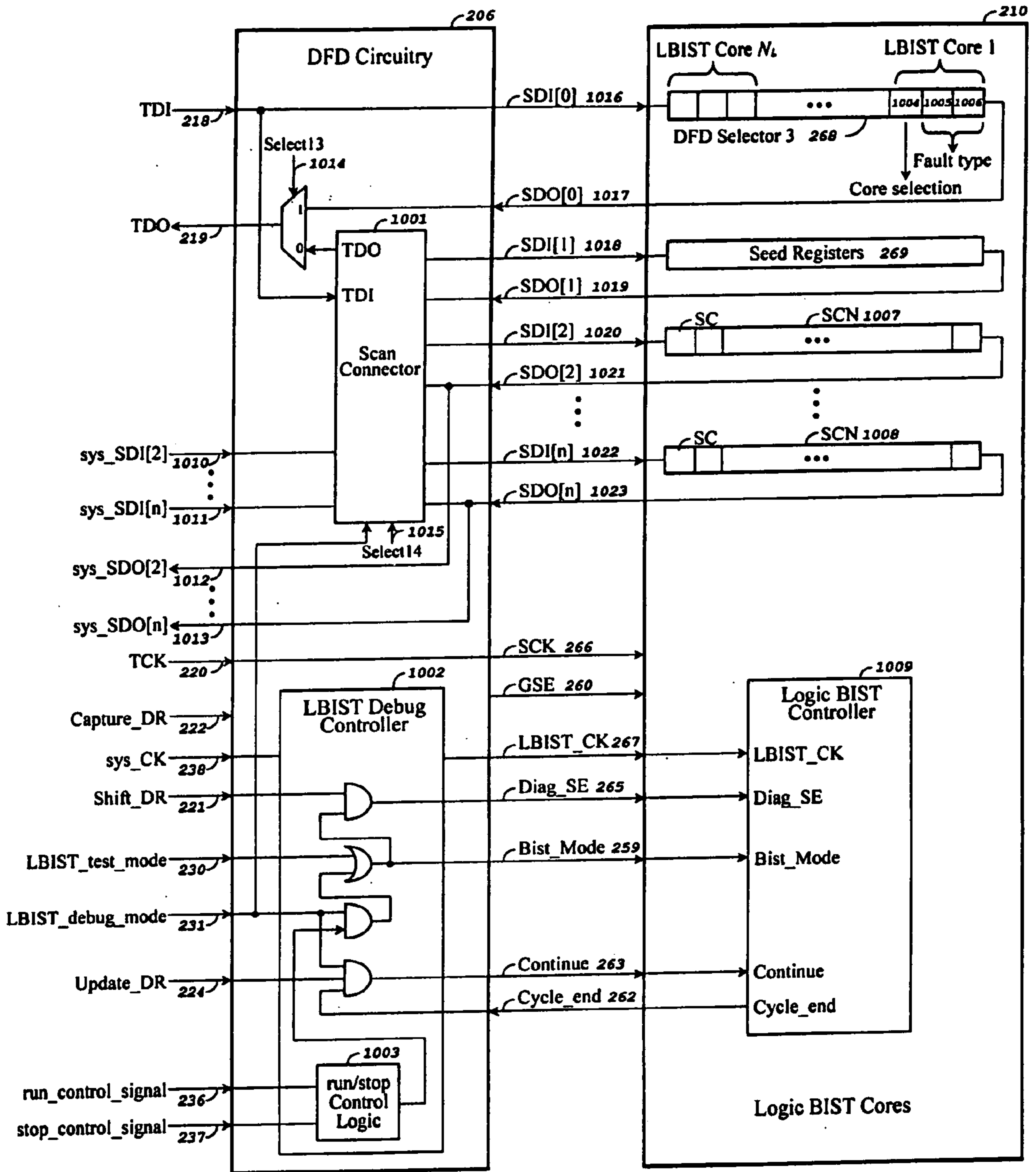
FIG. 10
