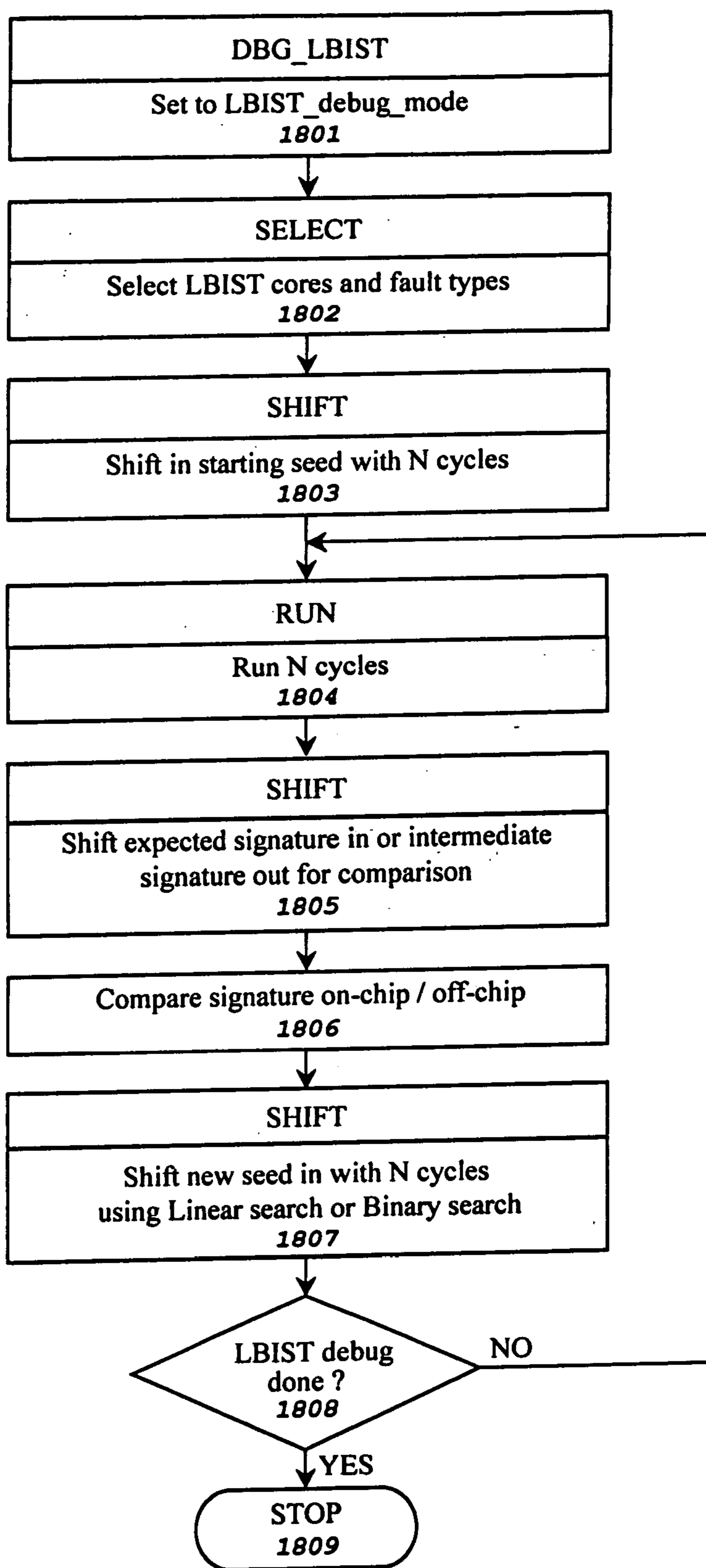
FIG. 18
