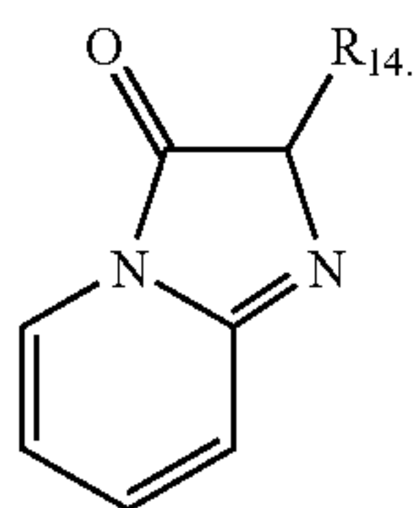
Imidazo[1,2-a]pyridine-3(2H)-ones.
