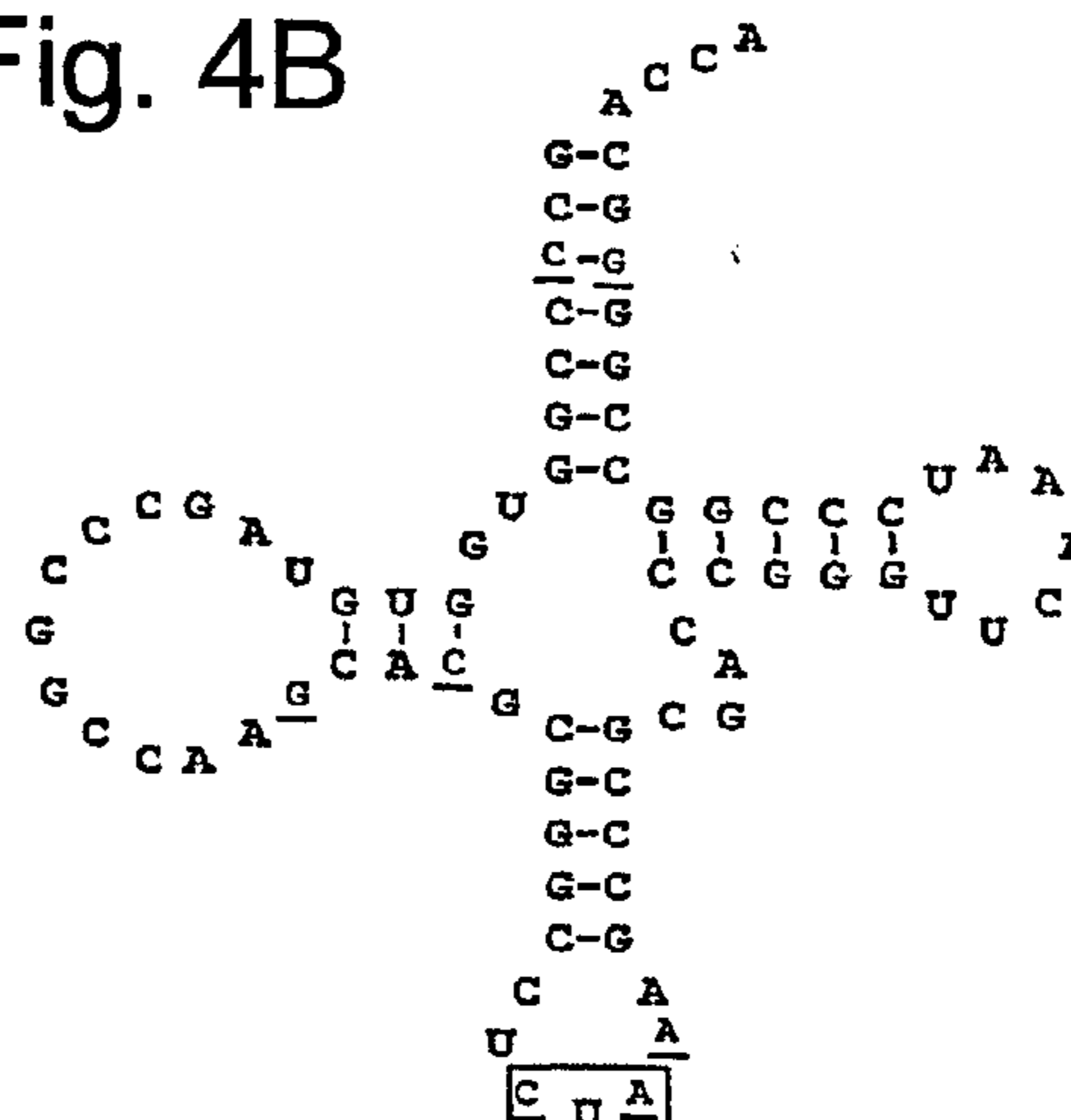
AE(GC) tRNA
