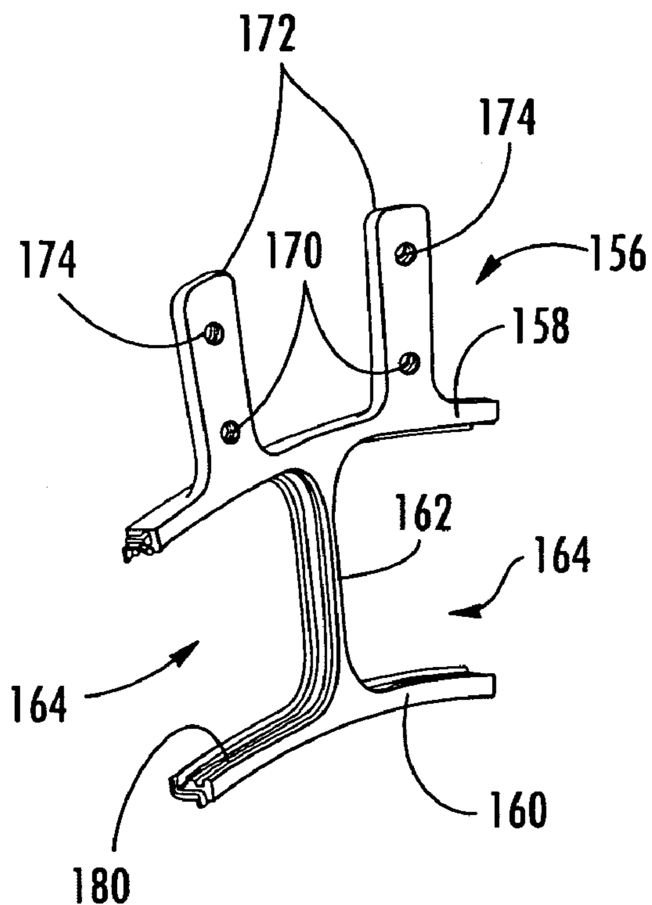
FIG. 10
