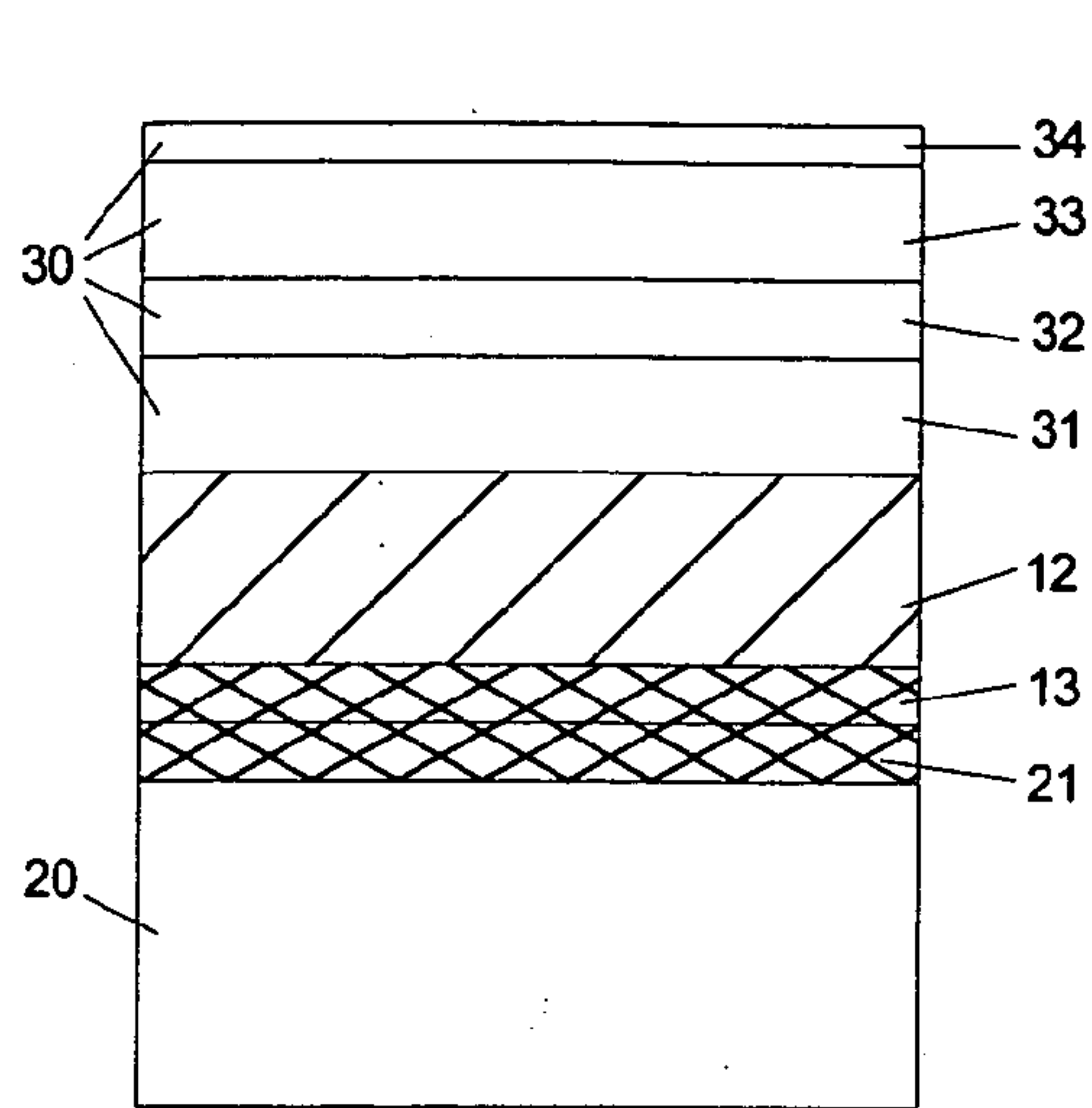
FIG. 2I: MOCVD Epitaxial Growth
