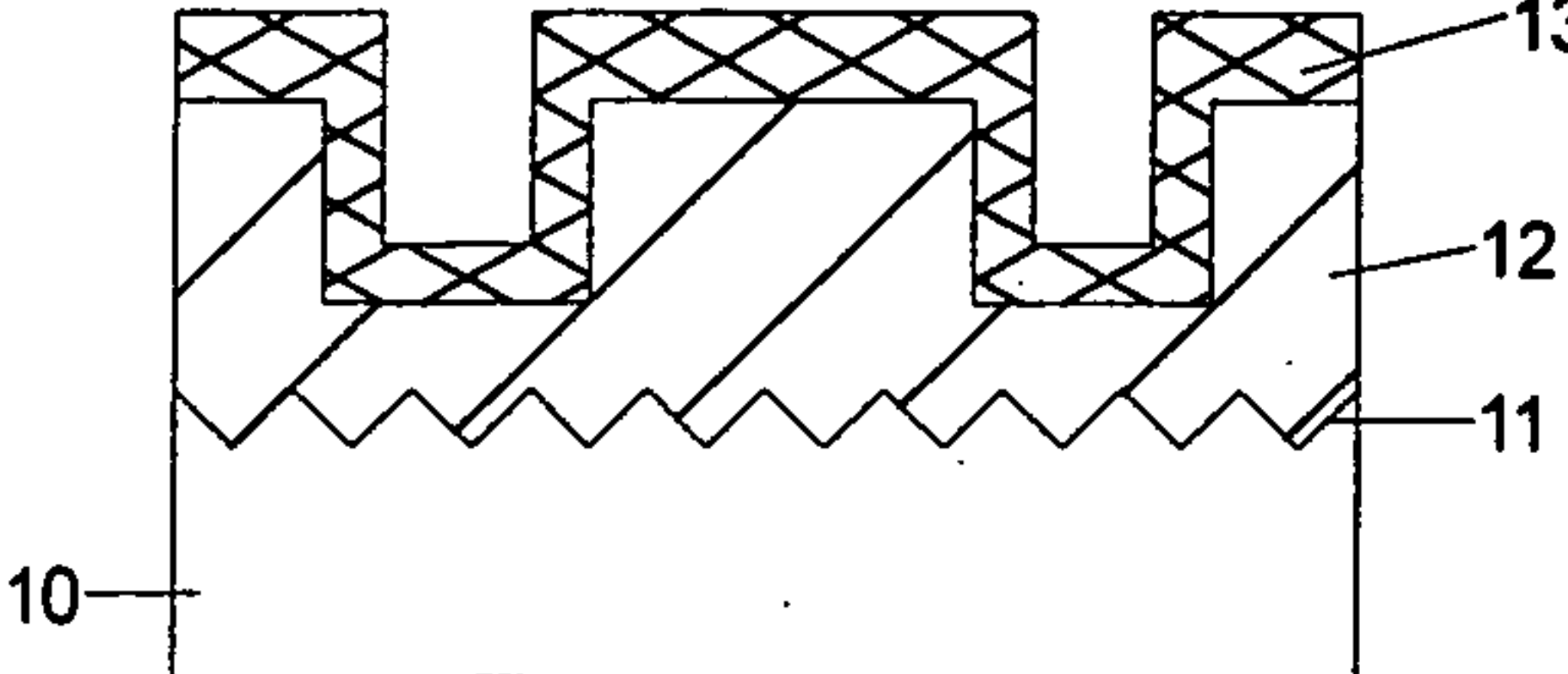
FIG. 3B: SiO2 Deposition
