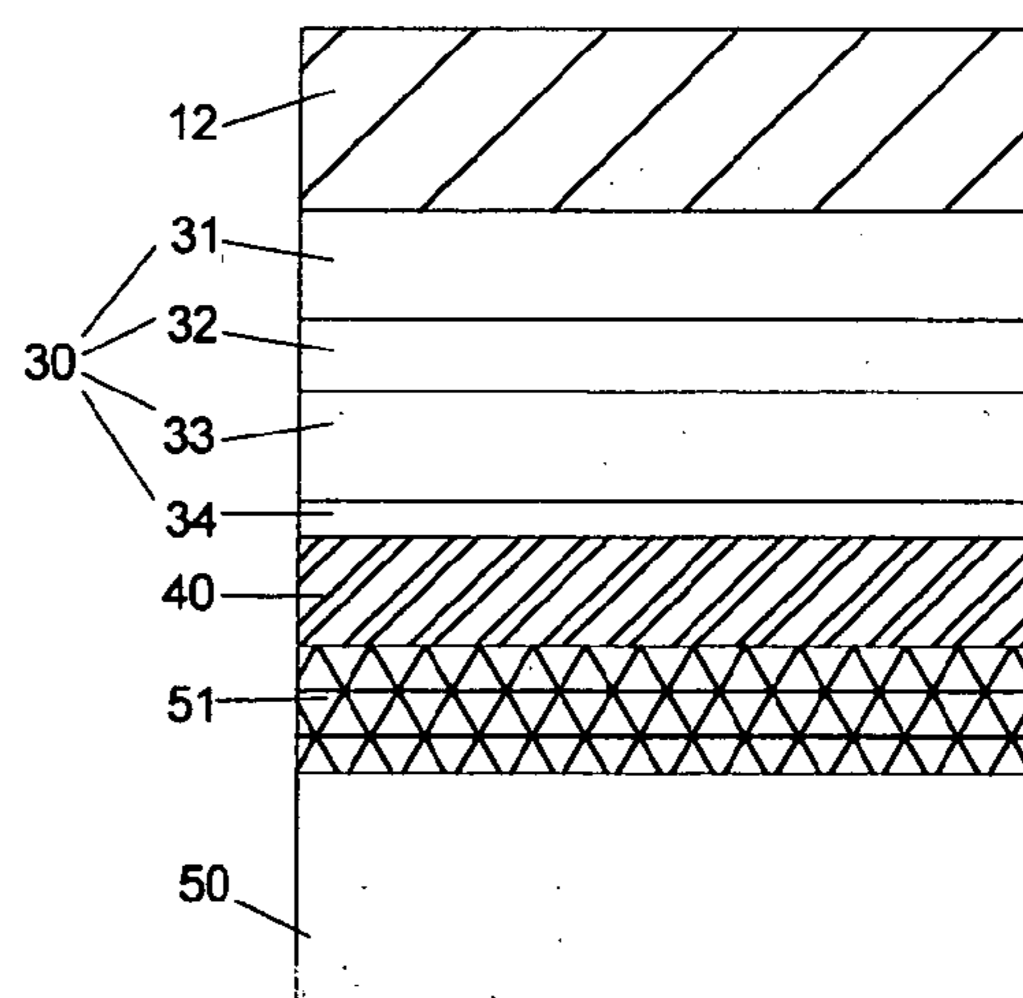
FIG. 2N: Etch
