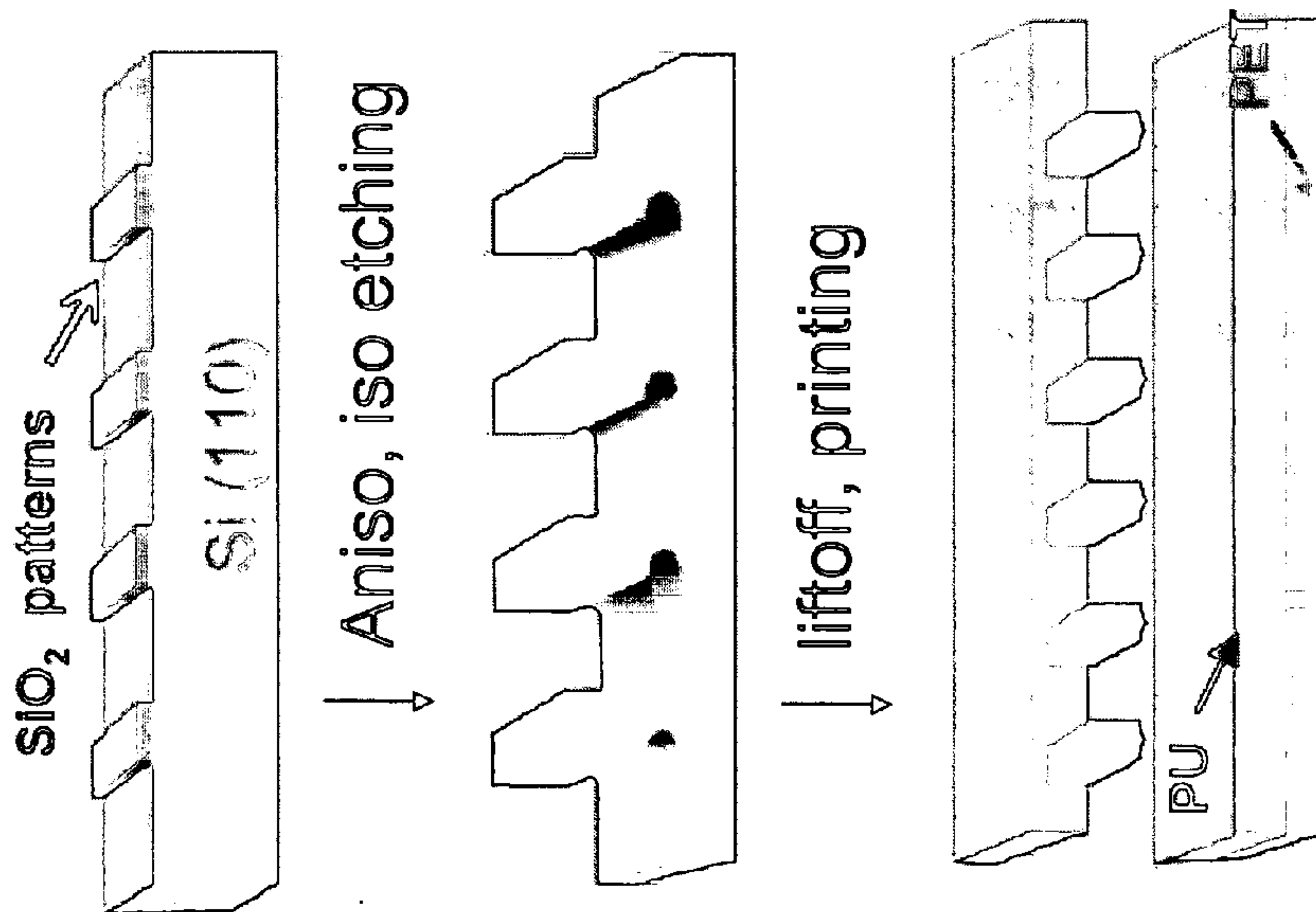
Fig. 18J: Bulk (110) Si to \mu S-Si
