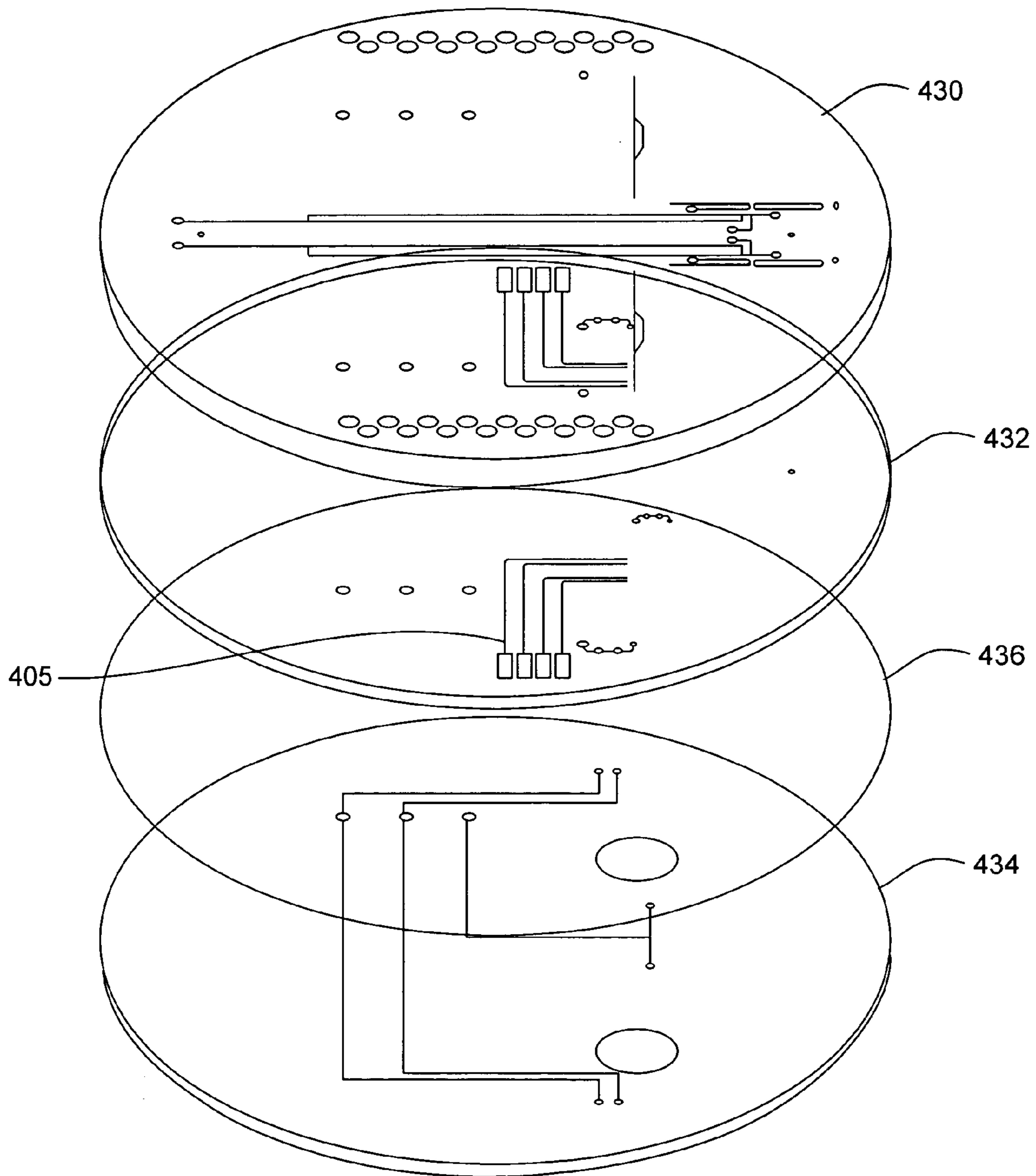
FIG. 4C
