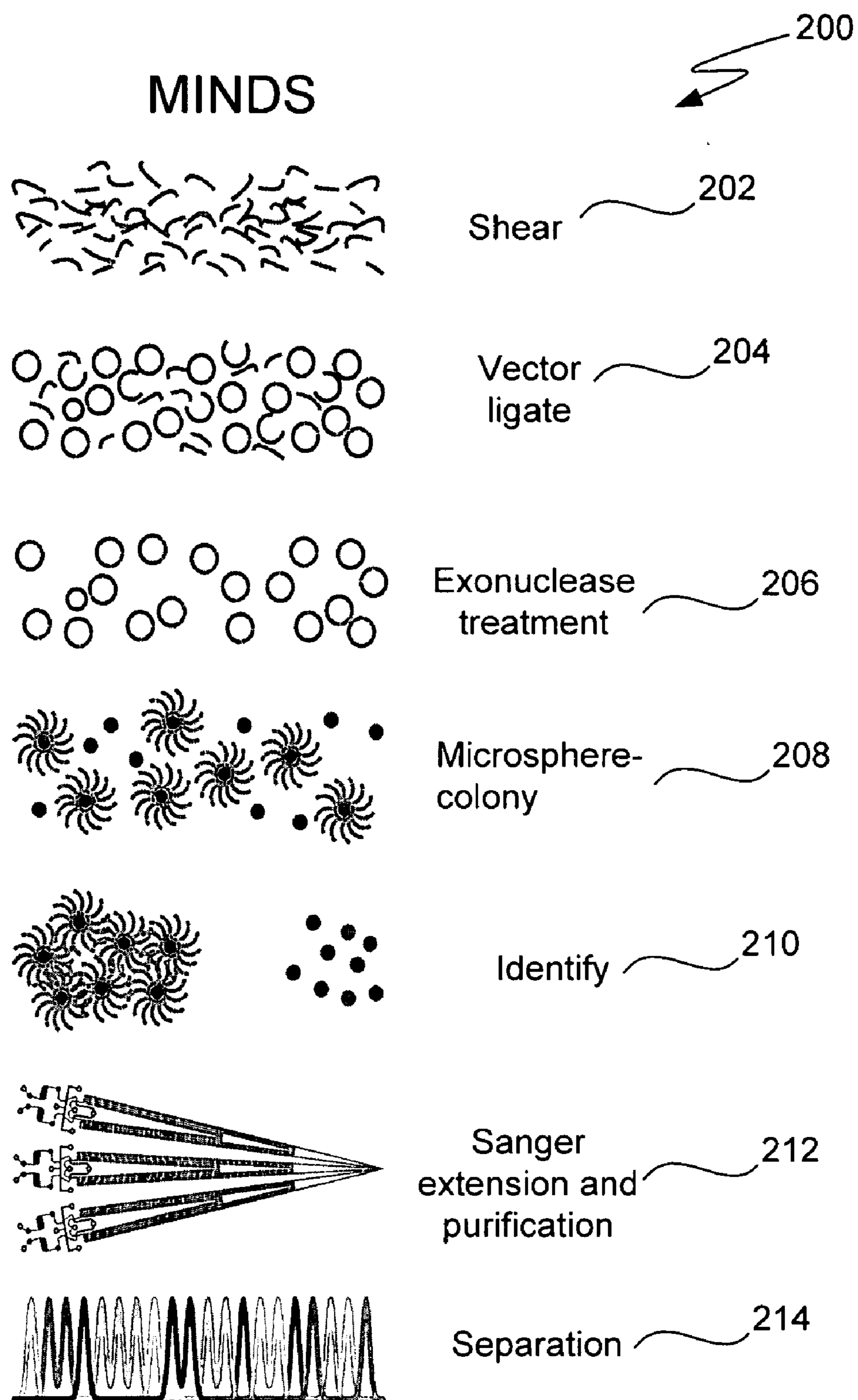
FIG. 2
