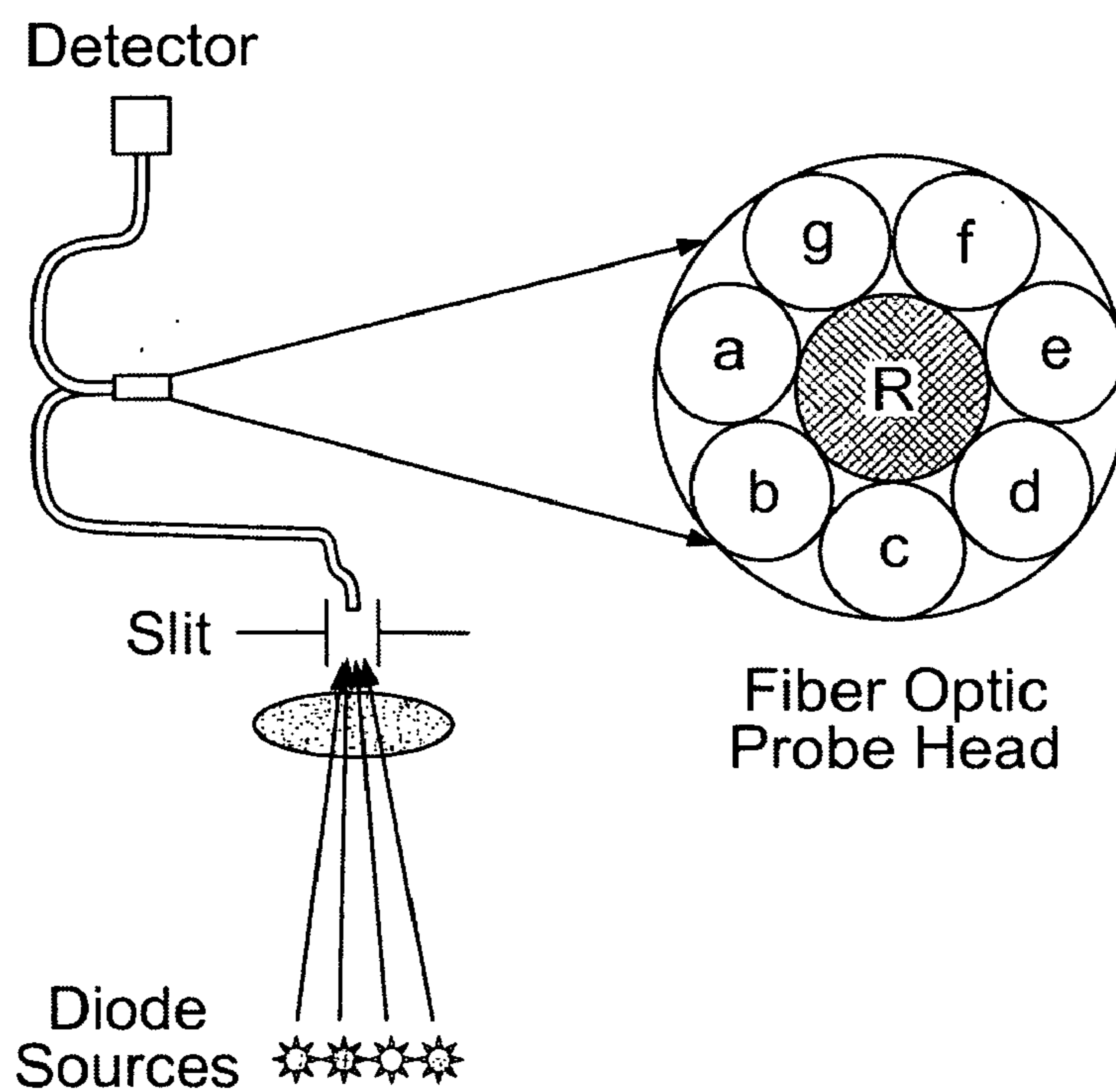
FIG. 33E
