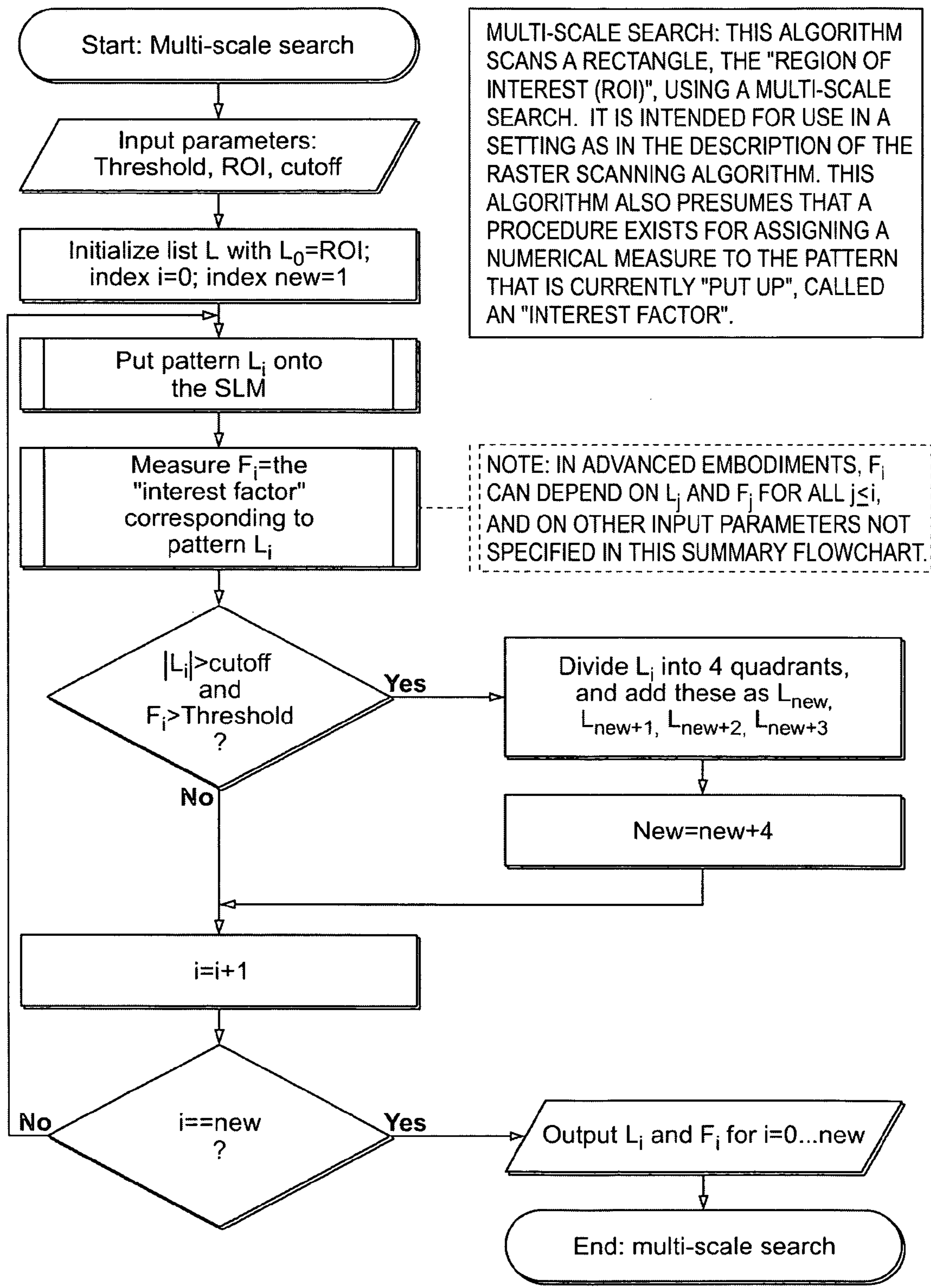
FIG. 26
