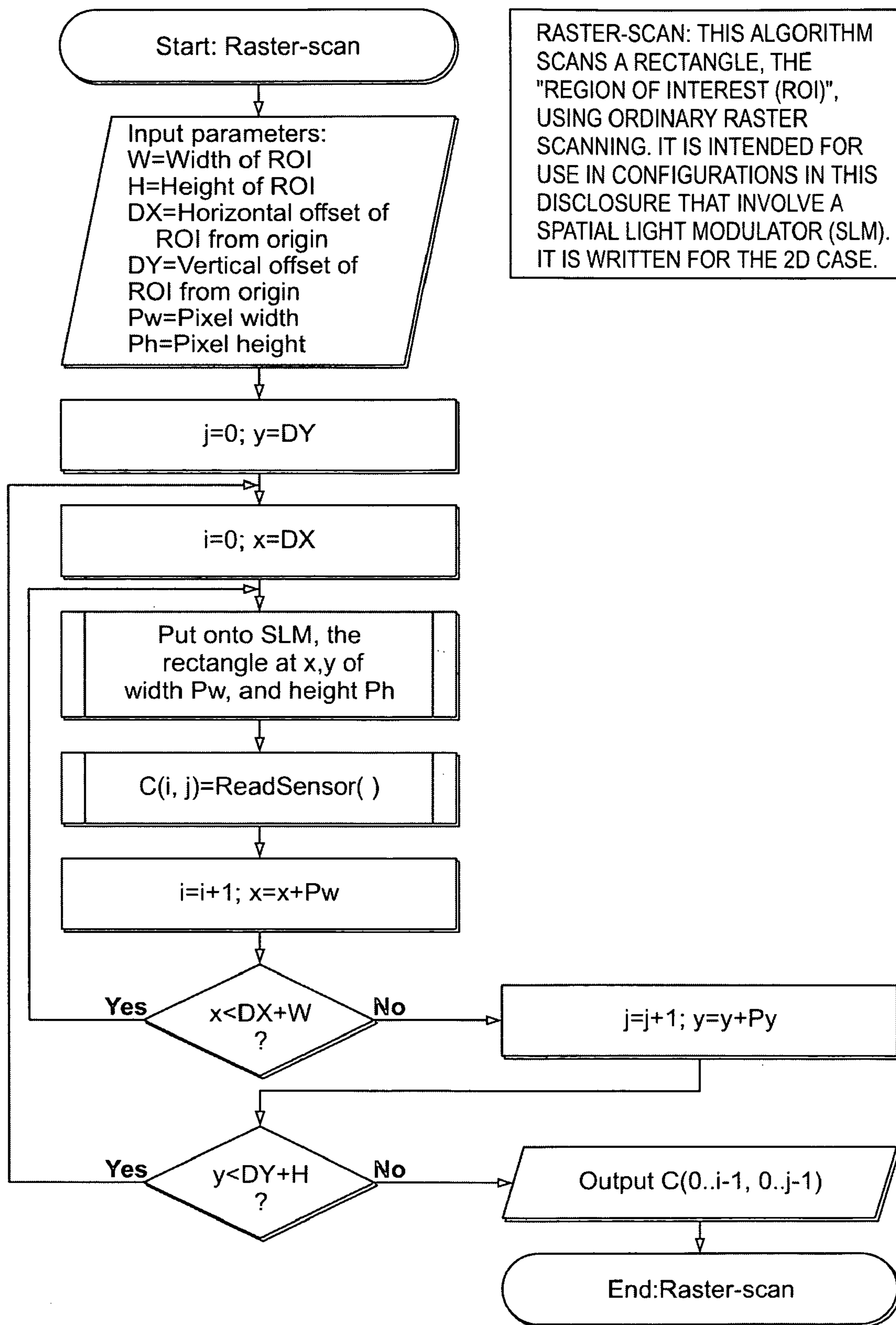
FIG. 24
