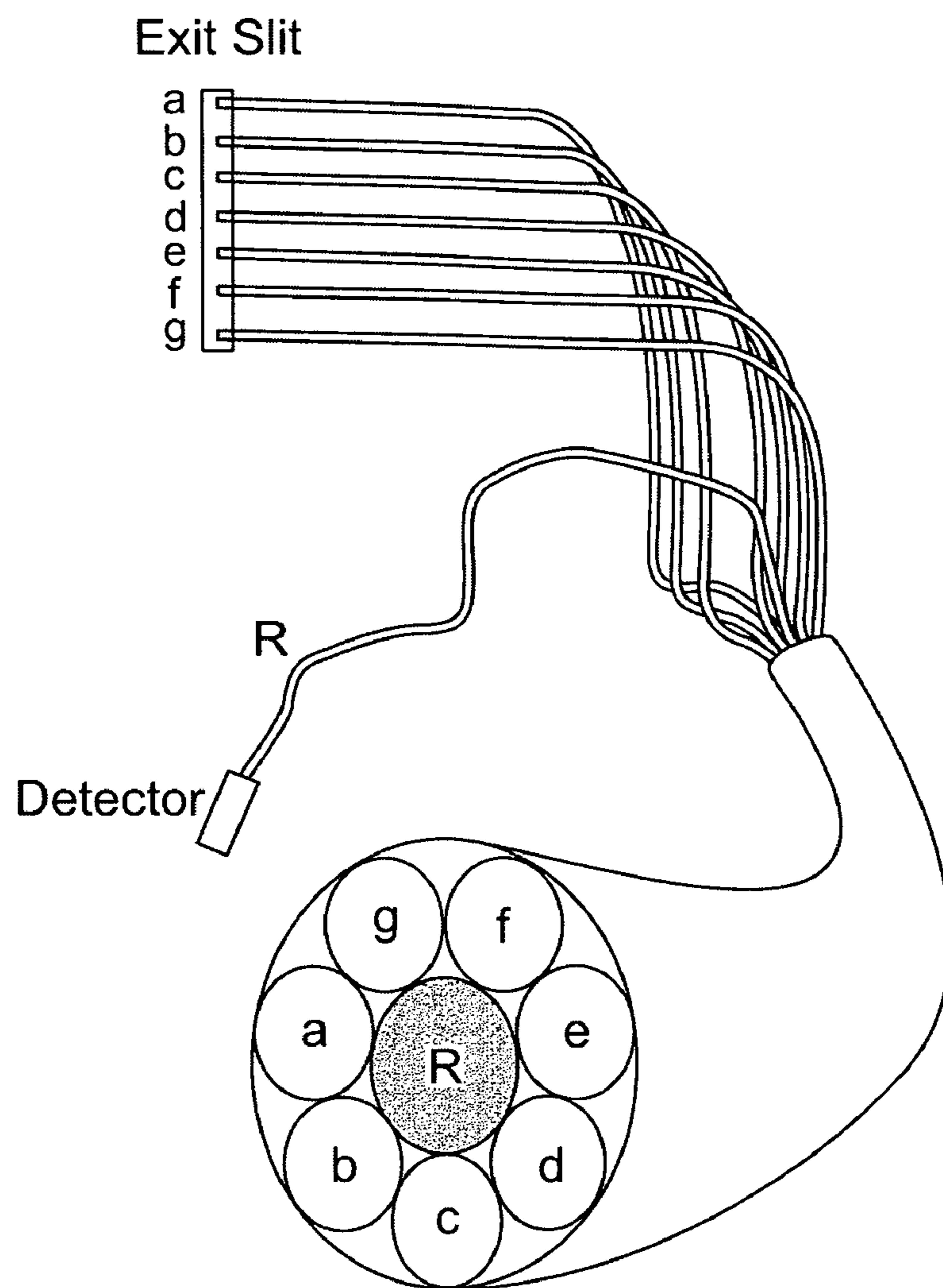
FIG. 35
