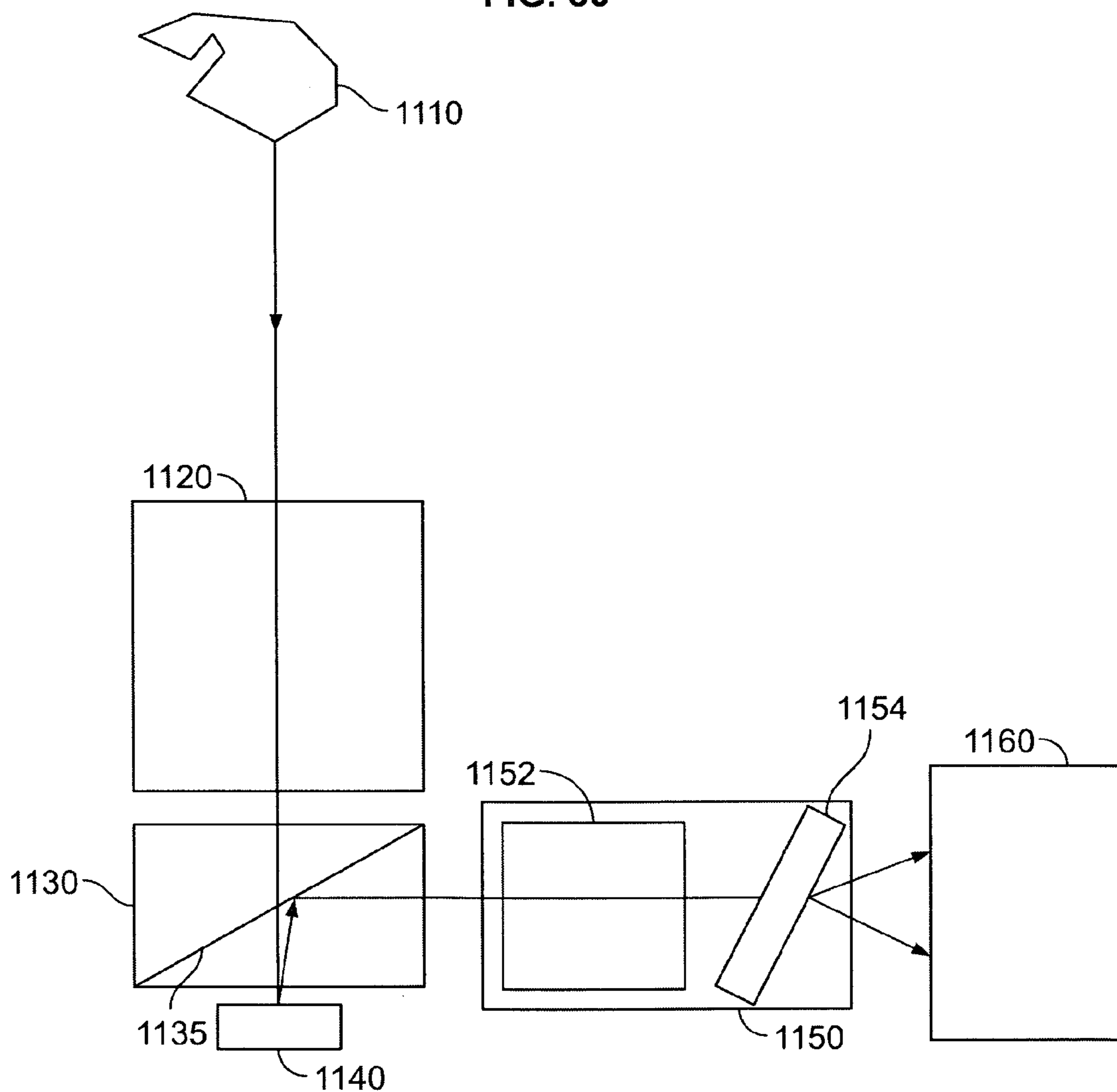
FIG. 50
