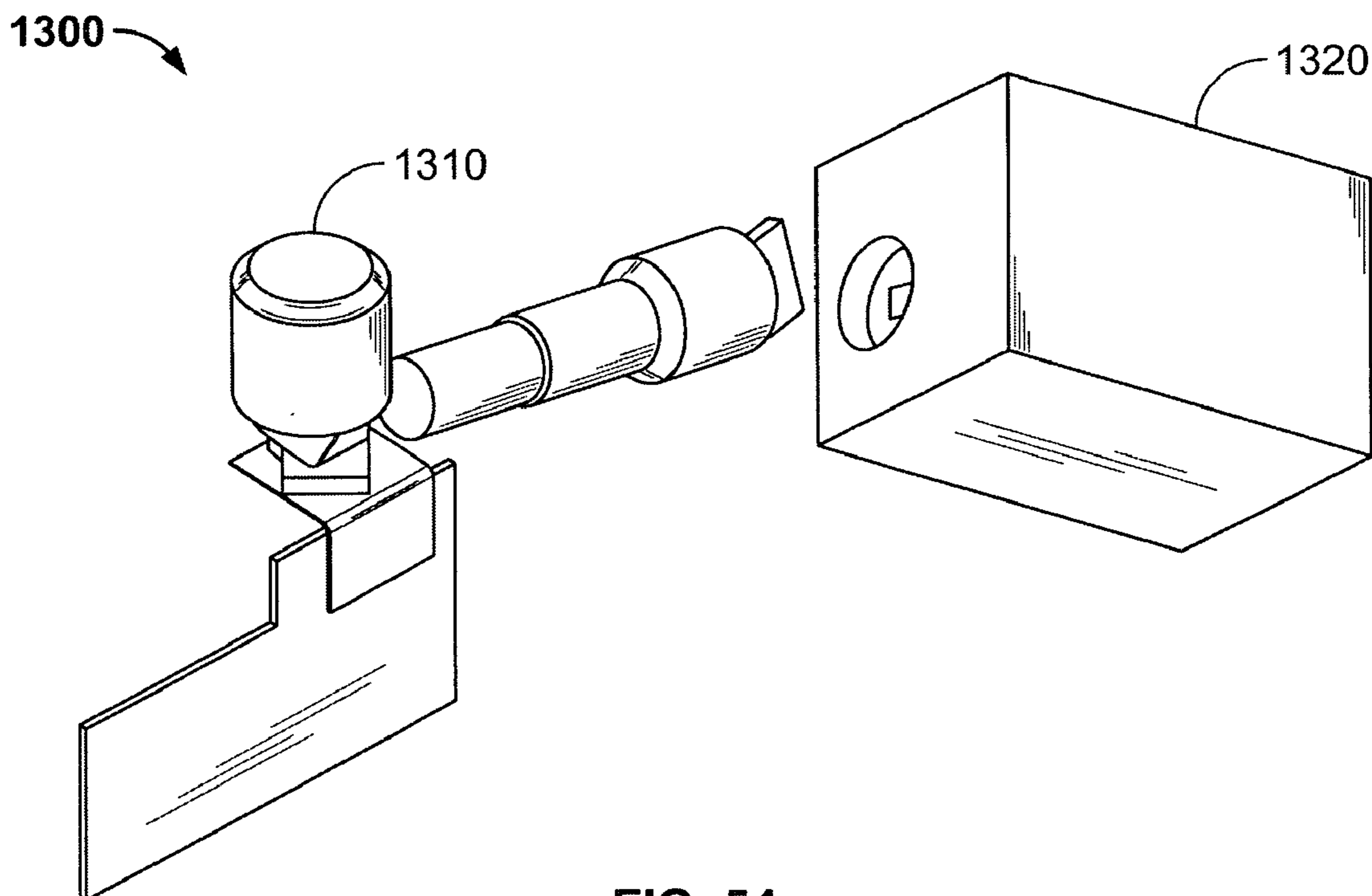
FIG. 54
