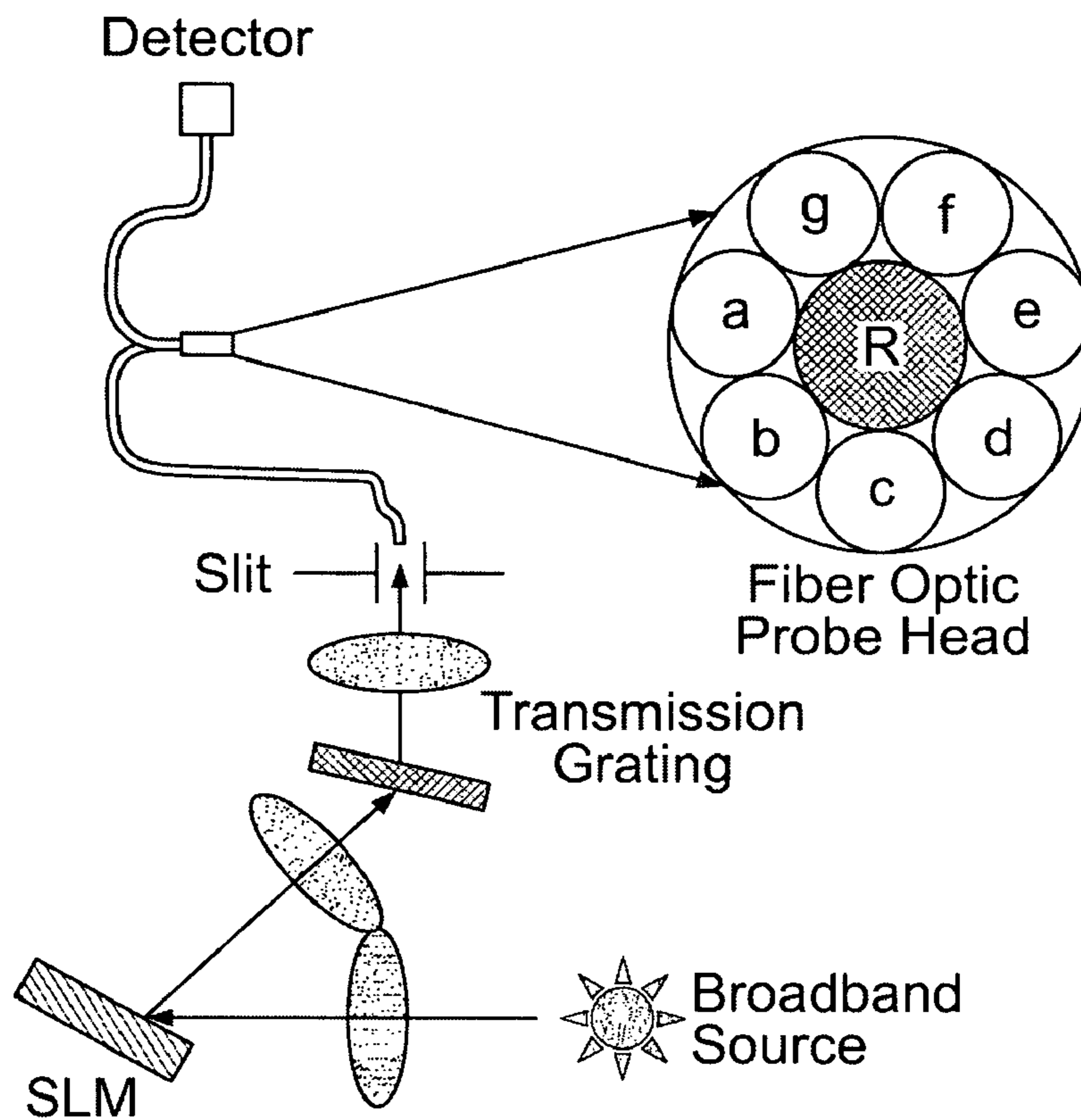
FIG. 33A
