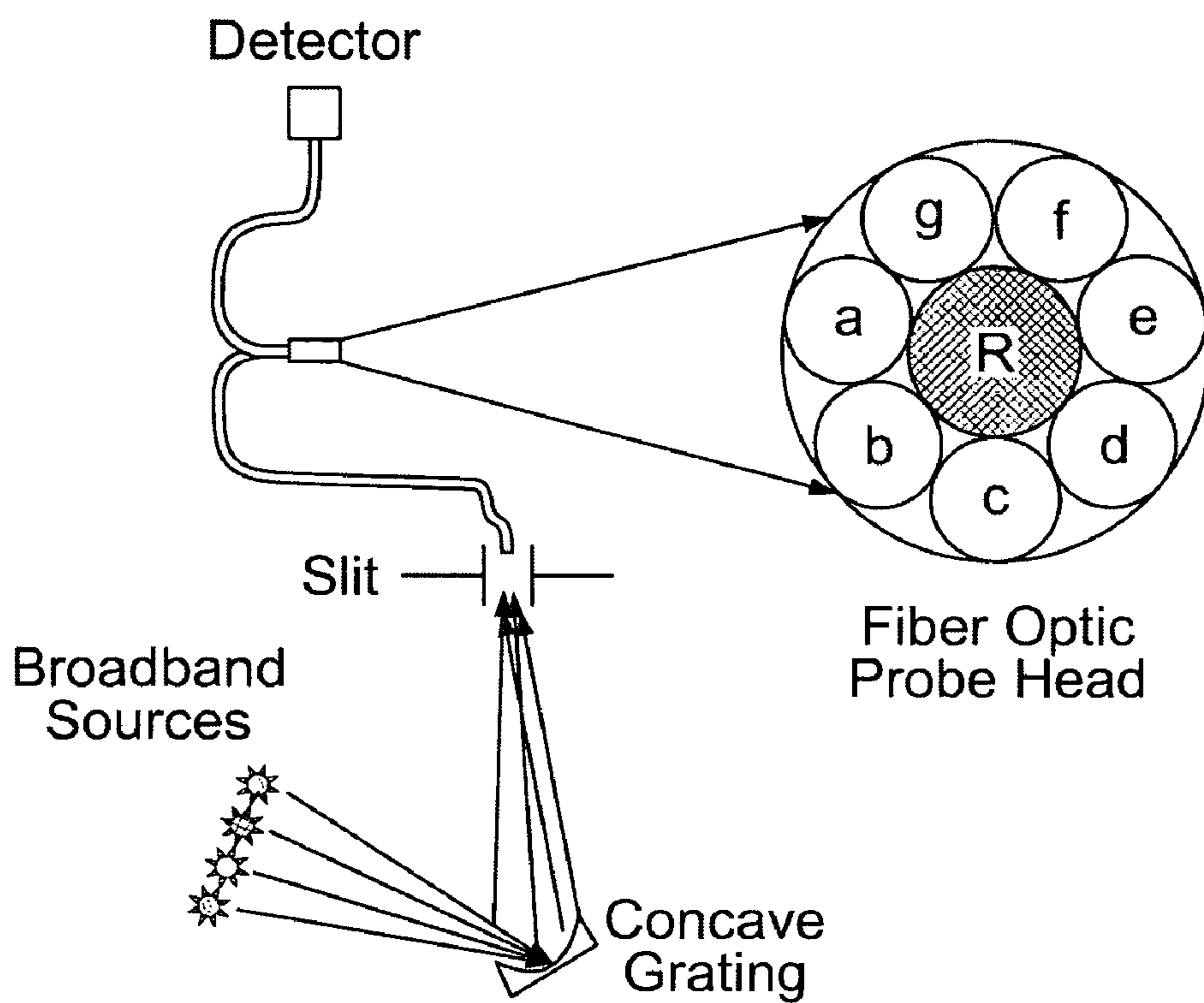
FIG. 33C
