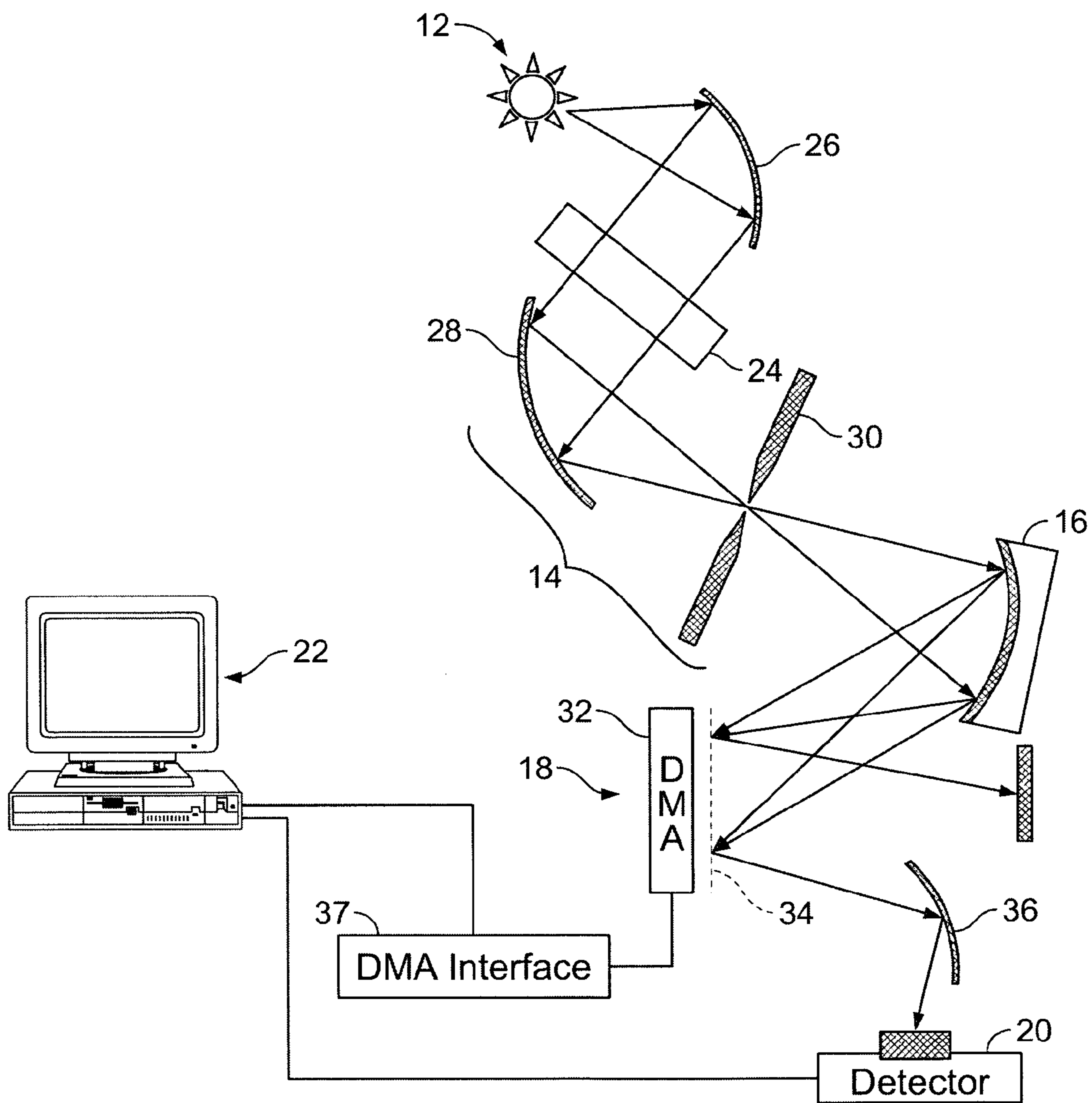
FIG. 1A
