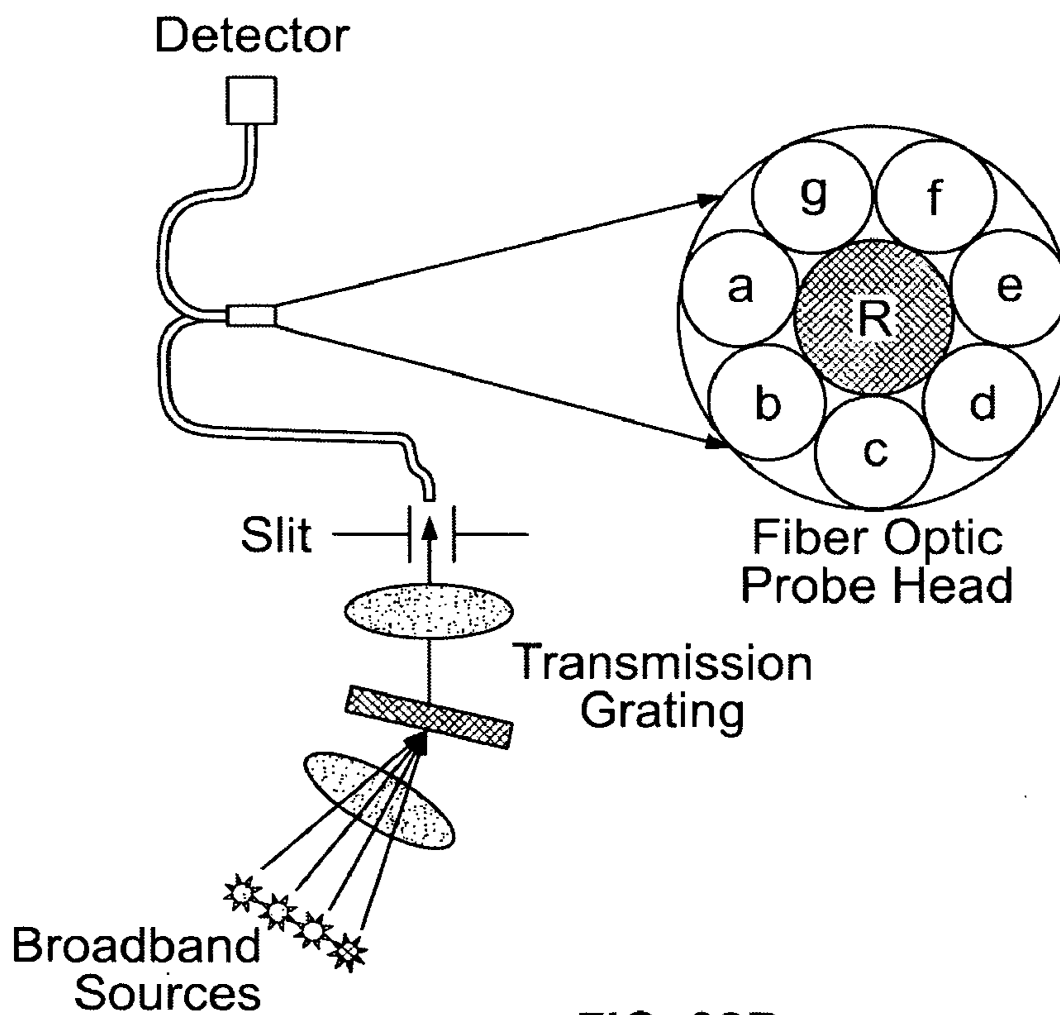
FIG. 33B
