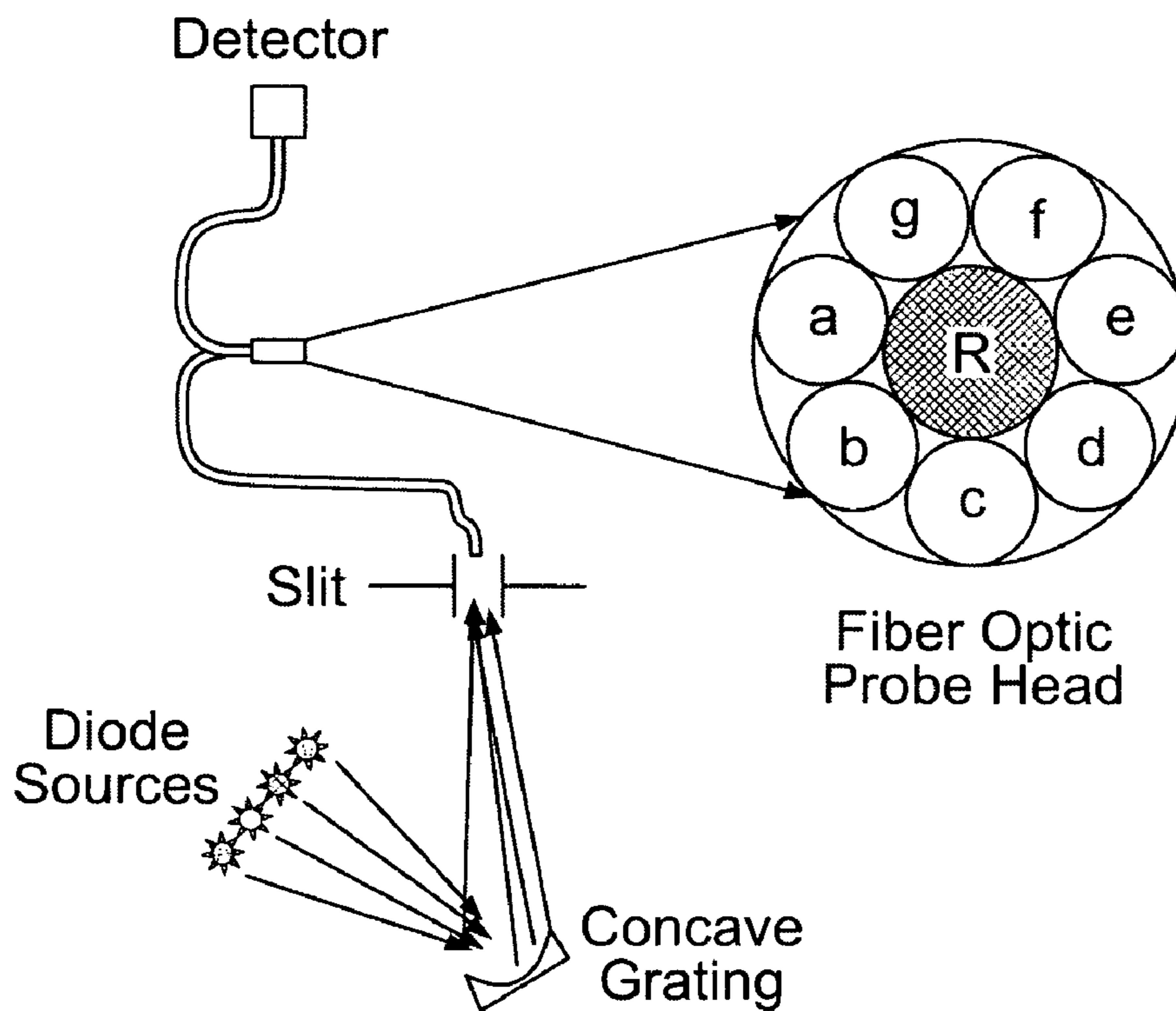
FIG. 33D
