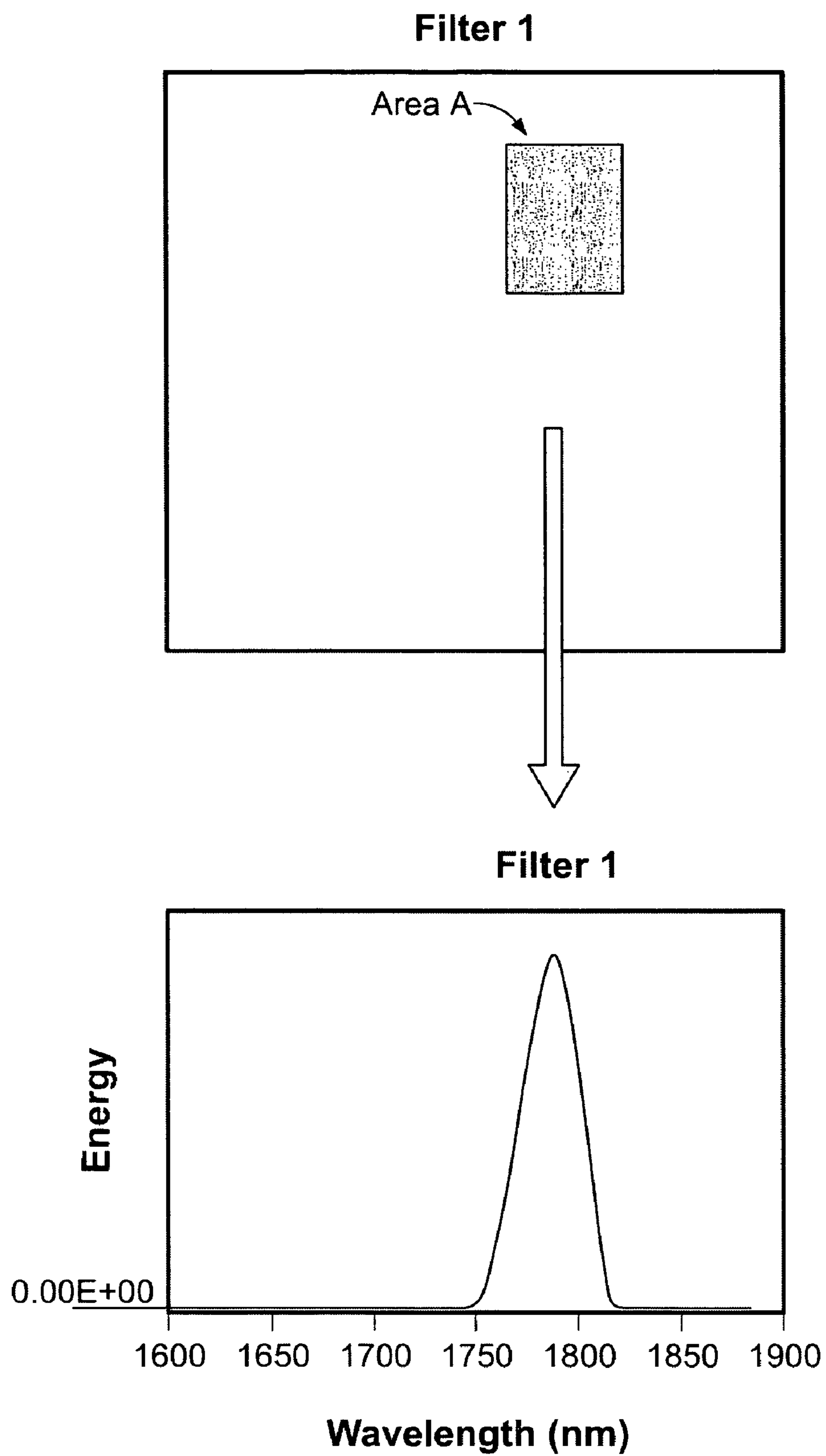
FIG. 9A
