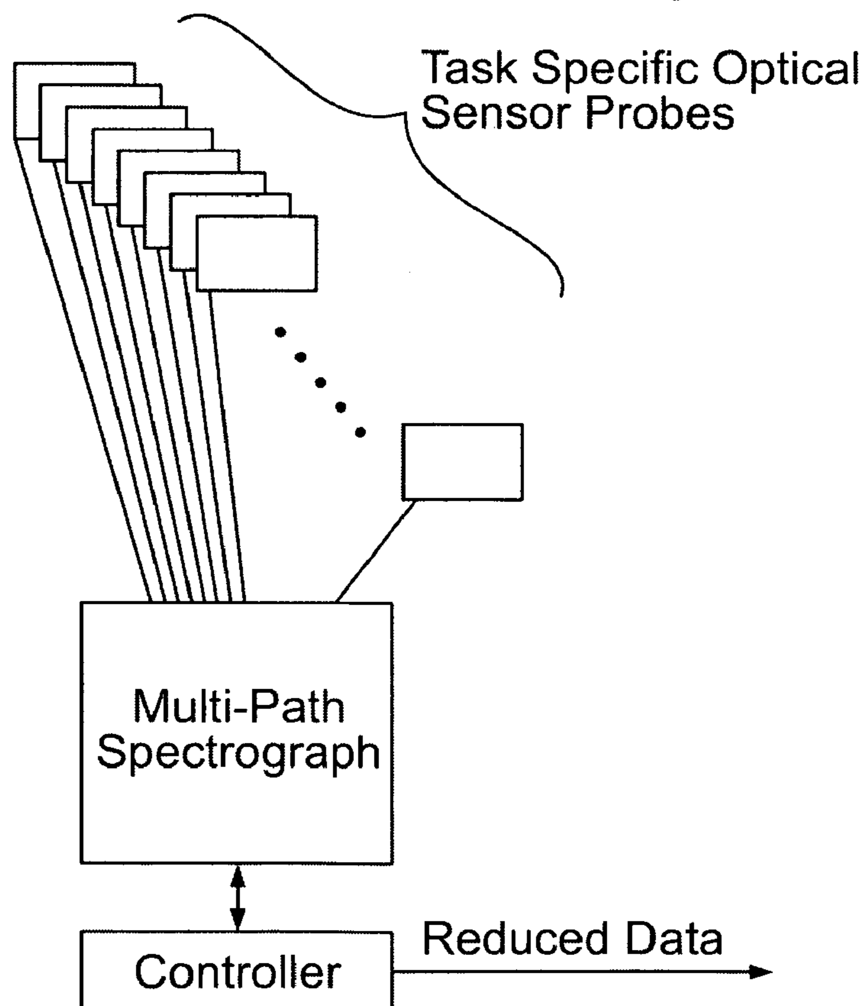
FIG. 29
